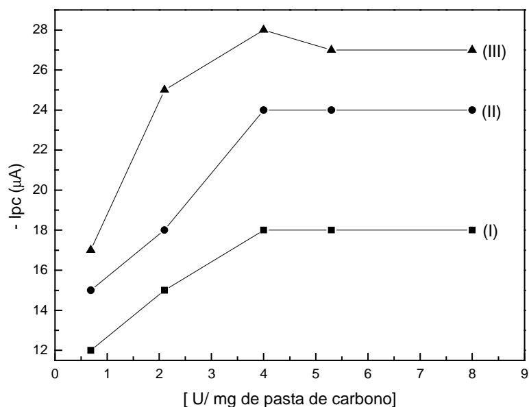
Figura 22. Efeito da concentração de peroxidase (0,69 a 8,0 U/ mg de pasta de carbono) em hidroquinona 3,0 \times 10^{-4} mol L -1 e peróxido de hidrogênio 2,0 \times 10^{-3} mol L -1 , 100 mV e 100 Hz.
