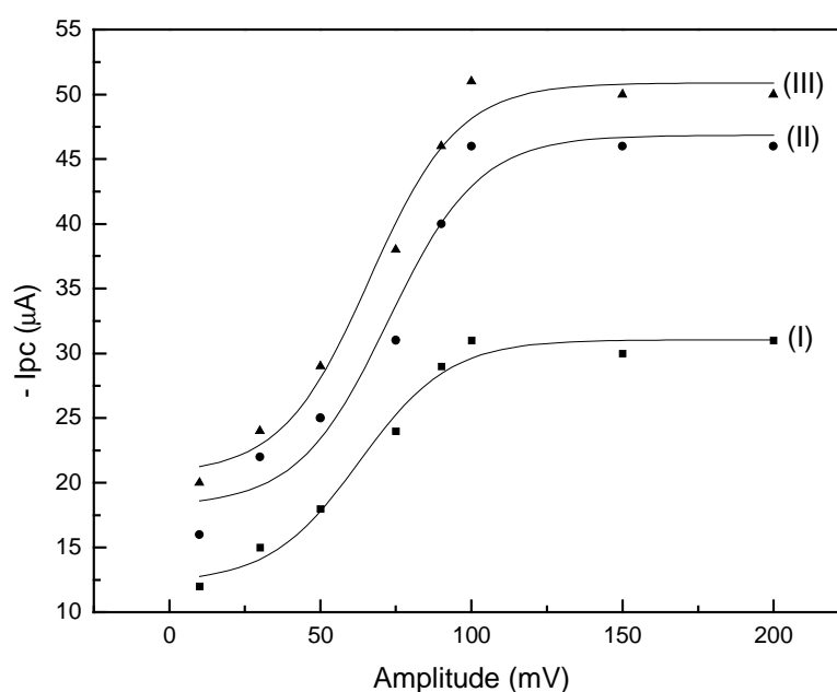
Figura 25. Estudo do efeito da amplitude do potencial (10 a 200 mV) em solução de hidroquinona 3,0 \times 10^{-4} \text{ mol L}^{-1} , peróxido de hidrogênio 2,0 \times 10^{-3} \text{ mol L}^{-1} e frequência de 100 Hz.
