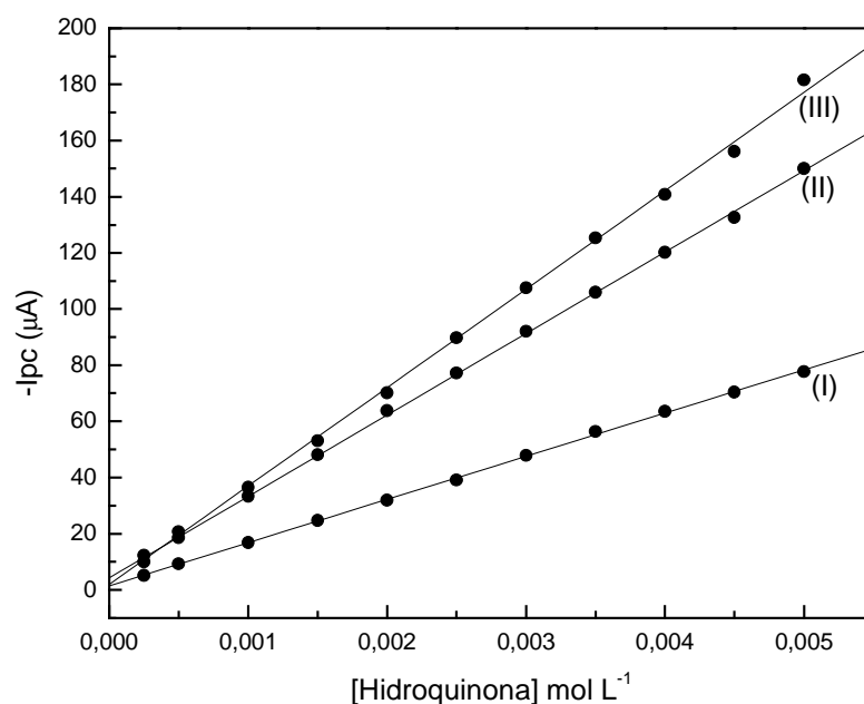
Figura 29. Curvas analíticas para hidroquinona obtidas com os biossensores propostos usando voltametria de onda quadrada.
