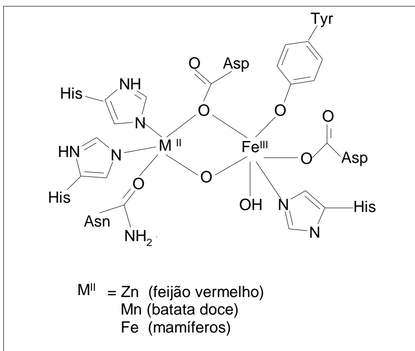
Figura 5. Representação esquemática da forma reduzida Fe^{III}M^{II} , do sítio ativo das fosfatases ácidas púrpuras extraídas de fontes animais e vegetais.
