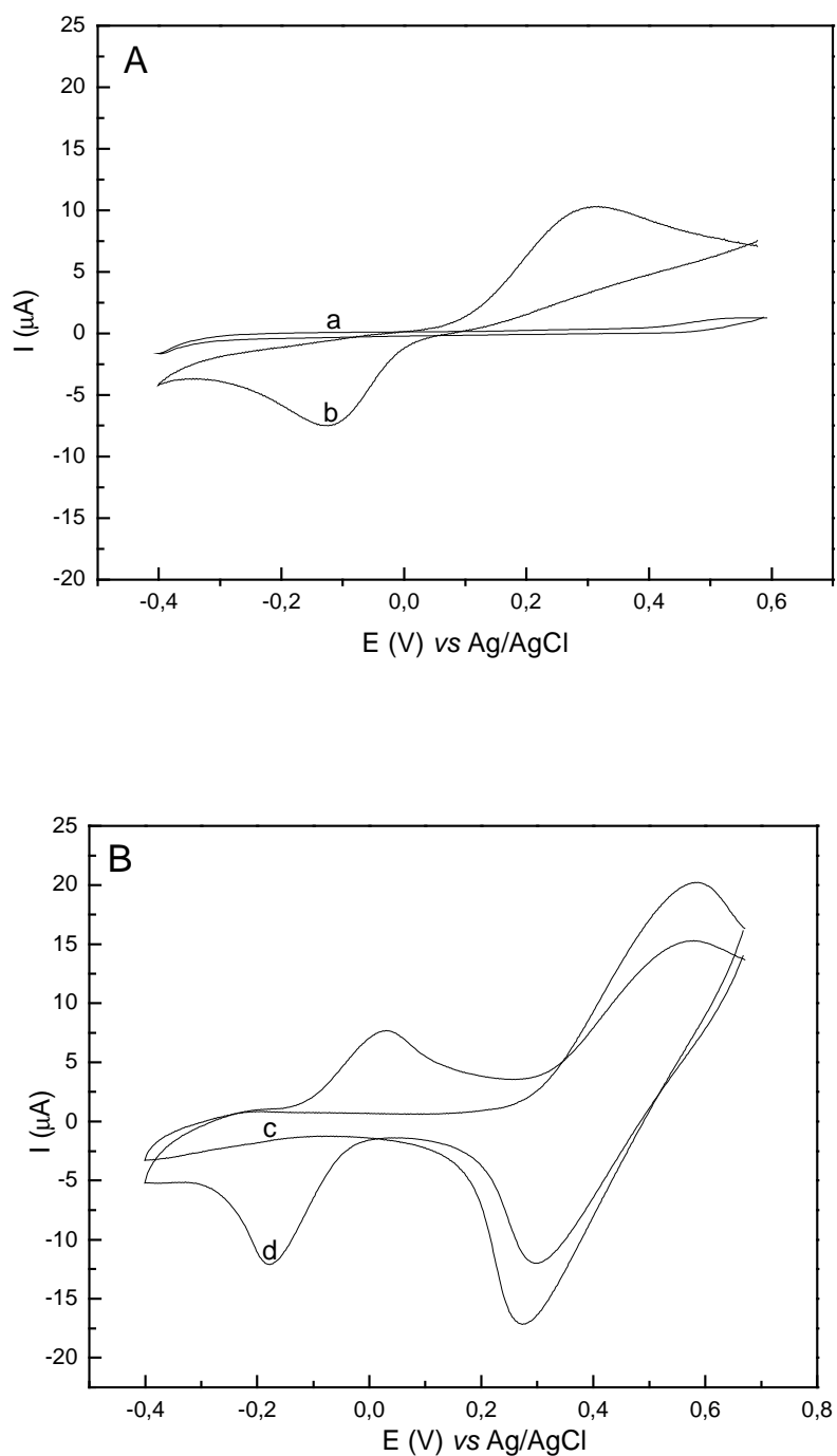
Figura 34. Voltamogramas cíclicos utilizando o (A) eletrodo de pasta de carbono e (B) sensor biomimético. Voltamogramas (a, c) obtidos em tampão fosfato 0,1 \text{ mol L}^{-1} (pH 7,0) e (b, d) hidroquinona 4,0 \times 10^{-4} \text{ mol L}^{-1} .
