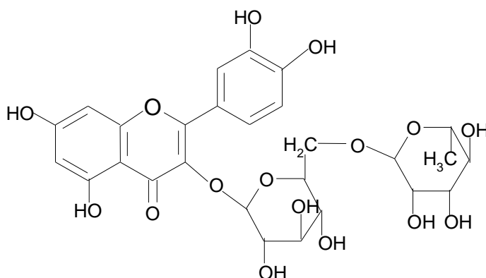
Figura 10. Estrutura química da rutina.
