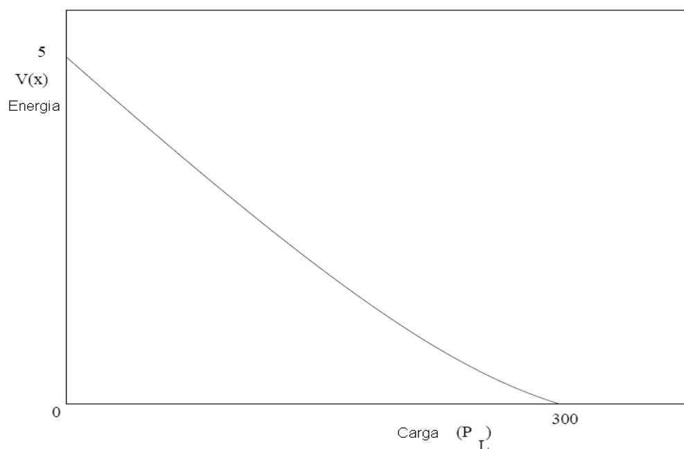
Figura 3.5 – Função energia versus potência ativa da carga
