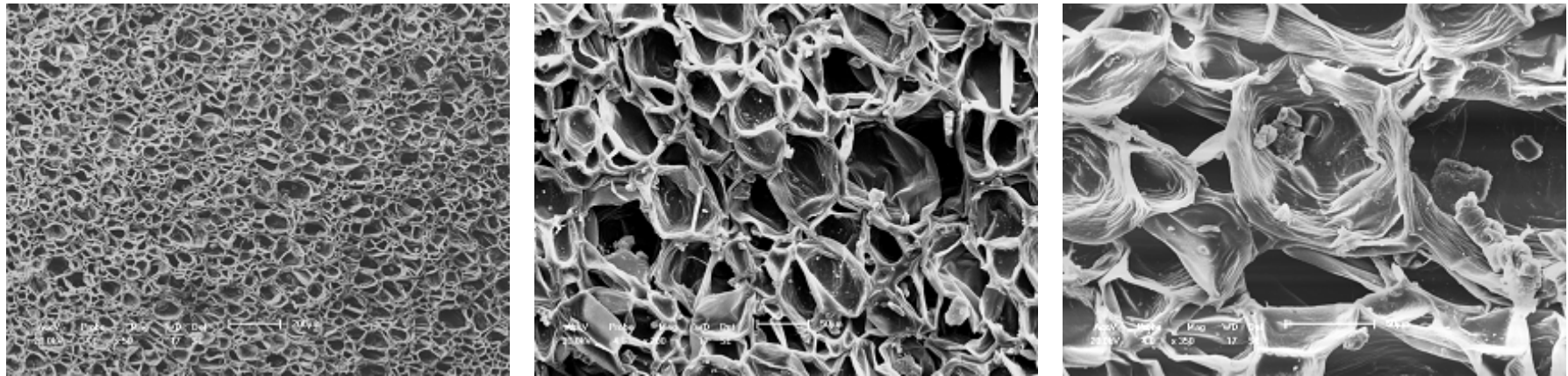
Figura 65 Espuma de EVA com 5 pcr de NCC, \phi de 8,3 \mu m, FDK 400 – Ampliação de 50X, 200X e 350X
