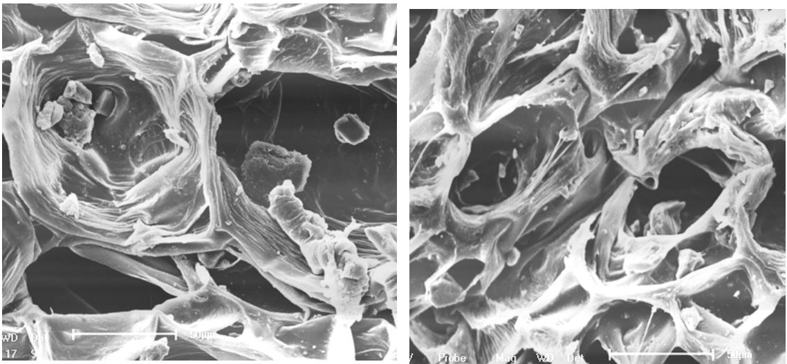
Figura 52. Espuma de EVA, ampliada 350X, com carbonato de cálcio natural EDK400, de \phi = 8,3 \mu\text{m} : (a) 5 pcr de carbonato; (b) 45 pcr de carbonato
