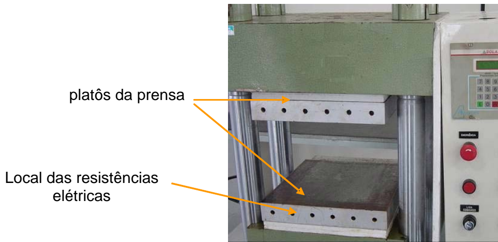
Figura 27. Prensa, com aquecimento elétrico, para reticulação e expansão
