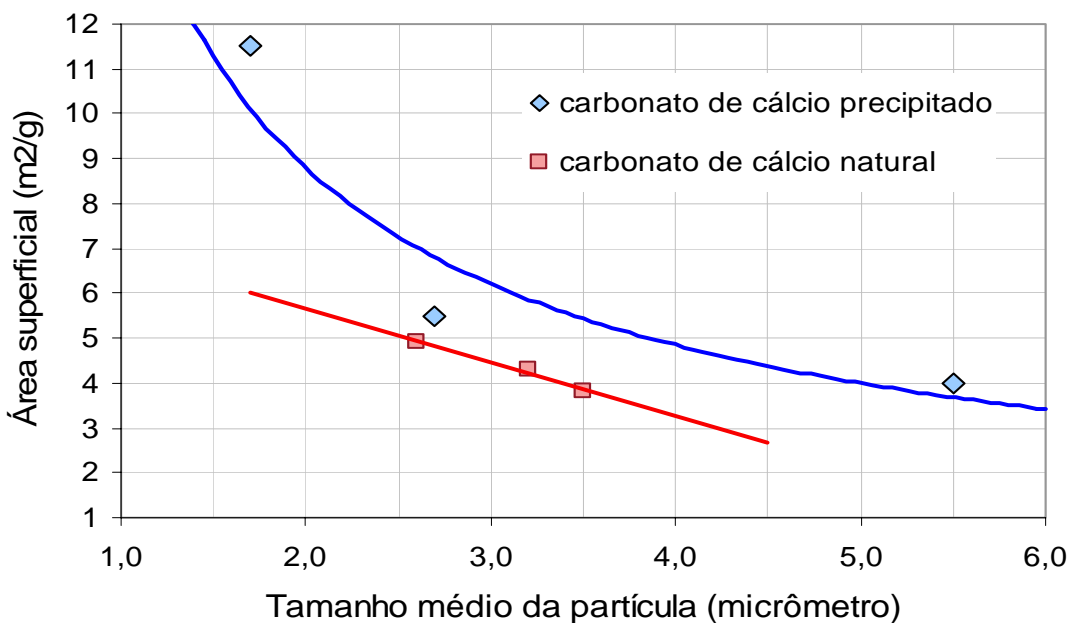
Figura 49. Área superficial dos carbonatos de cálcio naturais e precipitados (curvas construídas a partir dos dados da Tabela 20).
