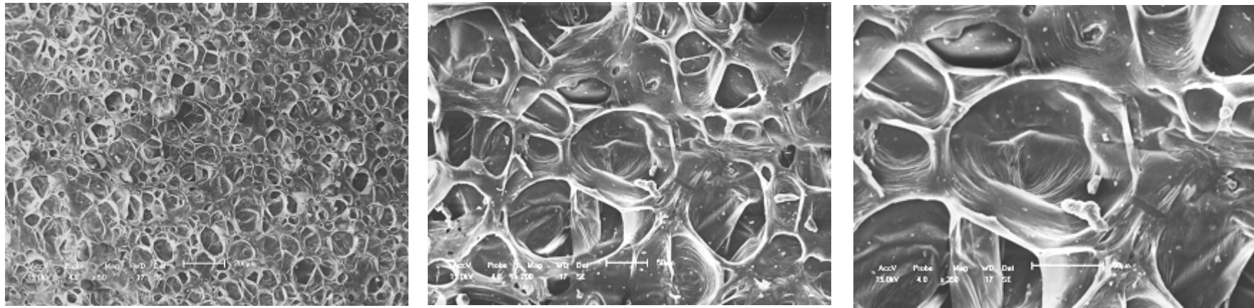
Figura 63. Espuma de EVA com 5 pcr de NCC, \phi de 5,3 \mu\text{m} , Supermicro K. Ampliação de 50X, 200X e 350X.
