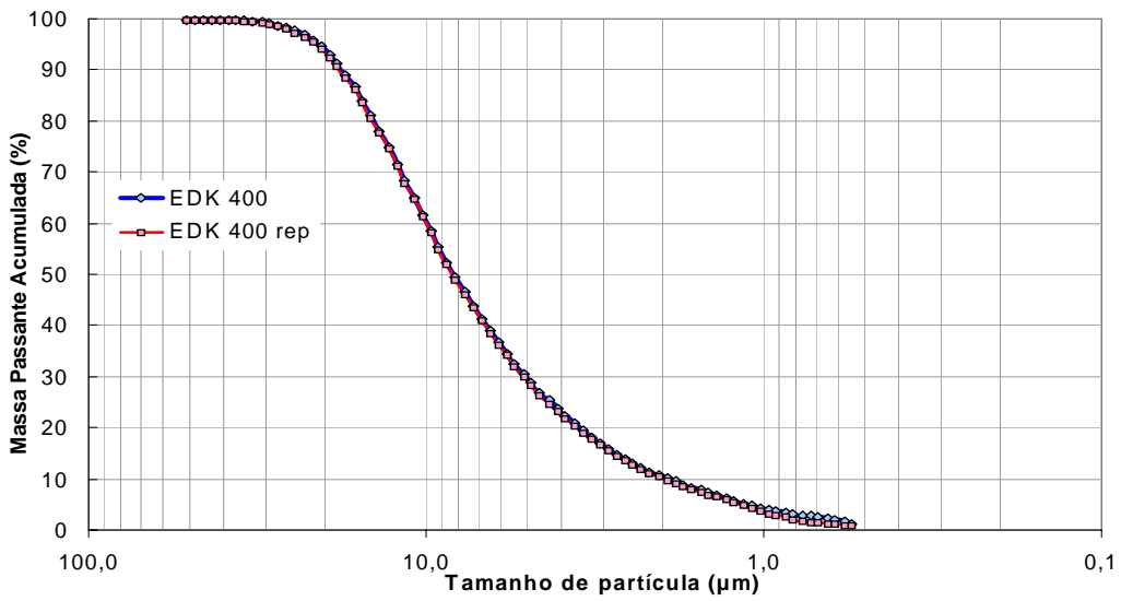
Figura 58. Curva da distribuição de tamanhos de partícula do carbonato de cálcio natural EDK 400.
