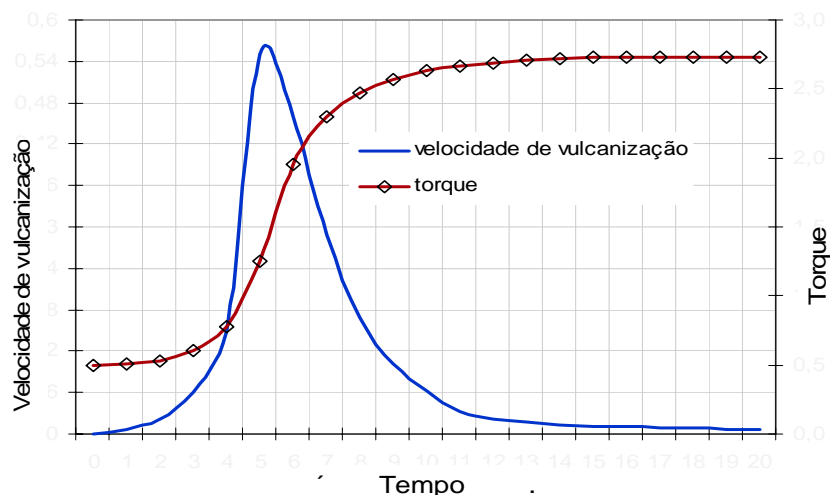
Figura 25. Curva ilustrativa do torque e velocidade de vulcanização em elastômeros. Reômetro de torque Monsanto
