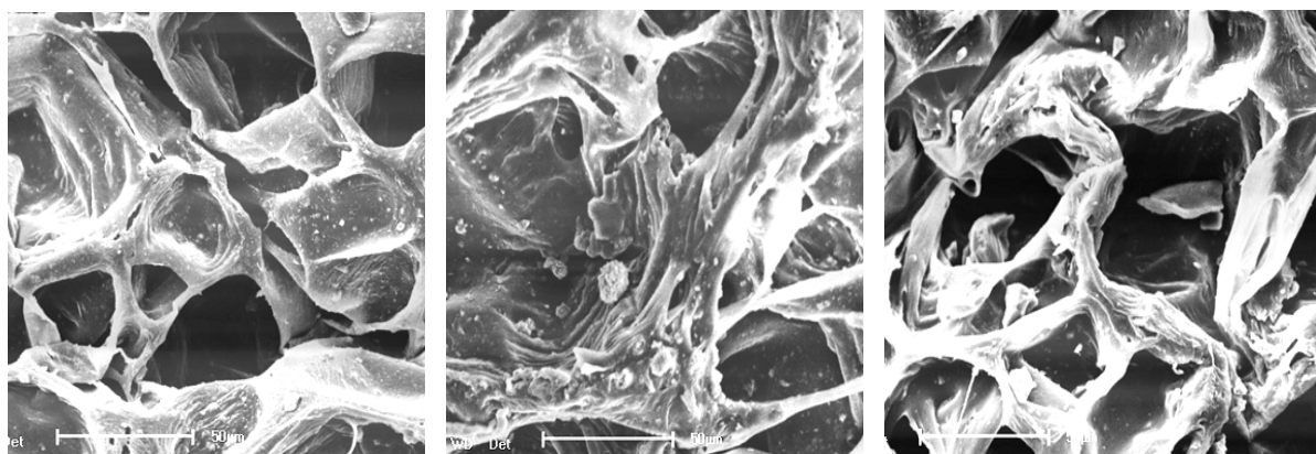
Figura 50. Espuma de EVA ampliada 350 X: (a) 45 pcr de PCC Barralin, \phi 1,7 \mu\text{m} ; (b) 45 pcr de PCC Barraleve, \phi 5,9 \mu\text{m} ; (c) 45 pcr de NCC EDK 400, \phi 8,3 \mu\text{m}
