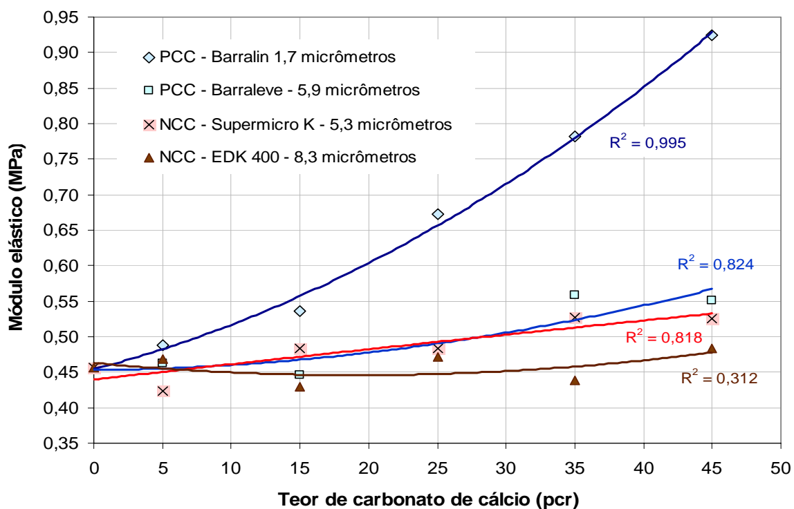
Figura 44. Módulo elástico da espuma de EVA, em função do tipo e teor de carbonato de cálcio
