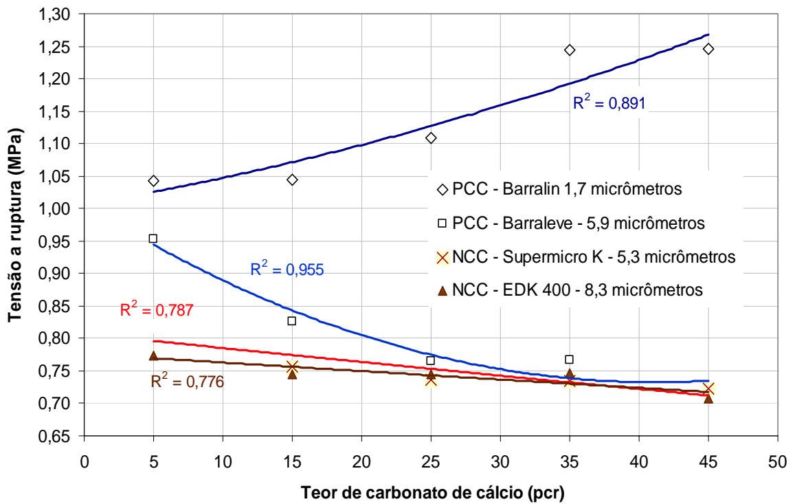
Figura 46. Resistência à tração da espuma de EVA, em função do tipo e teor de carbonato de cálcio
