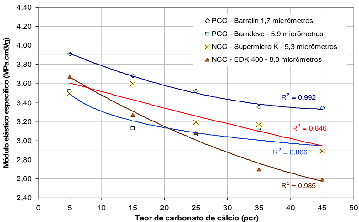
Figura 45. Módulo elástico específico da espuma de EVA, em função do tipo e teor de carbonato de cálcio
