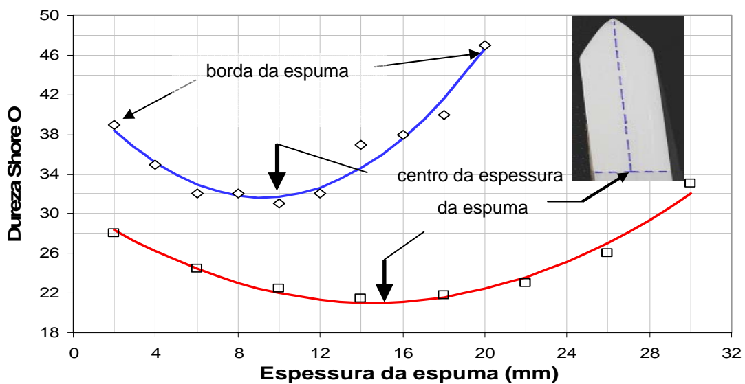
Figura 41. Dureza ao longo da espessura da espuma: (a) espuma com 35 pcr de PCC Barralin; (b) espuma com 35 pcr de PCC Barraleve
