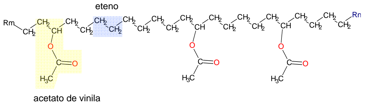
Figura 5. Modelo da estrutura do EVA [KAKUGO, 1984].
