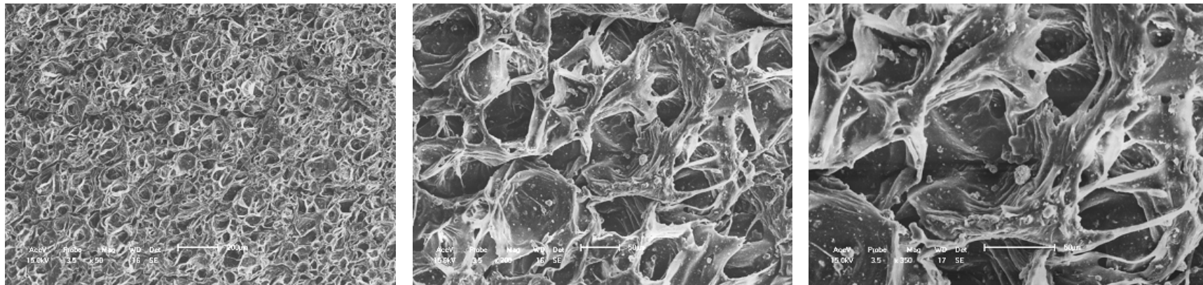
Figura 62. Espuma de EVA com 45 pcr de PCC, \phi de 5,9 \mu\text{m} , Barraleve. Ampliação de 50X, 200X e 350X.
