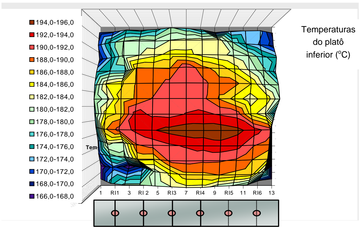
Figura 29. Temperaturas do platô inferior da prensa
