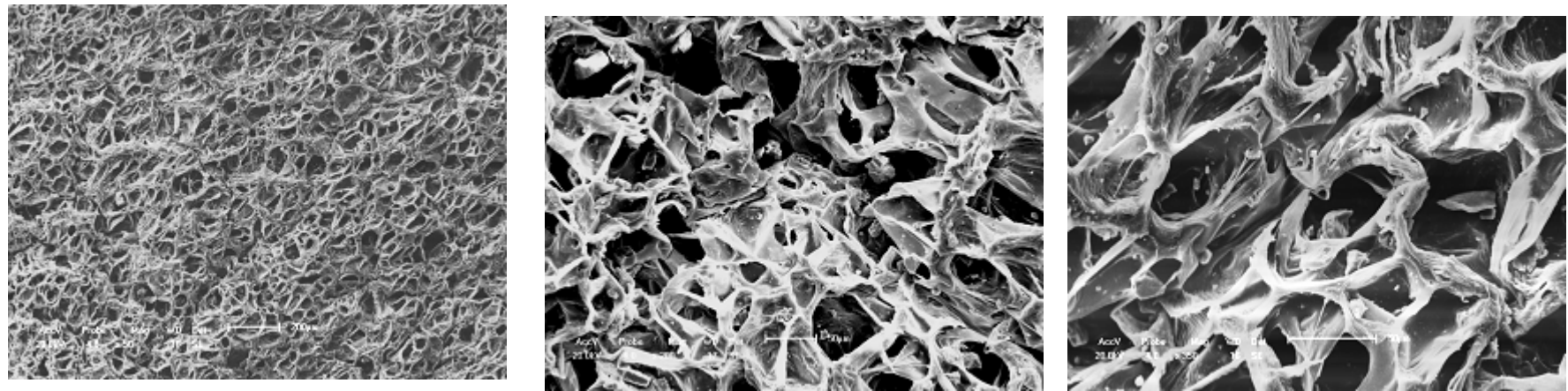
Figura 66. Espuma de EVA com 45 pcr de NCC, \phi de 8,3 \mu m, EDK 400 – Ampliação de 50X, 200X e 350X.
