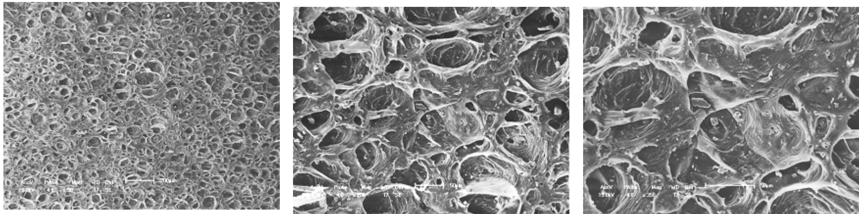
Figura 64. Espuma de EVA com 45 pcr de NCC, \phi de 5,3 \mu\text{m} , Supermicro K. Ampliação de 50X, 200X e 350X.
