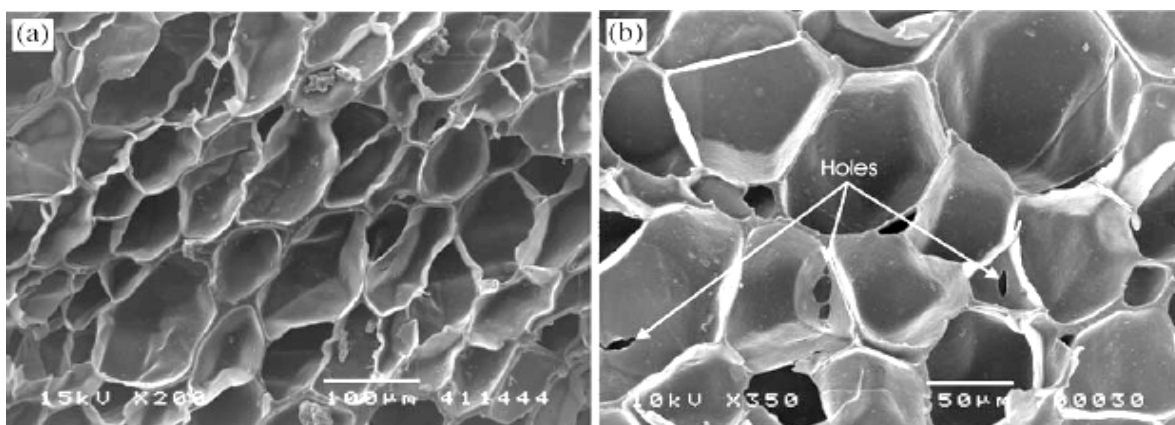
Figura 4. Salto de sapatos tênis, de espuma de EVA, com células deformadas ou com furos, após (a) 500km e (b) 750 km [VERDEJO e MILLS, 2004].
