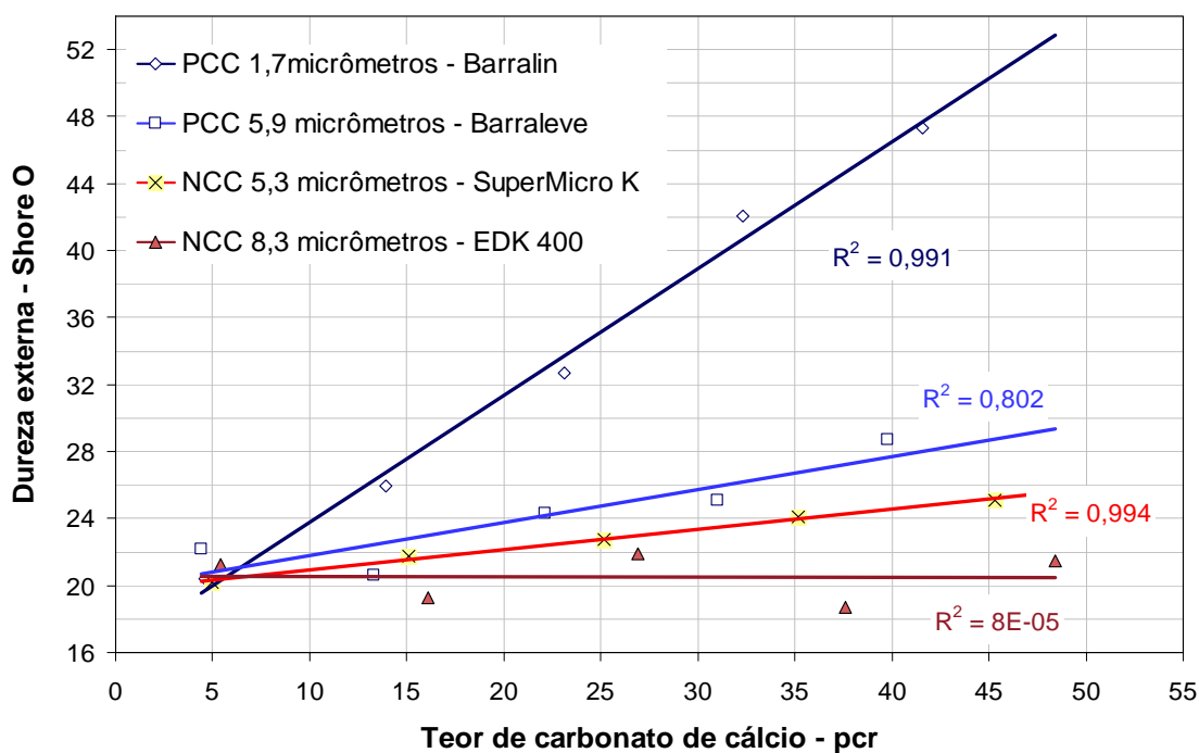
Figura 38. Dureza externa da espuma de EVA em função da granulometria e teor de carbonato de cálcio na formulação
