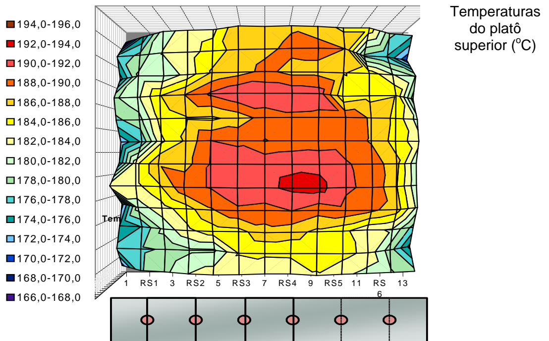
(b) Temperaturas do platô superior, vista de cima.
