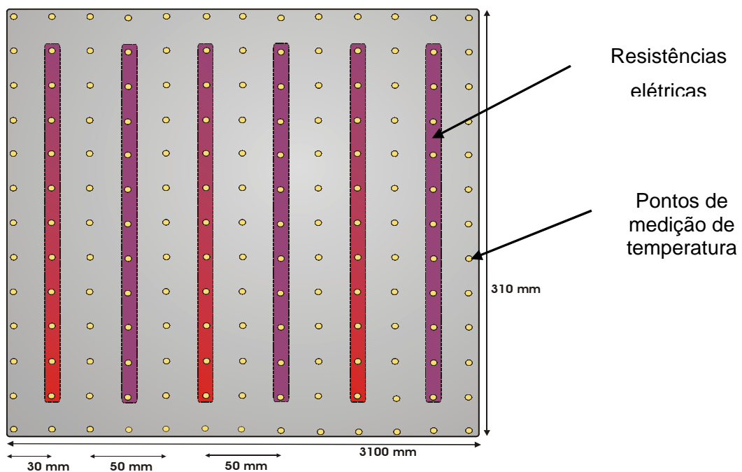
Figura 28. Resistências elétricas no platô da prensa e pontos de medição de temperatura
