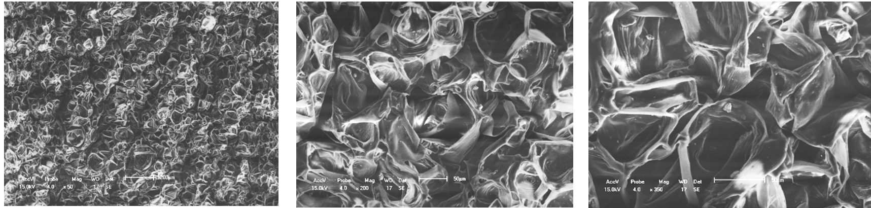
Figura 59. Espuma de EVA com 5 pcr de PCC, \phi de 1,7 \mu m, Barralin. Ampliação de 50 X, 200 X e 350 X.
