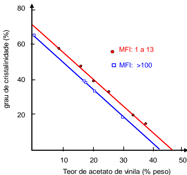
Figura 7. Grau de cristalinidade do EVA em função do teor de acetato de vinila.
