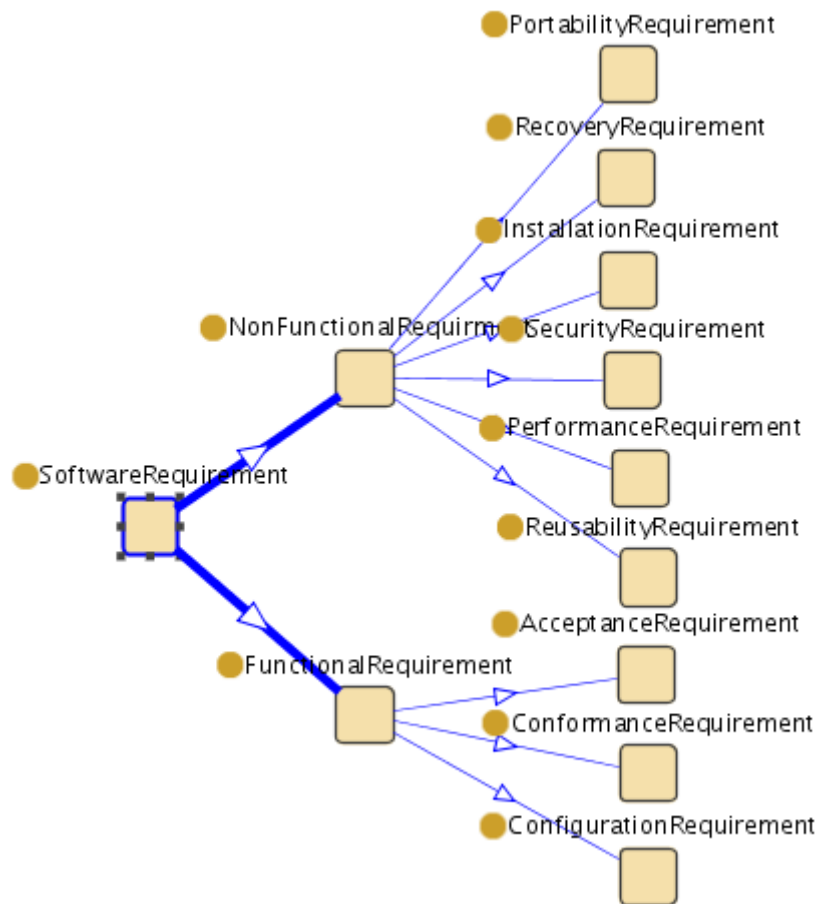
Figura A.17: A classe SoftwareRequirement e suas subclasses
