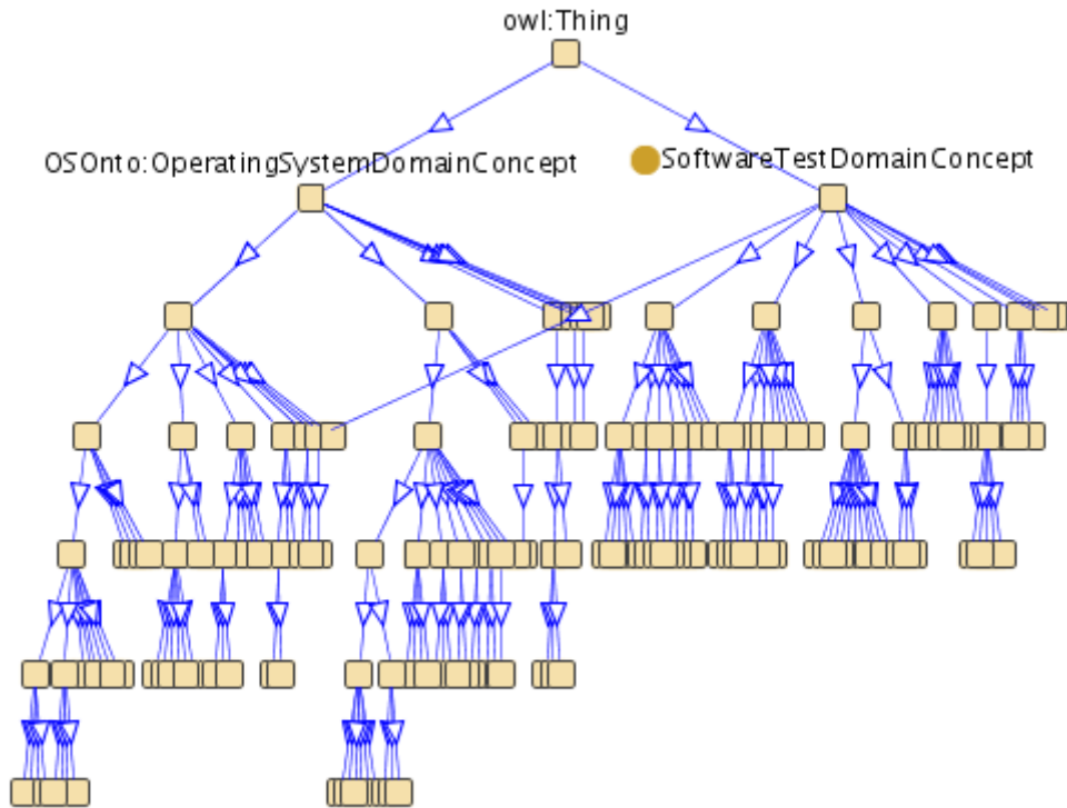
Figura 7.1: Árvore formada por classes e relações é-um da SwTO I
