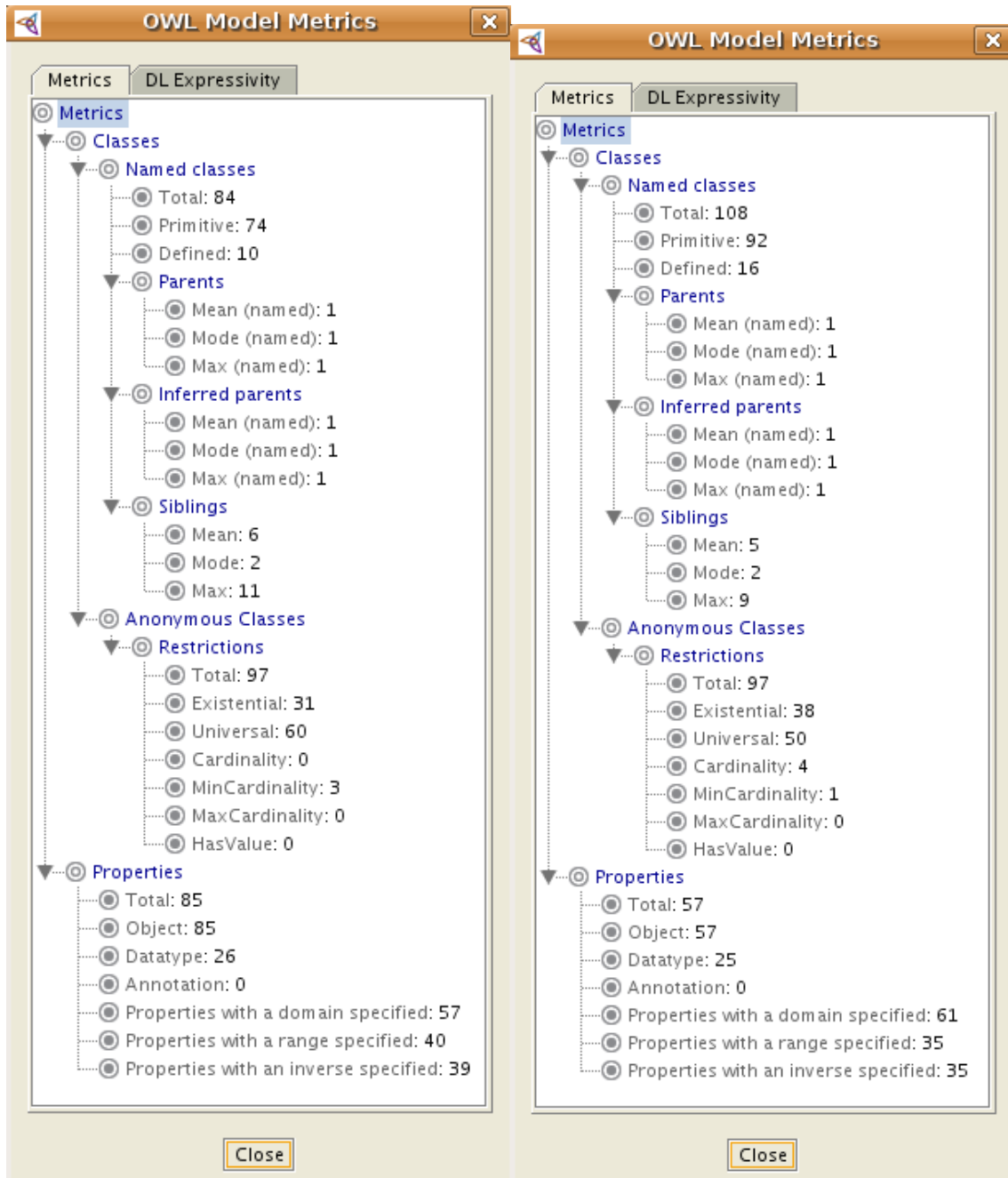
Figura 7.4: Métricas da SwTO
