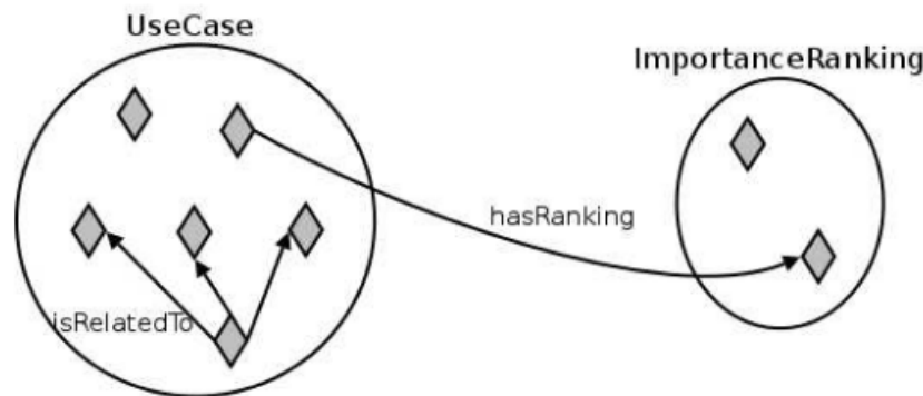
Figura 6.5: Relacionamento entre indivíduos da classe UseCase e ImportanceRanking [7].
