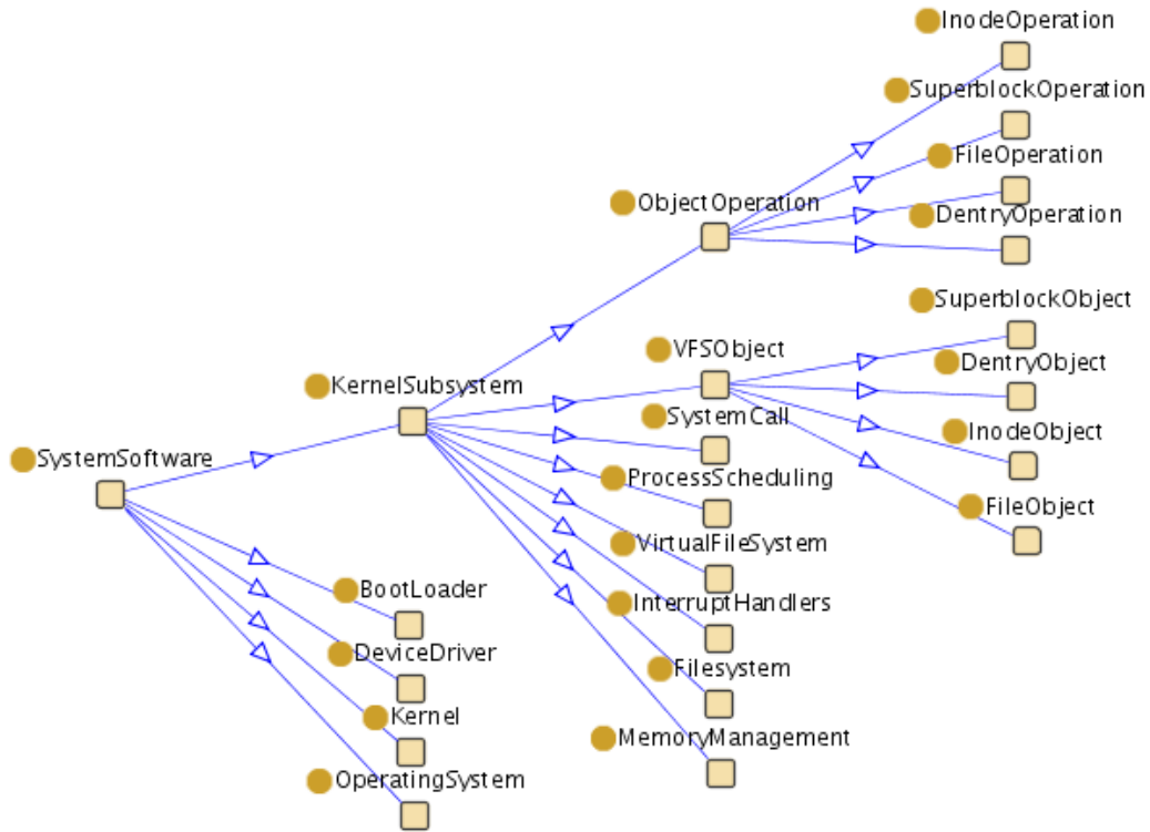
Figura A.9: A classe System Software e suas subclasses
