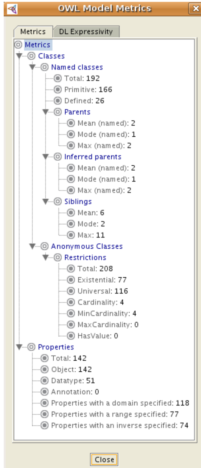
Figura 7.3: Métricas da SwTO I
