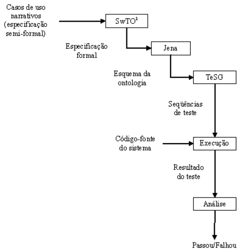
Figura 6.1: Visão geral do fluxo da TeSG
