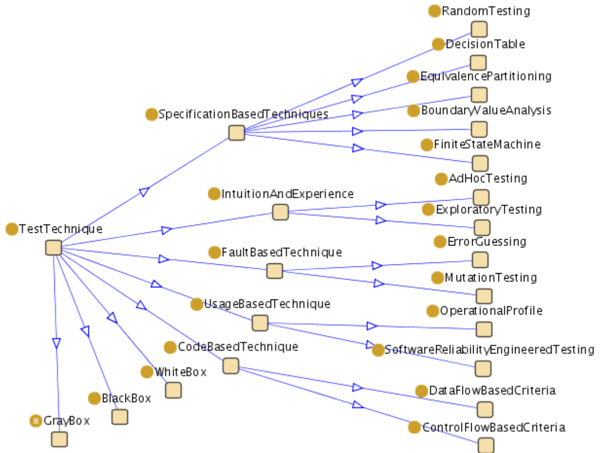
Figura 5.13: TestTechnique e suas subclasses
