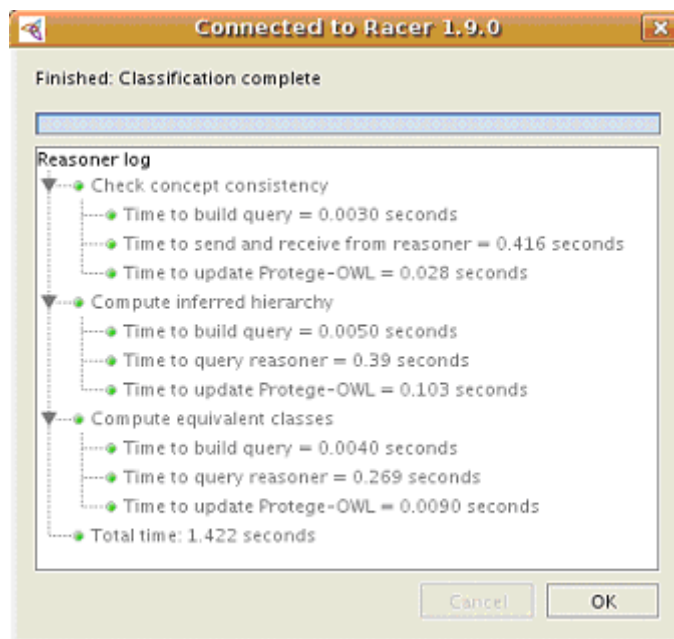
Figura 7.8: Resultados após a classificação de taxonomia da SwTO I
