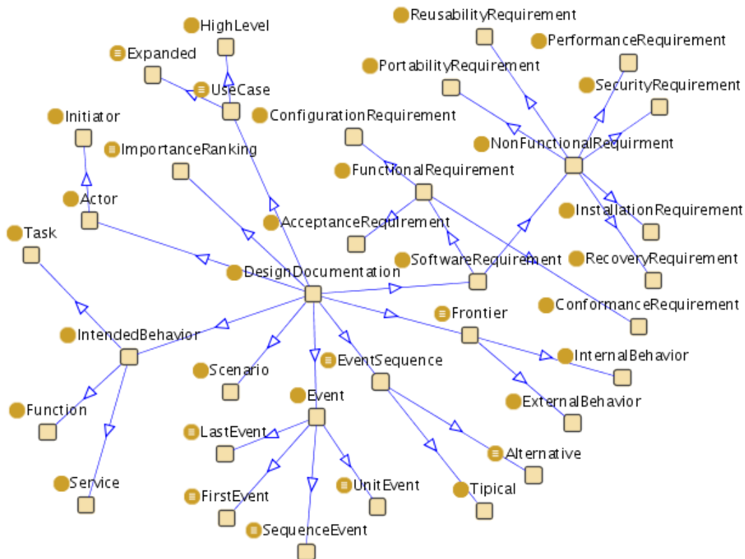
Figura A.12: A classe DesignDocumentation e suas subclasses
