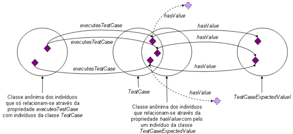
Figura 5.7: Esquema da condição necessária e suficiente da classe TestExecution
