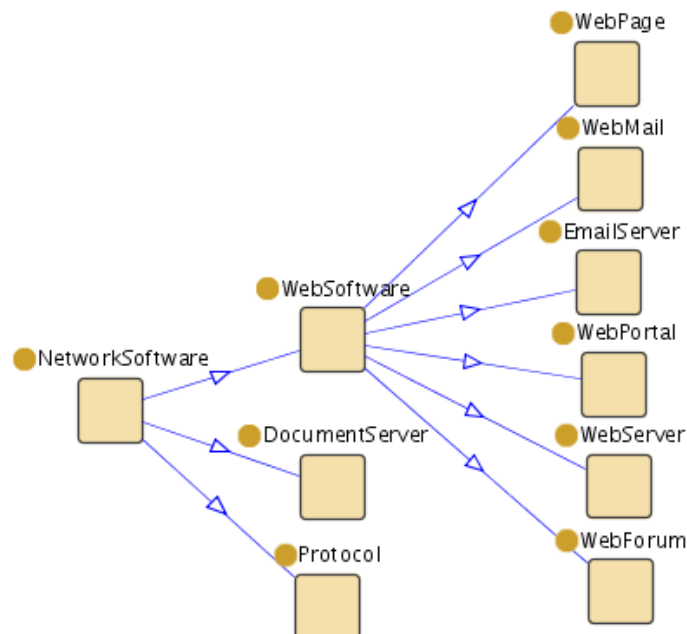
Figura A.8: A classe NetworkSoftware e suas subclasses
