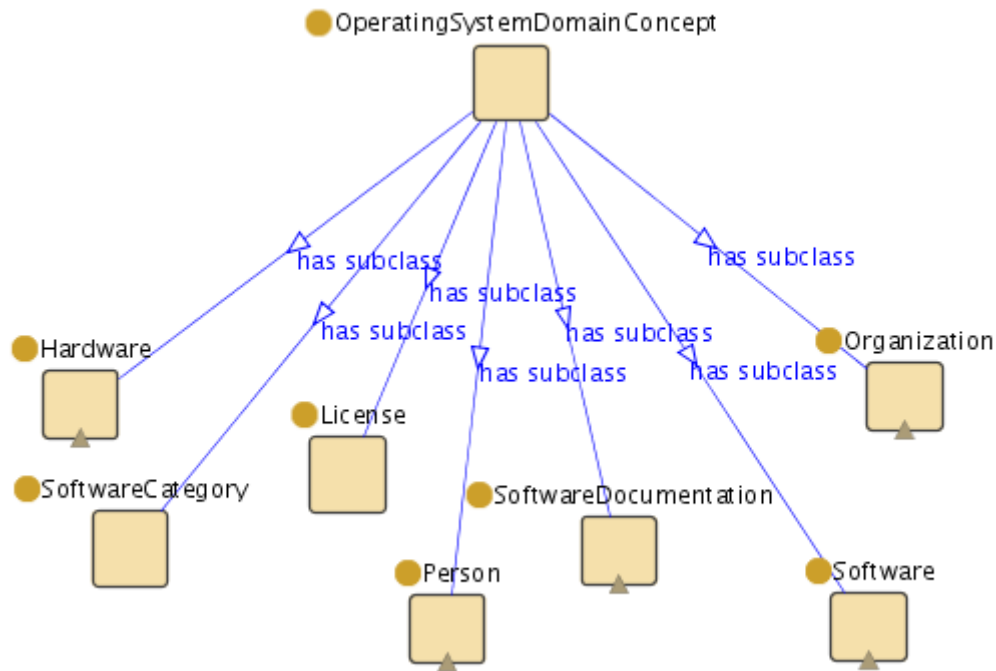
Figura A.1: A classe OperatingSystemDomainConcept e suas subclasses
