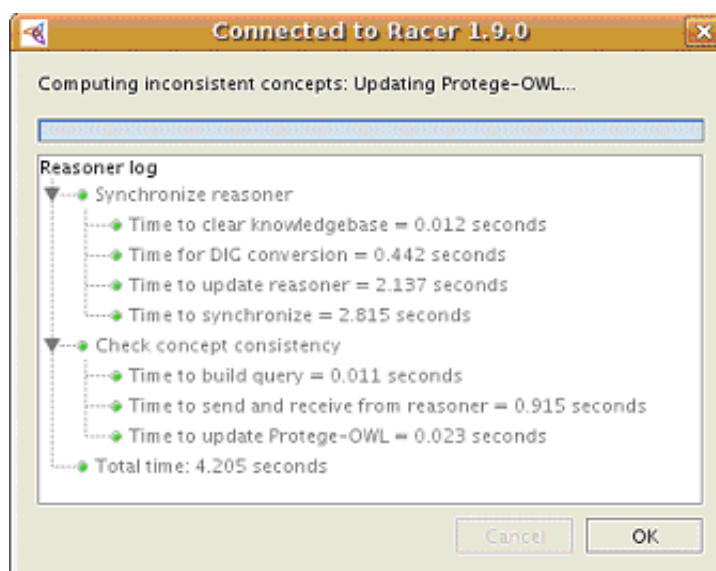
Figura 7.7: Resultados após a verificação de consistência da SwTO I
