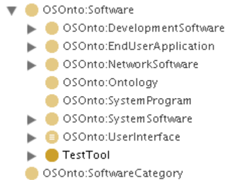
Figura 7.11: A classe TestTool na taxonomia inferida
