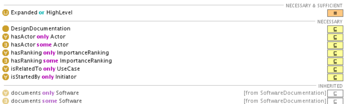
Figura 6.3: Descrição lógica da classe UseCase
