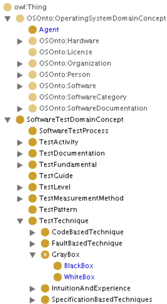
Figura 7.9: A hierarquia inferida da SwTO I destacada pelo Protégé
