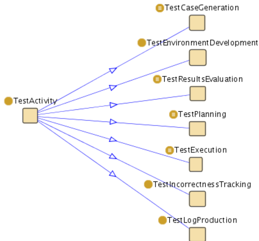
Figura 5.6: TestActivity e suas subclasses
