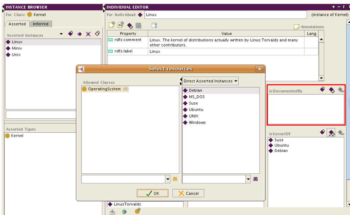
Figura 4.2: Associação entre instâncias através da propriedade isKernelOf
