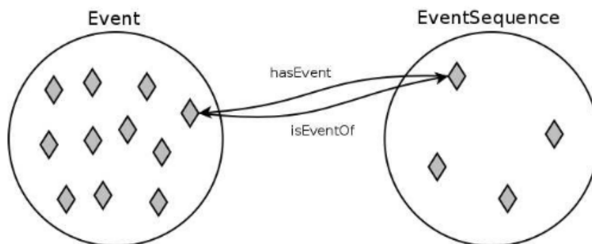
Figura 6.12: Relacionamento entre instâncias da classe Event e EventSequence [7]
