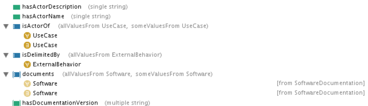
Figura 6.9: Propriedades que descrevem a classe Actor
