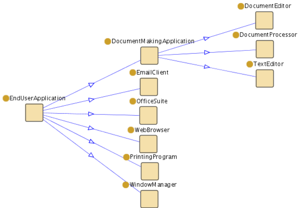
Figura A.7: A classe EndUserApplication e suas subclasses
