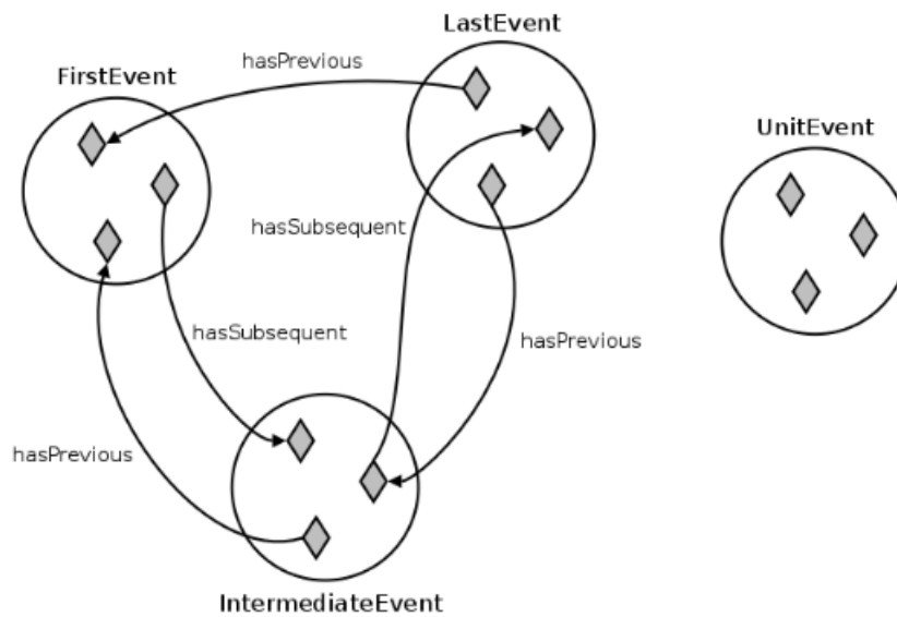
Figura 6.17: As subclasses de Event e o relacionamento entre instâncias [7]
