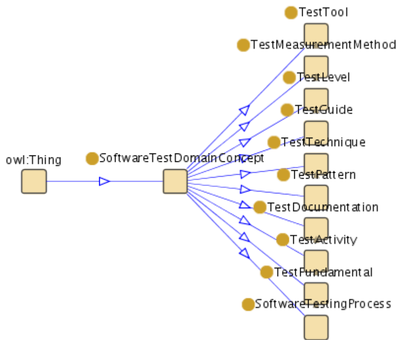
Figura 5.2: SoftwareTestDomainConcept e suas subclasses
