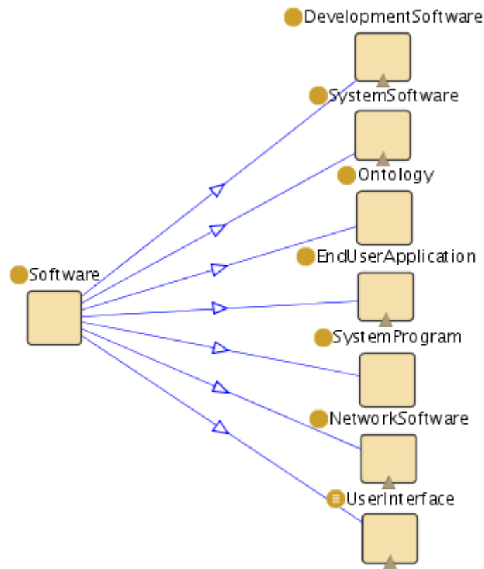
Figura A.5: A classe Software e suas subclasses
