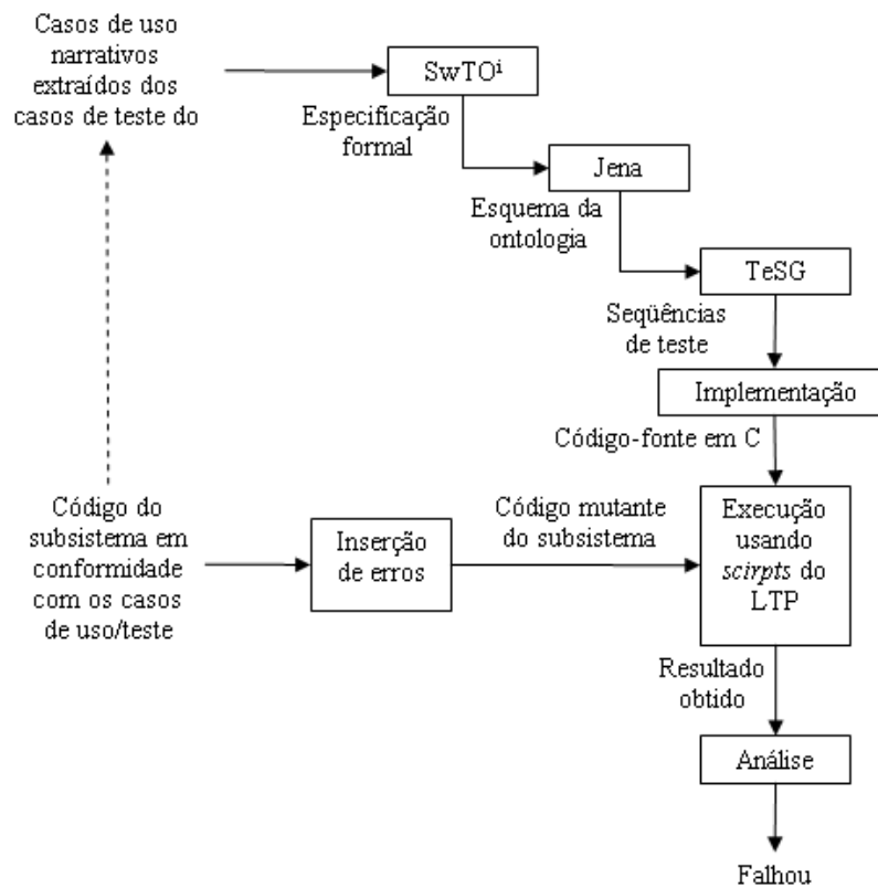
Figura 6.19: Fluxo em alto nível do primeiro experimento da TeSG usando a SwTO I
