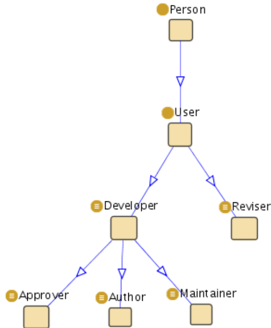
Figura A.3: A classe Person e suas subclasses
