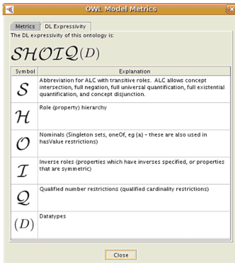
Figura 7.6: Expressividade das ontologias
