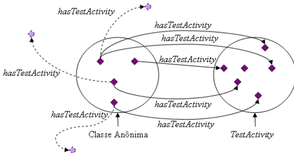
Figura 5.4: Um esquema da restrição existencial ( \exists \text{hasTestActivity} . \text{TestActivity} )
