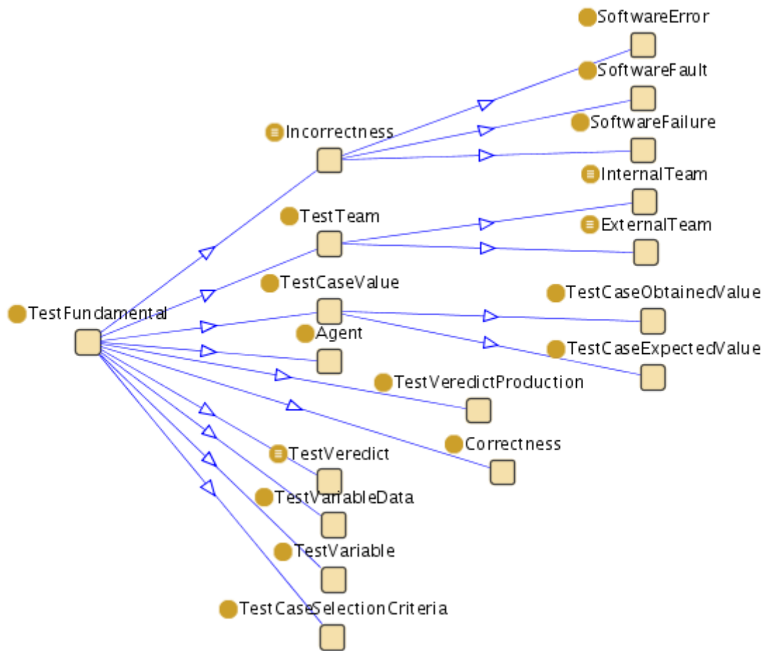
Figura 5.11: TestFundamental e suas subclasses
