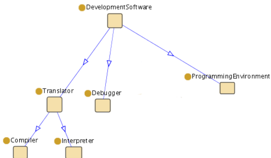
Figura A.6: A classe DevelopmentSoftware e suas subclasses
