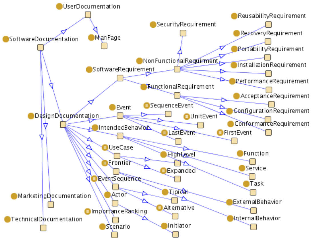
Figura A.11: A classe SoftwareDocumentation e suas subclasses
