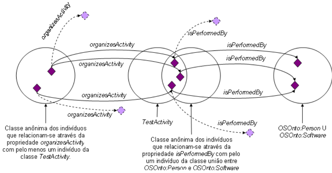
Figura 5.10: Uma descrição da classe TestPlan
