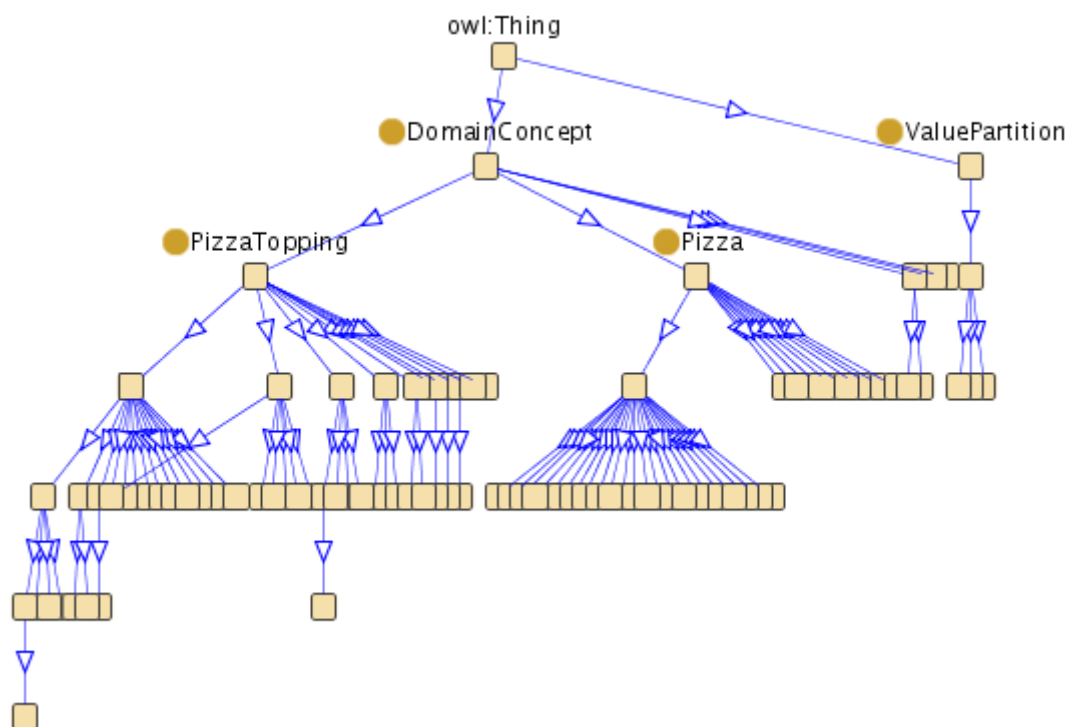
Figura 7.2: Árvore formada por classes e relações é-um da Pizza Ontology
