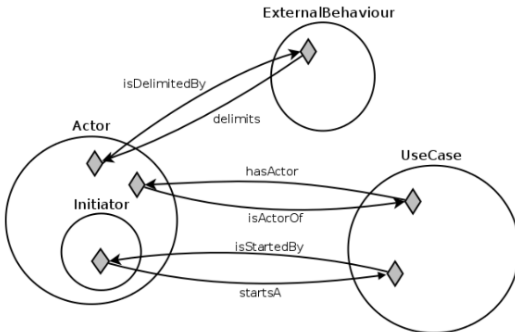
Figura 6.8: Relacionamento entre instâncias da classe Actor , Initiator , External-Behavior e UseCase [7]
