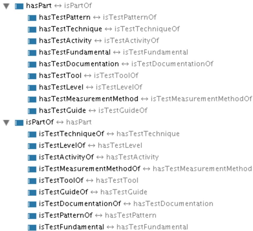
Figura 5.5: Hierarquia das propriedades hasPart e isPartOf
