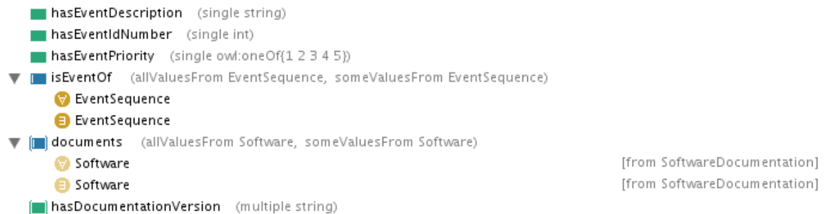
Figura 6.11: Propriedades que descrevem a classe Event
