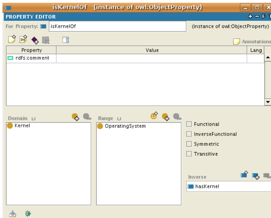
Figura 4.1: Domínio e contradomínio da propriedade isKernelOf
