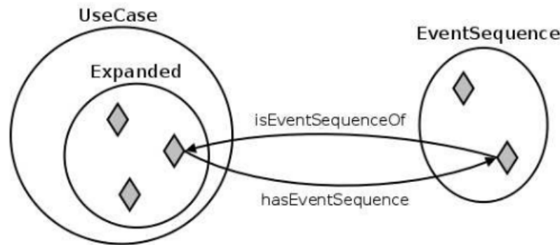
Figura 6.4: Relacionamento entre indivíduos da classe Expanded e EventSequence [7].
