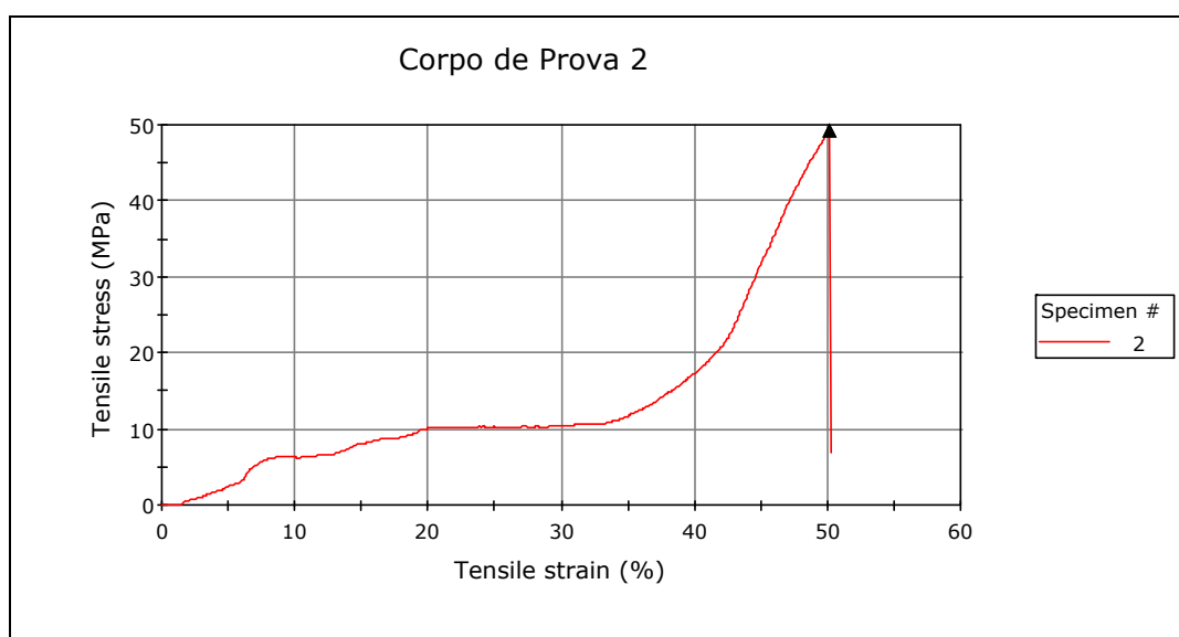
Figura 8 - Resultado do ensaio de tração expresso pela curva tensão x deformação. A seta representa a tensão de ruptura do espécime.
