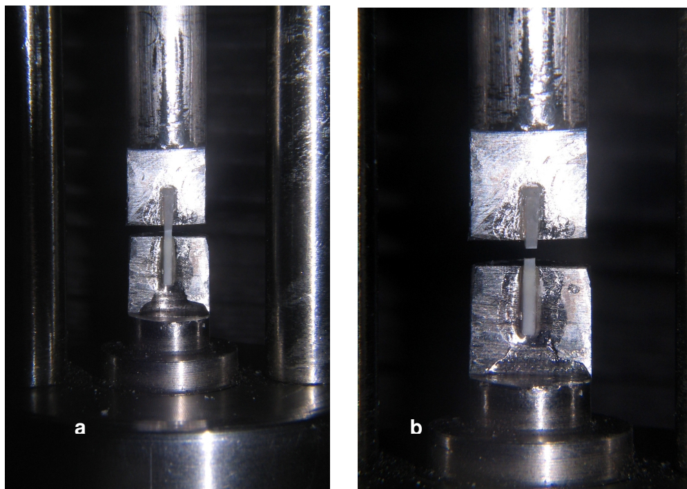
Figuras 7a e 7b - CP submetido ao ensaio de tração (a) até a ruptura da interface adesiva (b)
