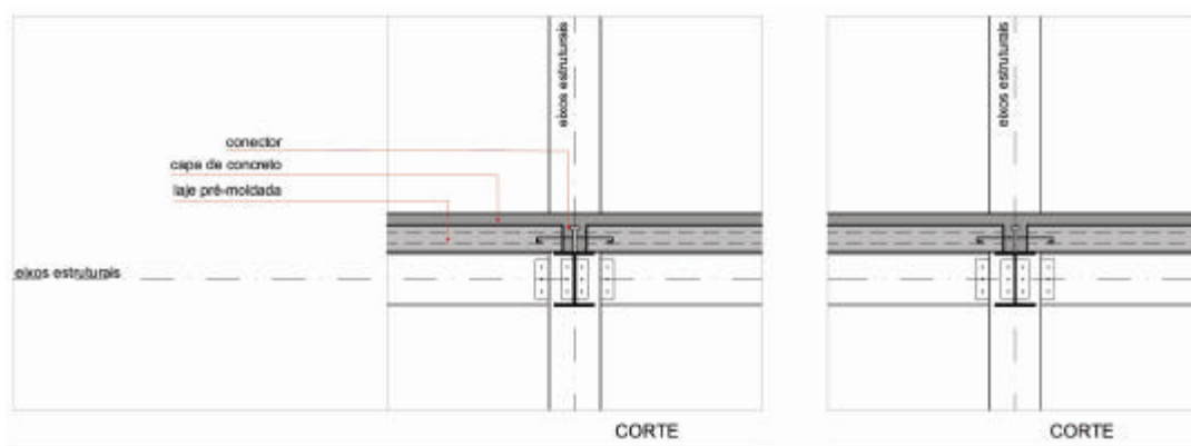
Figura 6.43 - Detalhe construtivo - lajes pré-fabricadas protendidas.
