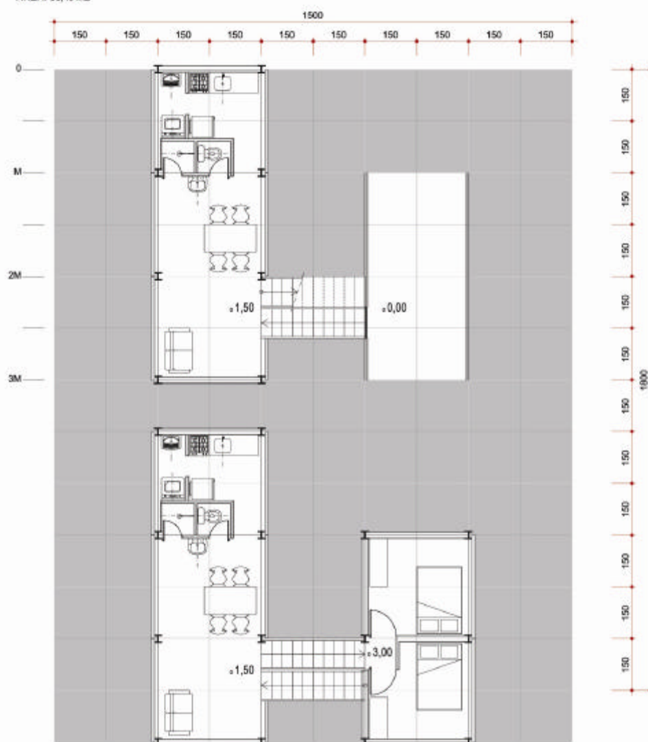
PLANTA
