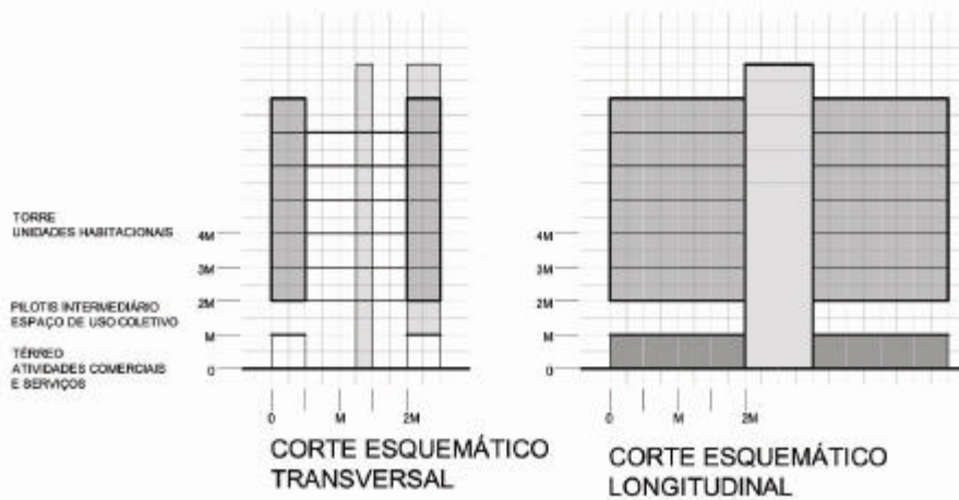
Figura 6.49 – Implantação 03 Planta pavimento tipo, planta pavimento térreo e cortes esquemáticos.
