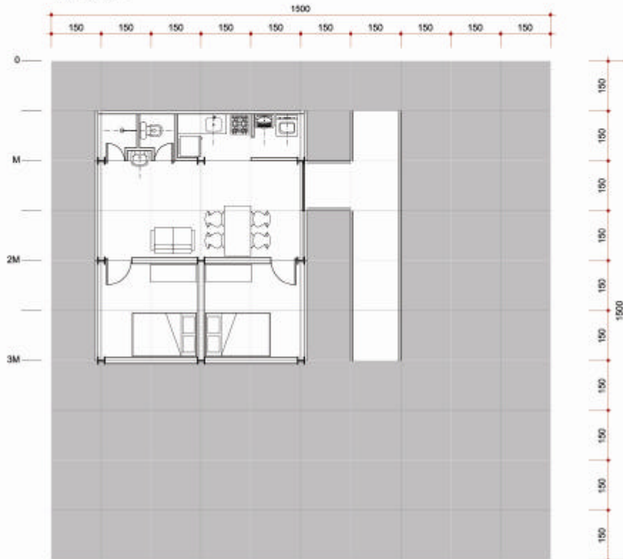
PLANTA
