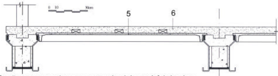
Seção transversal, no encontro das lajes pré-fabricadas com as vigas de piso, espaçadas a cada 2,50 m
