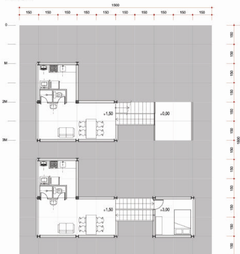
PLANTA
