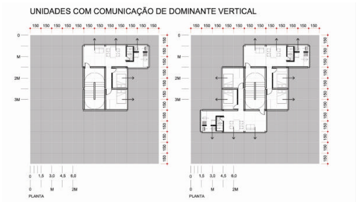
Figura 6.19 – Unidades com comunicações de dominante vertical. Unidades habitacionais poligonais orientadas (aberturas para o exterior) em todas as direções, com capacidade de adição ao longo de dois ou mais eixos verticais.
