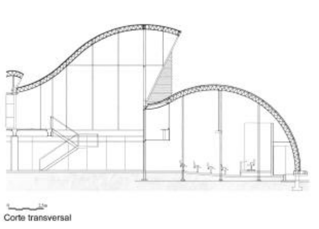
Figura 4.22 – Sede do Tribunal de Contas da União no Estado do Espírito Santo – CTRS – Vitória, ES, Brasil, 1998. Arquiteto: João Filgueiras Lima, Lelé. Corte transversal.
