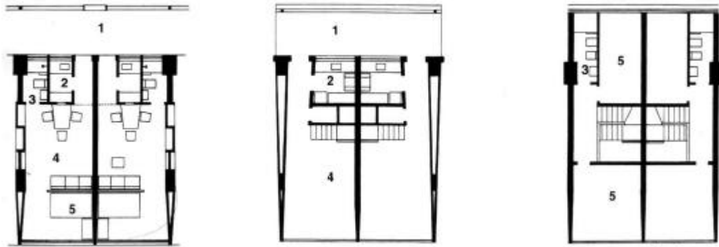
Figura 3.12 - Conjunto Pedregulho, Rio de Janeiro, Brasil, 1946. Arquiteto: Affonso Eduardo Reidy. Apartamento quitinete (1º e 2º pavimentos) e duplex de dois dormitórios (4º, 5º, 6º e 7º pavimentos). Fonte: BONDUKI, 1999.
