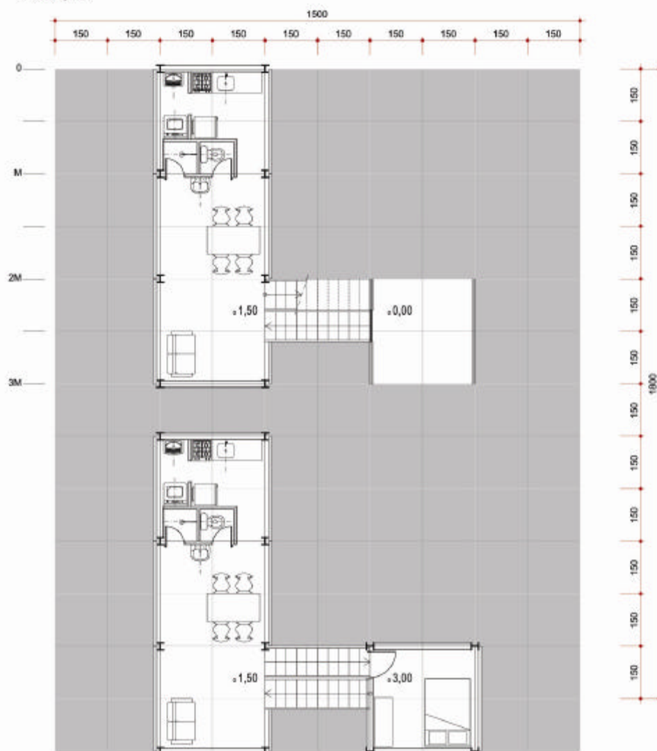
PLANTA
