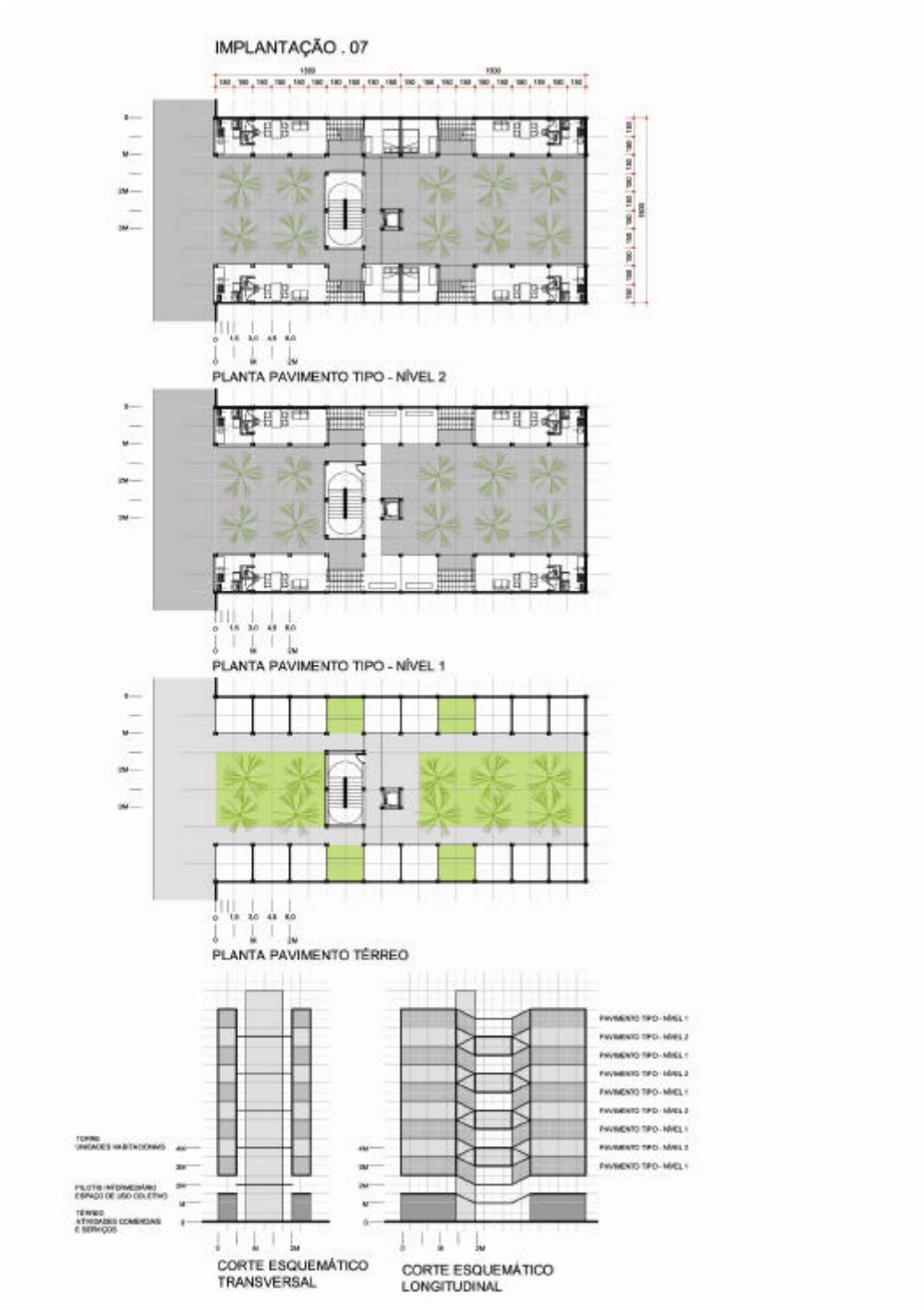
Figura 6.57 – Implantação 07 Planta pavimento tipo, planta pavimento térreo e cortes esquemáticos.
