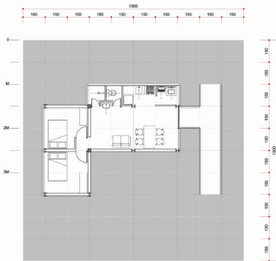
PLANTA
