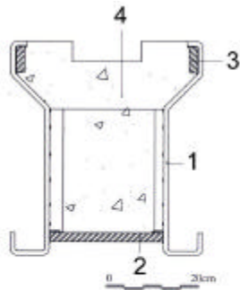
Seção transversal - VP - 1 das vigas de piso: aço-concreto
