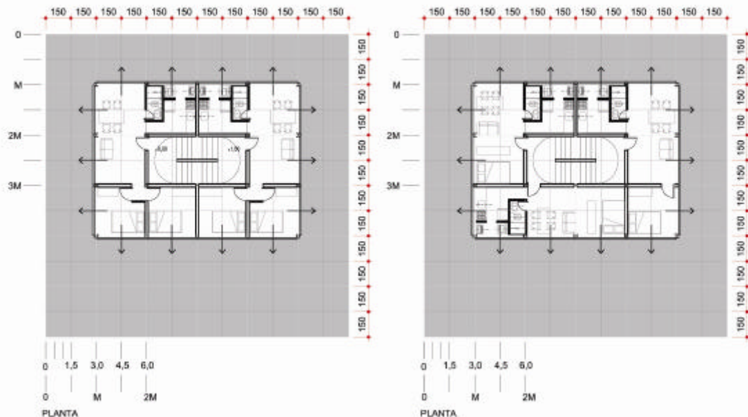
Figura 6.20 – Unidades com comunicações de dominante vertical. Unidades habitacionais isoladas, orientadas (aberturas para o exterior) em todas as direções, com capacidade de adição ao longo de um único eixo vertical.
