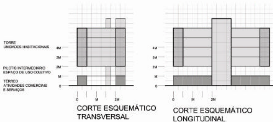
Figura 6.51 – Implantação 04 Planta pavimento tipo, planta pavimento térreo e cortes esquemáticos.
