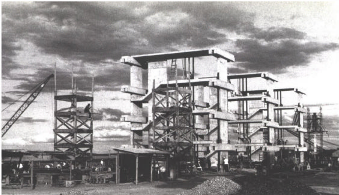
Figura 4.4 – Apartamentos para professores da Universidade de Brasília – Brasília, DF, 1962. Arquiteto: João Filgueiras Lima, Lelé. Foto do edifício e Conjunto de circulação vertical fundido no local durante a obra.
