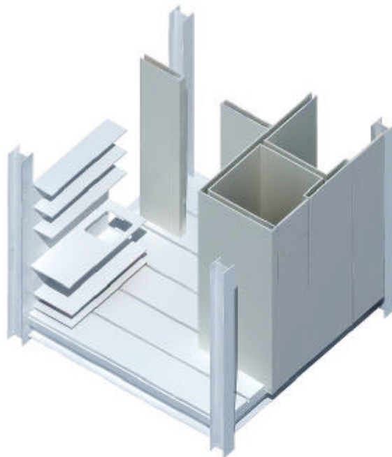
Figura 6.5 - Núcleo hidráulico – perspectivas isométricas. O núcleo hidráulico é formado por um módulo de 3m x 3m x 3m ou por duas metades do mesmo módulo. Área: 9,00 m 2 .
