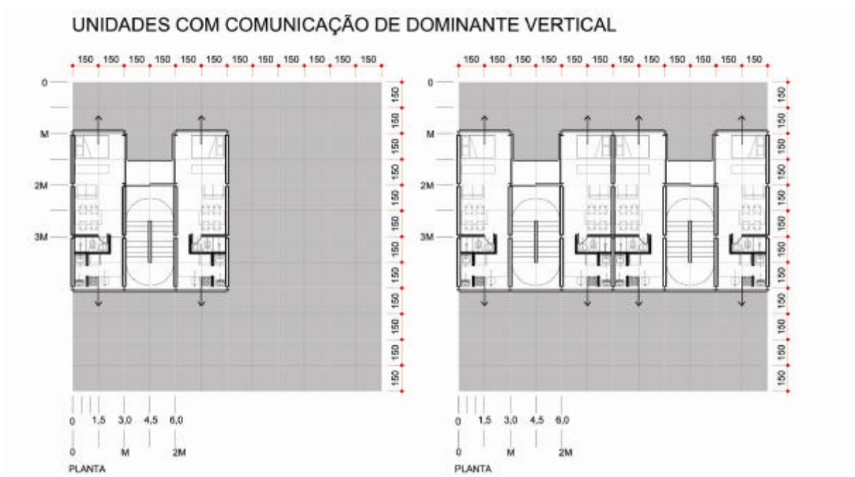
Figura 6.18 – Unidades com comunicações de dominante vertical. Unidades habitacionais orientadas (aberturas para o exterior) em duas direções, com capacidade de adição ao longo de um eixo vertical.
