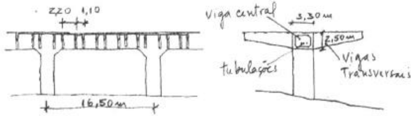
Figura 4.9 – Secretarias do Centro Administrativo da Bahia – Salvador, BA, Brasil, 1973. Arquiteto: João Filgueiras Lima, Lelé. Croqui do sistema estrutural, plataforma elevada.
