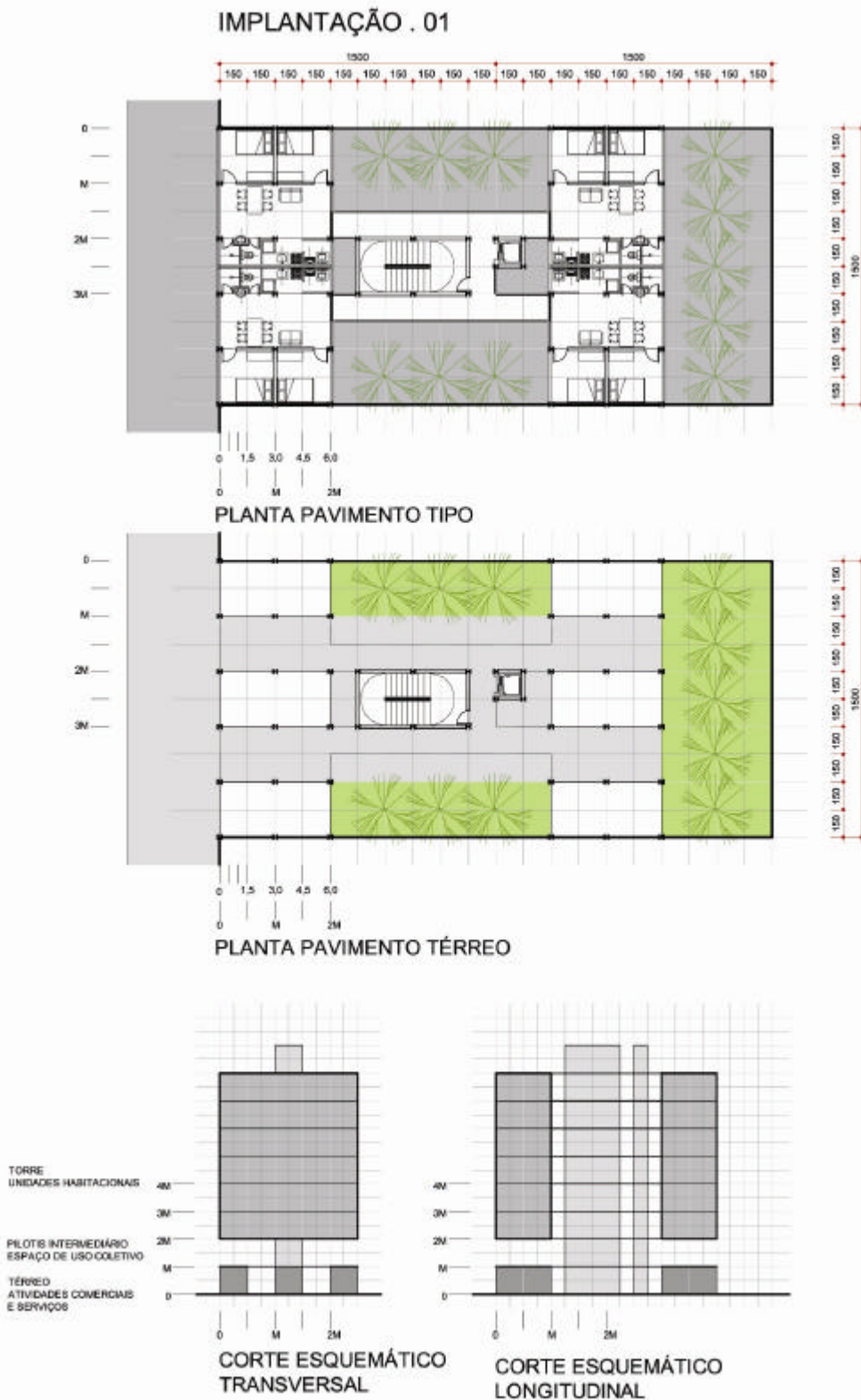
Figura 6.45 – Implantação 01 Planta pavimento tipo, planta pavimento térreo e cortes esquemáticos.
