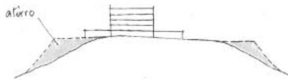
Figura 4.5 – Secretarias do Centro Administrativo da Bahia – Salvador, BA, Brasil, 1973. Arquiteto: João Filgueiras Lima, Lelé. Croqui da implantação, corte esquemático. Situação não desejada: blocos colados ao solo.
