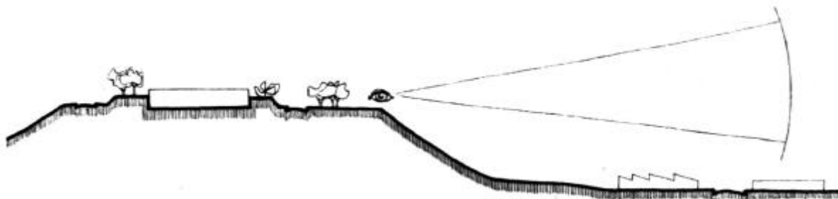
Figura 3.8 – Conjunto Pedregulho, Rio de Janeiro, Brasil, 1946. Arquiteto: Affonso Eduardo Reidy. Situação topográfica do morro do Pedregulho. Fonte: BONDUKI, 1999.
