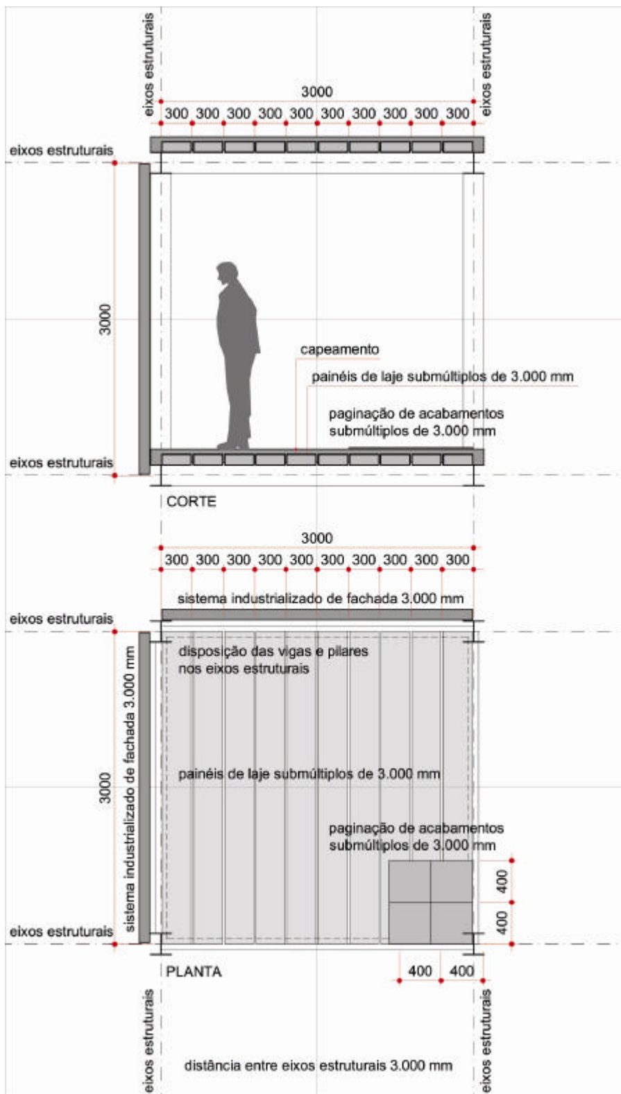
Figura 6.29 - Coordenação modular entre estrutura, sistemas de lajes, sistemas de vedações e acabamentos. Planta e corte de um módulo típico – 3x3m, com vedações externas.
