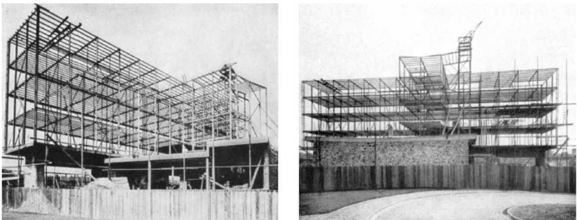
Figura 3.5 – Pavilhão Suíço, Paris, França, 1931. Arquiteto: Le Corbusier. Construção, estrutura metálica sobre embasamento de concreto. Fonte: PUNTONI, 2004.
