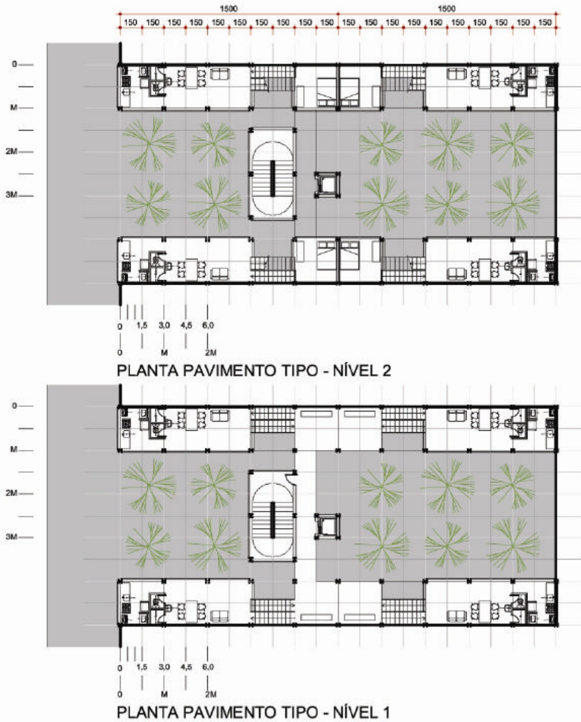
Figura 6.58 – Implantação 07 Planta pavimento tipo ampliada.
