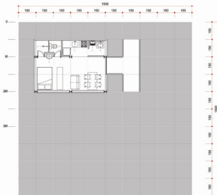
PLANTA
