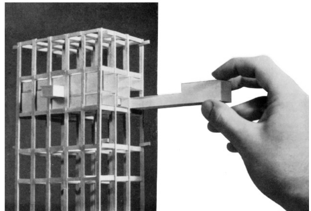
Figura 3.7 – Unidade Habitacional de Tamanho Adequado, Marselha, França, 1946-51. Arquiteto: Le Corbusier. Construção, macro estrutura em concreto e infra estrutura em aço. Unidades independentes da estrutura. Fonte: PUNTONI, 2004.
