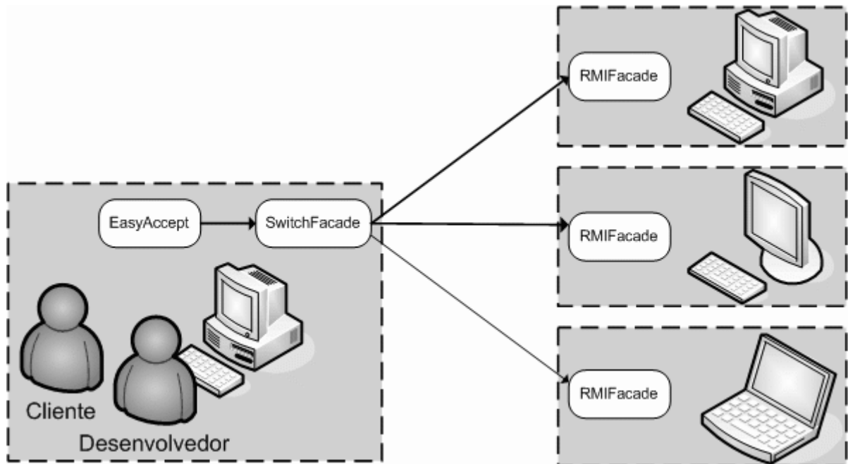
Figura 37 – EasyAccept distribuído
