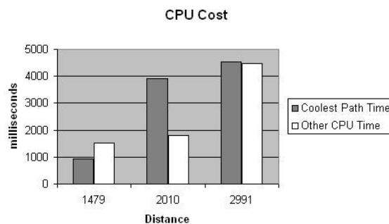
Figura 5.22 Gráfico do tempo de execução de uma consulta a-autonomy com a igual a 900 metros
