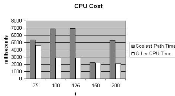
Figura 5.24 Gráfico do tempo de execução de uma consulta t-autonomy com distância de rede fixa em 2991 metros
