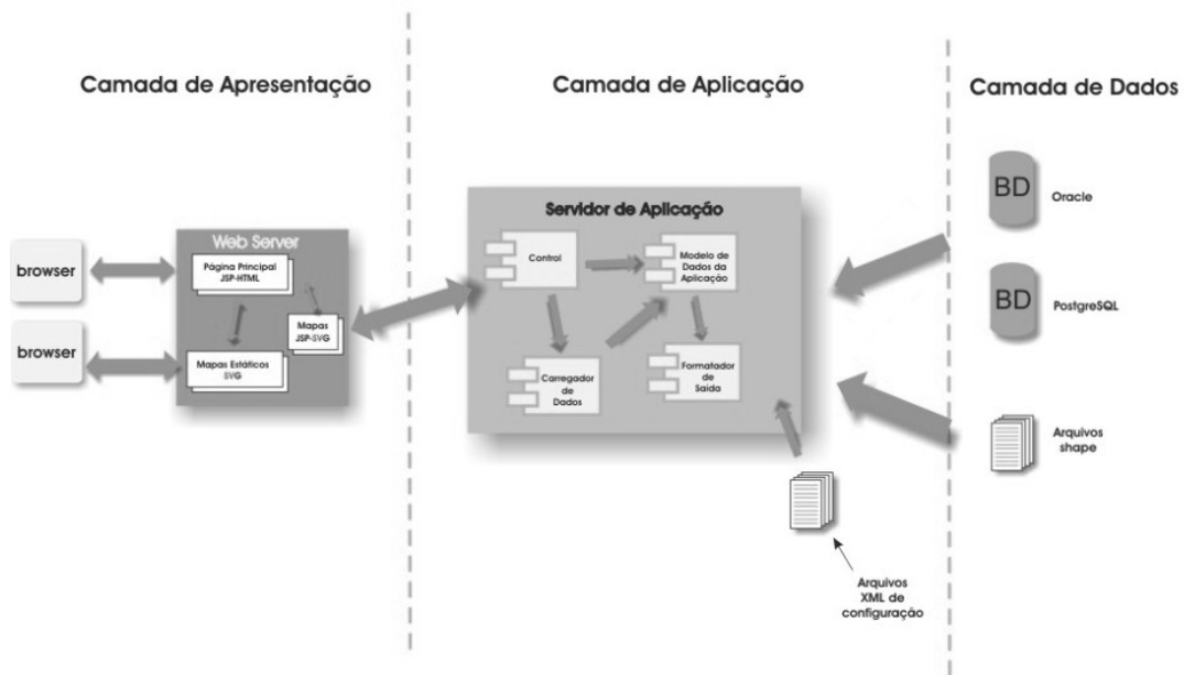
Figura 2.1 Arquitetura do iGIS
