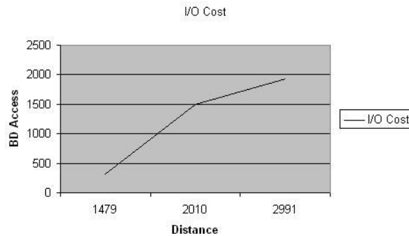
Figura 5.23 Gráfico do custo de acesso ao banco de dados de uma consulta a-autonomy com a definido como sendo 900 metros
