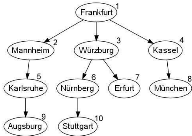
Figura 2.3 Árvore de caminamento de uma Busca em Largura (fonte: [Wik07a])
