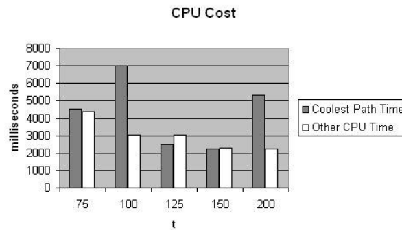
Figura 5.27 Gráfico do tempo de execução de uma consulta t -autonomy com o parâmetro fastest sendo de Muita Importância
