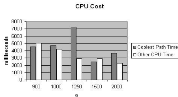
Figura 5.21 Gráfico do tempo de execução de uma consulta a-autonomy com o parâmetro fastest sendo de Muita Importância
