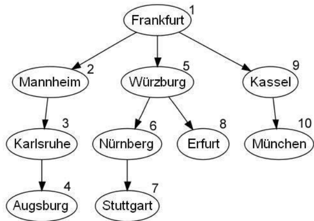
Figura 2.4 Árvore de caminamento de uma Busca em Profundidade (fonte: [Wik07a])
