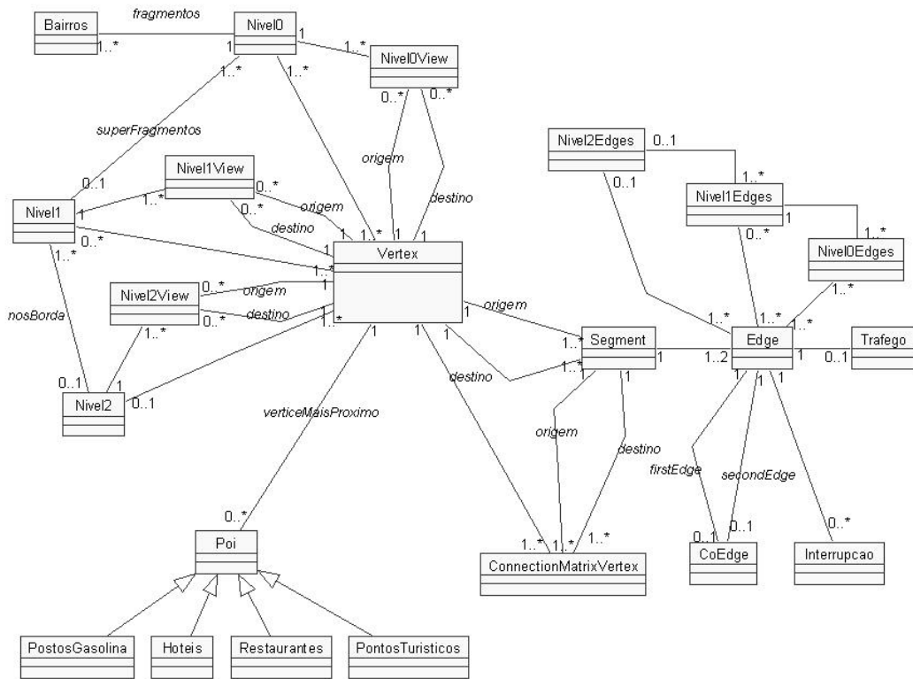
Figura 5.1 Esquema lógico do banco de dados
