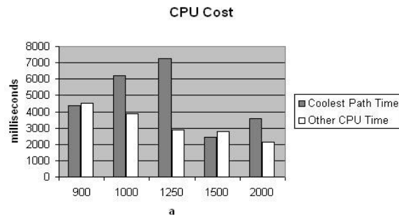
Figura 5.20 Gráfico do tempo de execução de uma consulta a-autonomy com o parâmetro shortest sendo de Muita Importância
