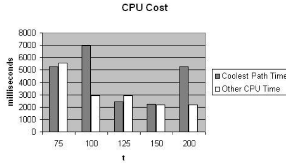
Figura 5.26 Gráfico do tempo de execução de uma consulta t -autonomy com o parâmetro shortest sendo de Muita Importância
