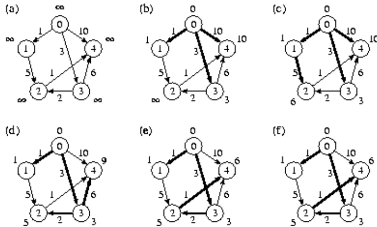
Figura 2.5 Passo a passo da execução do algoritmo de Dijkstra (fonte: [Ziv03])
