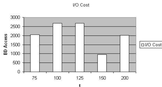
Figura 5.25 Gráfico do custo de acesso ao banco de dados de uma consulta t-autonomy com distância de rede fixa em 2991 metros
