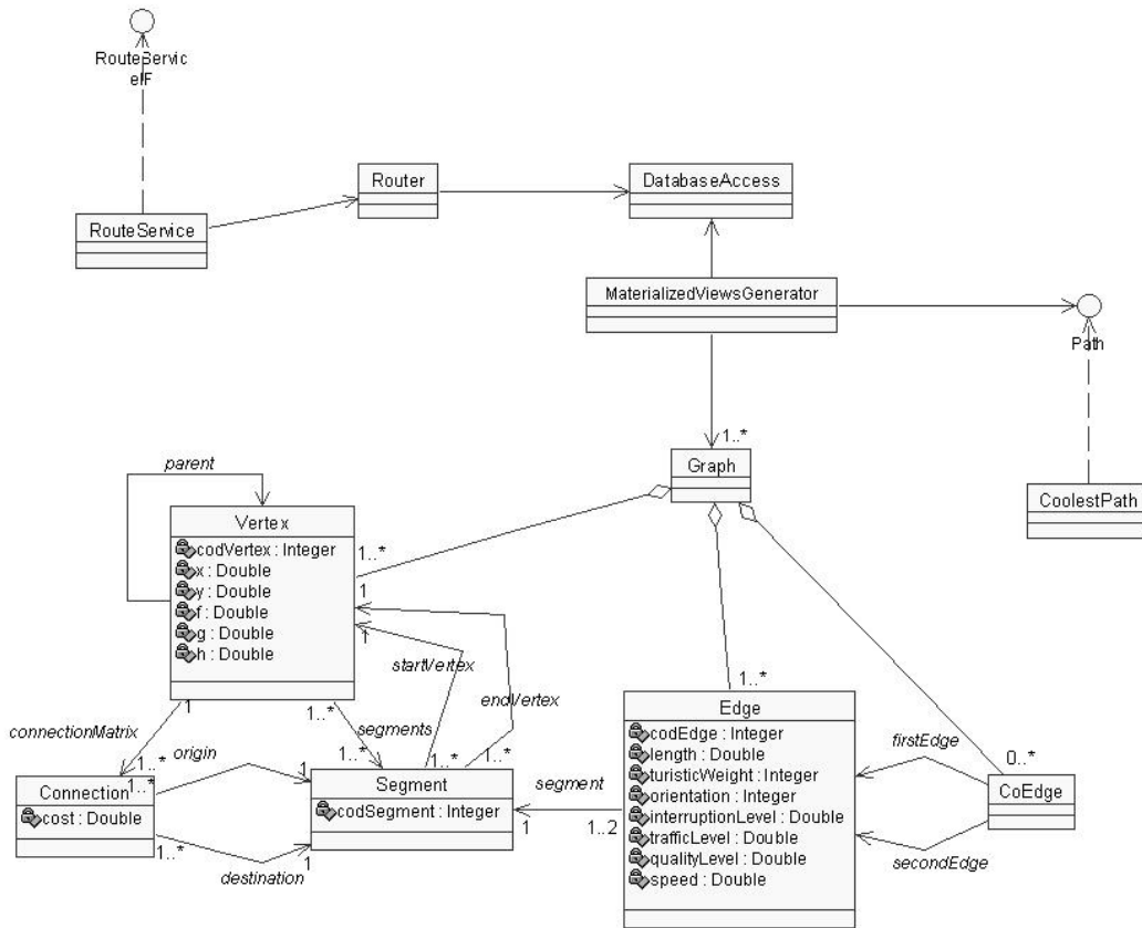
Figura 4.3 Diagrama de classes do serviço de rotas
