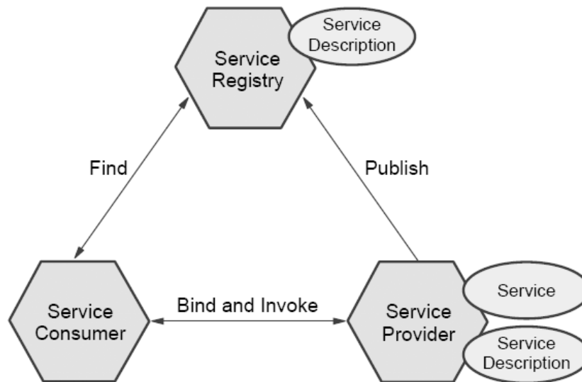
Figura 4.1 Componentes básicos de um Web service (fonte: [EAA+04])
