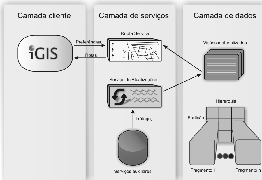
Figura 4.2 Arquitetura do sistema de busca de rotas
