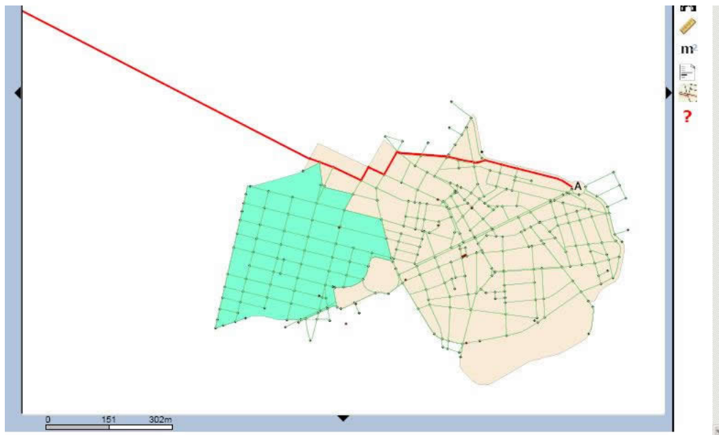
Figura 5.15 Caminho a-autonomy partindo de A, com a = 10000 , tipo de PoI = qualquer
