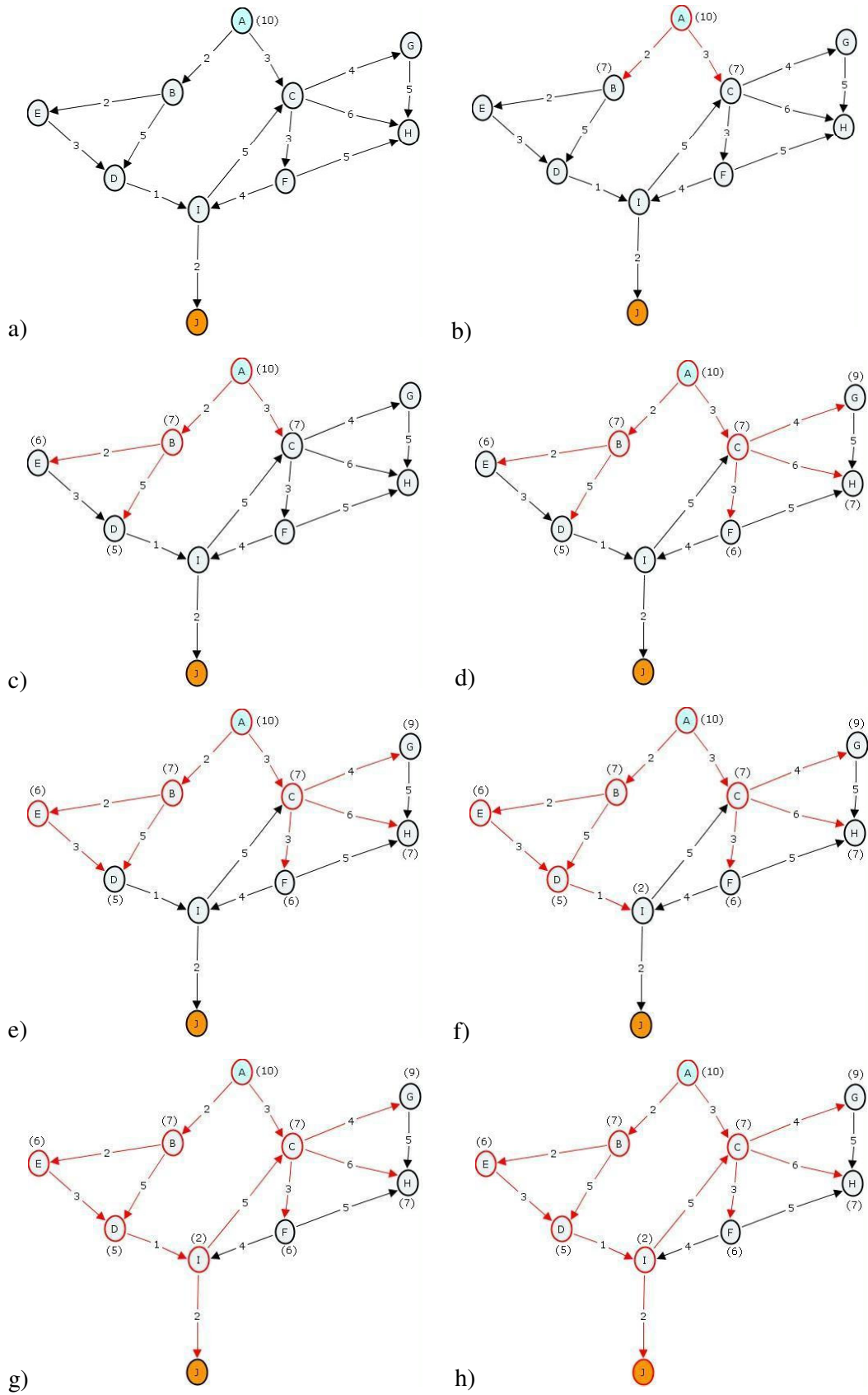
Figura 2.6 Execução do algoritmo A* em um grafo
