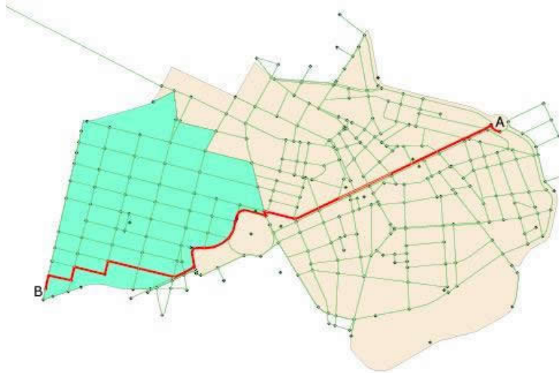
Figura 5.3 Rota de A a B maximizando o parâmetro shortest
