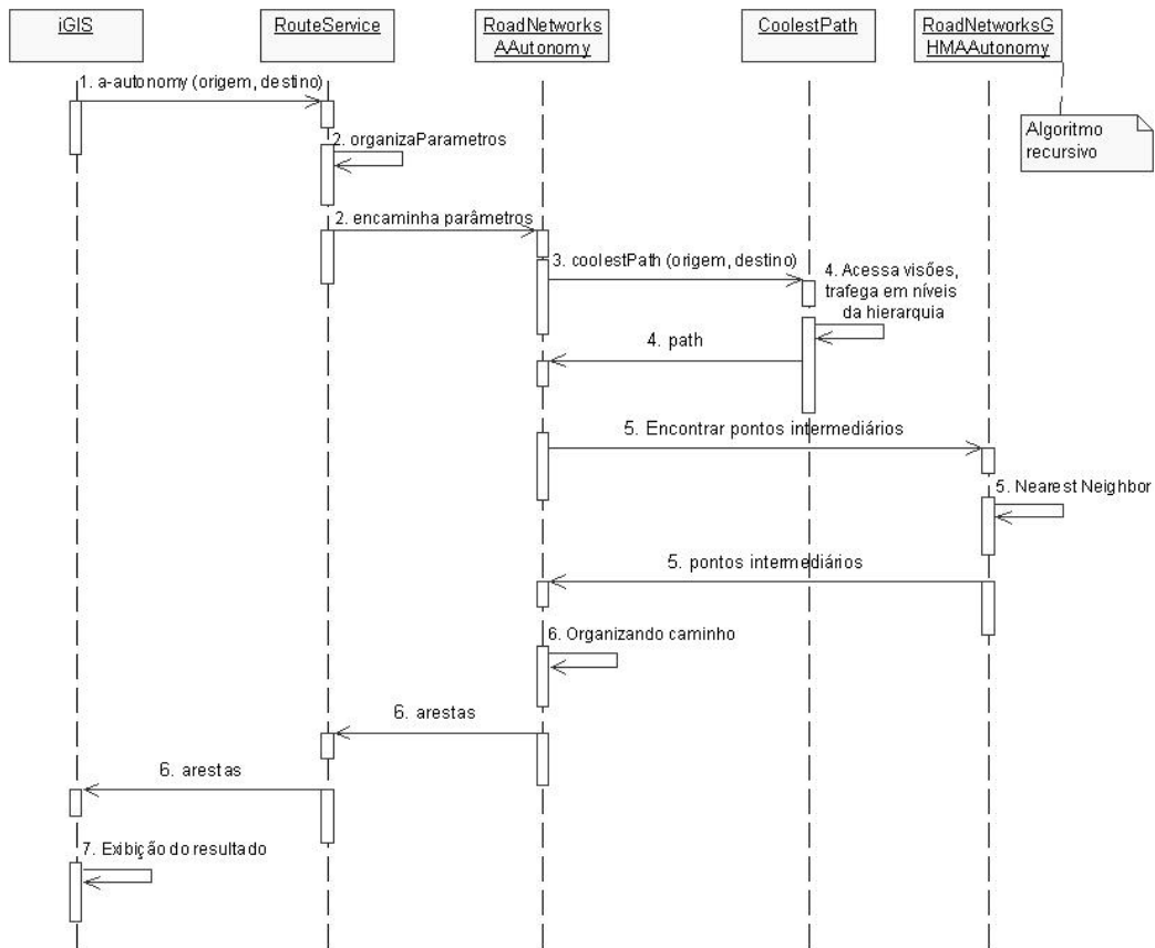
Figura 4.6 Diagrama de seqüência de uma operação a-autonomy
