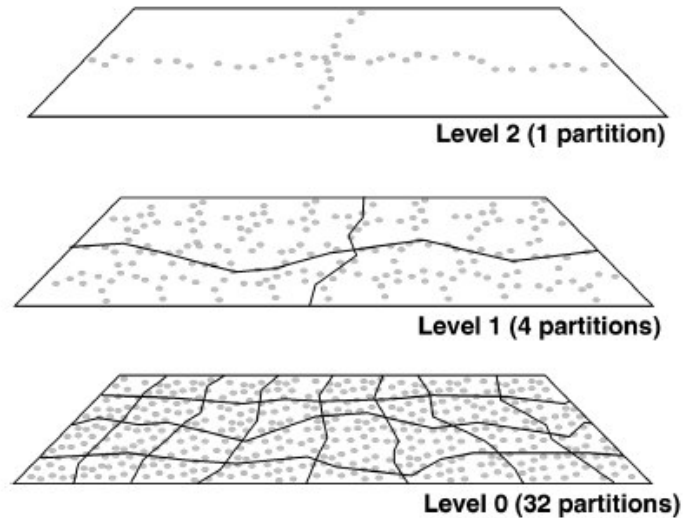
Figura 2.11 Exemplo de hierarquia em três níveis (fonte: [JHR98])
