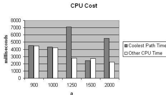
Figura 5.18 Gráfico do tempo de execução de uma consulta a-autonomy com distância de rede fixa em 2991 metros
