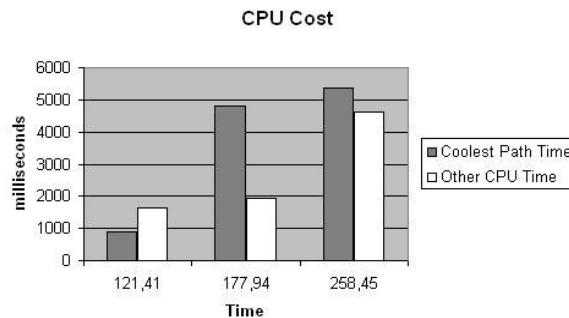
Figura 5.28 Gráfico do tempo de execução de uma consulta t -autonomy com t fixo em 75 segundos
