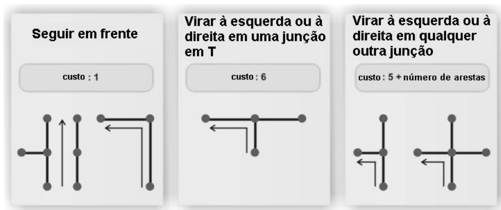
Figura 3.1 Custos das transições entre arestas
