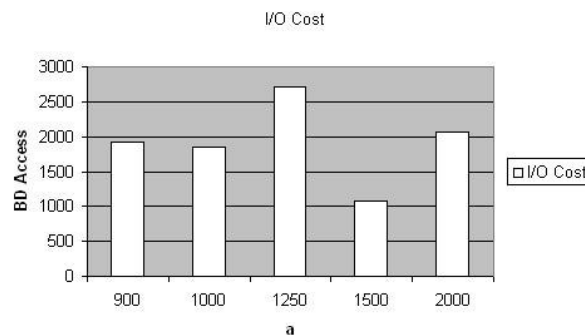
Figura 5.19 Gráfico do custo de acesso ao banco de uma consulta a-autonomy com distância de rede fixa em 2991 metros
