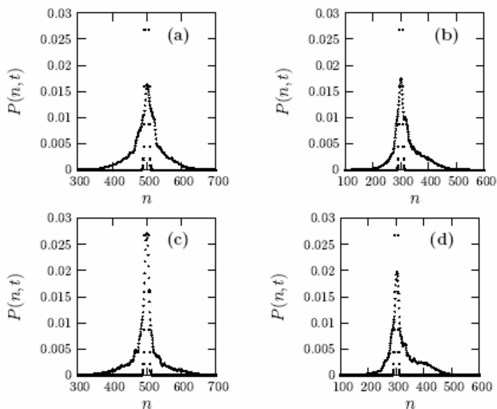
Figura 2.14 - Comparação entre os casos estudados por Wells e colaboradores. Sistema randômico sem campo elétrico (a) e com campo elétrico (b); Sistema fractal sem campo elétrico (c) e com campo elétrico (d). Surgimento de difusão assimétrica em um sistema com desordem e anisotrópico. A distribuição inicial está representada na figura por pontos [Wells et al. , 2005].
