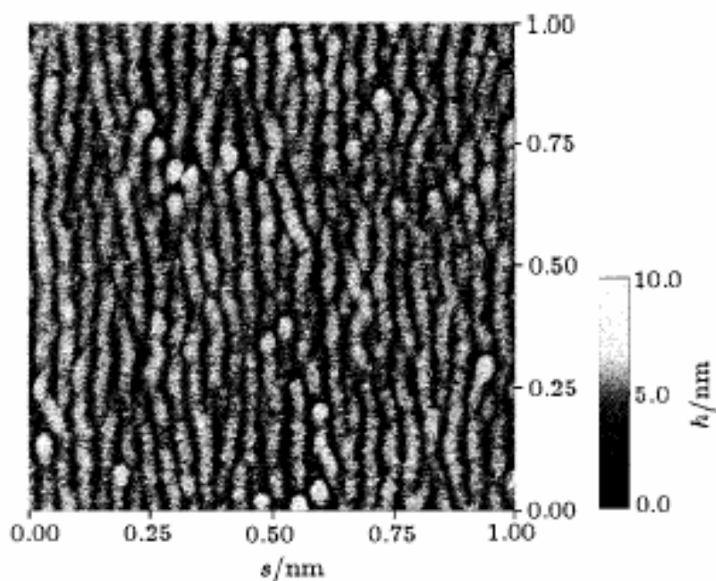
Figura 2.7 - Fios quânticos de InGaAs arranjados ordenadamente sobre conjunto de degraus por MBE assistida por hidrogênio atômico [Da-Yong et al. , 2003].
