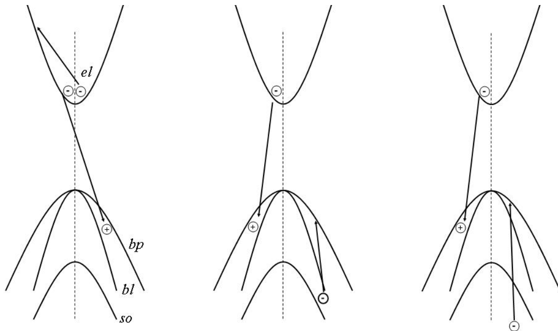
Figura 2.3 - Diferentes processos possíveis de recombinação Auger banda-banda em um semicondutor de gap direto.
