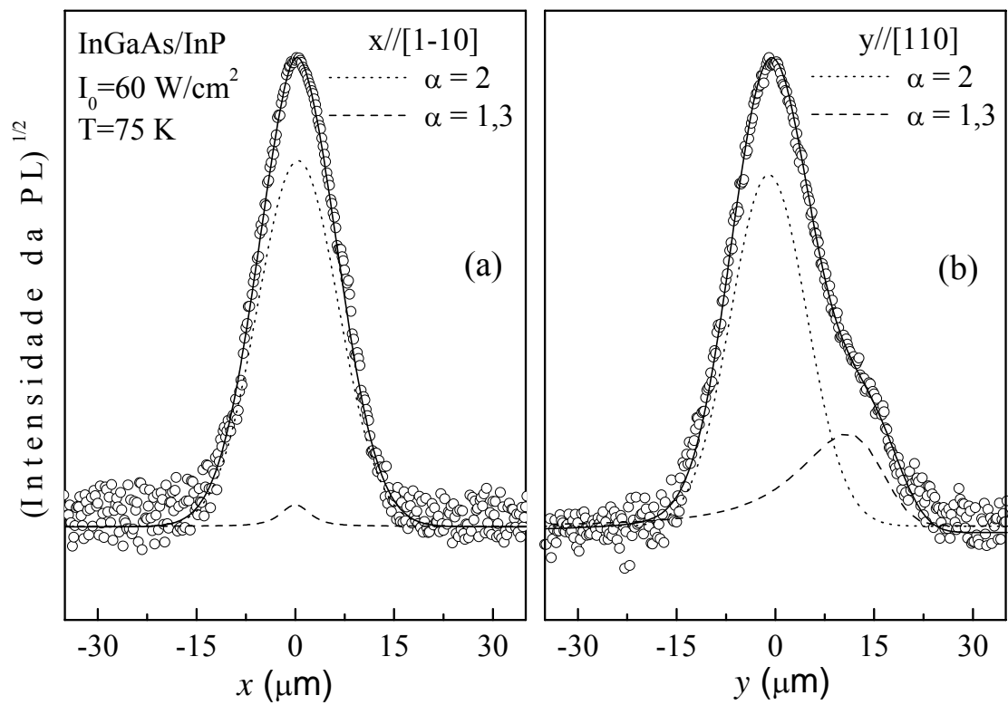
Figura 5.2 - Raiz quadrada dos perfis de intensidade da fotoluminescência (I_{PL})^{1/2} ao longo de dois eixos ortogonais que se cruzam no centro do spot de excitação. As linhas sólidas representam o melhor ajuste dos dados experimentais, como discutido no texto.
