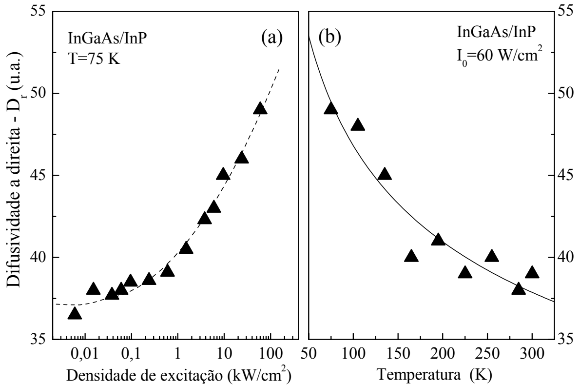
Figura 5.8 – Dependência da Difusividade D_r como função da (a) densidade de excitação e (b) da temperatura. A linha sólida representa o melhor ajuste obtido com D_r \propto T/T^{-a} . A linha pontilhada é somente guia para os olhos.
