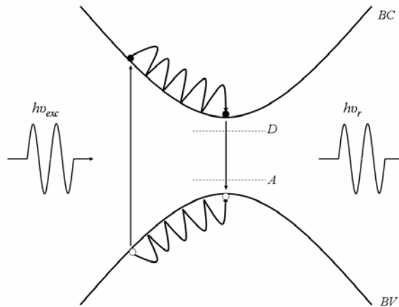
Figura 2.2 - Representação esquemática dos processos de absorção, termalização e recombinação radiativa presentes em experimentos de PL. BC e BV representam as bandas de condução e de valência, respectivamente. D e A representam os eventuais níveis de impurezas doadoras (D) e aceitadoras (A) presentes no material.
