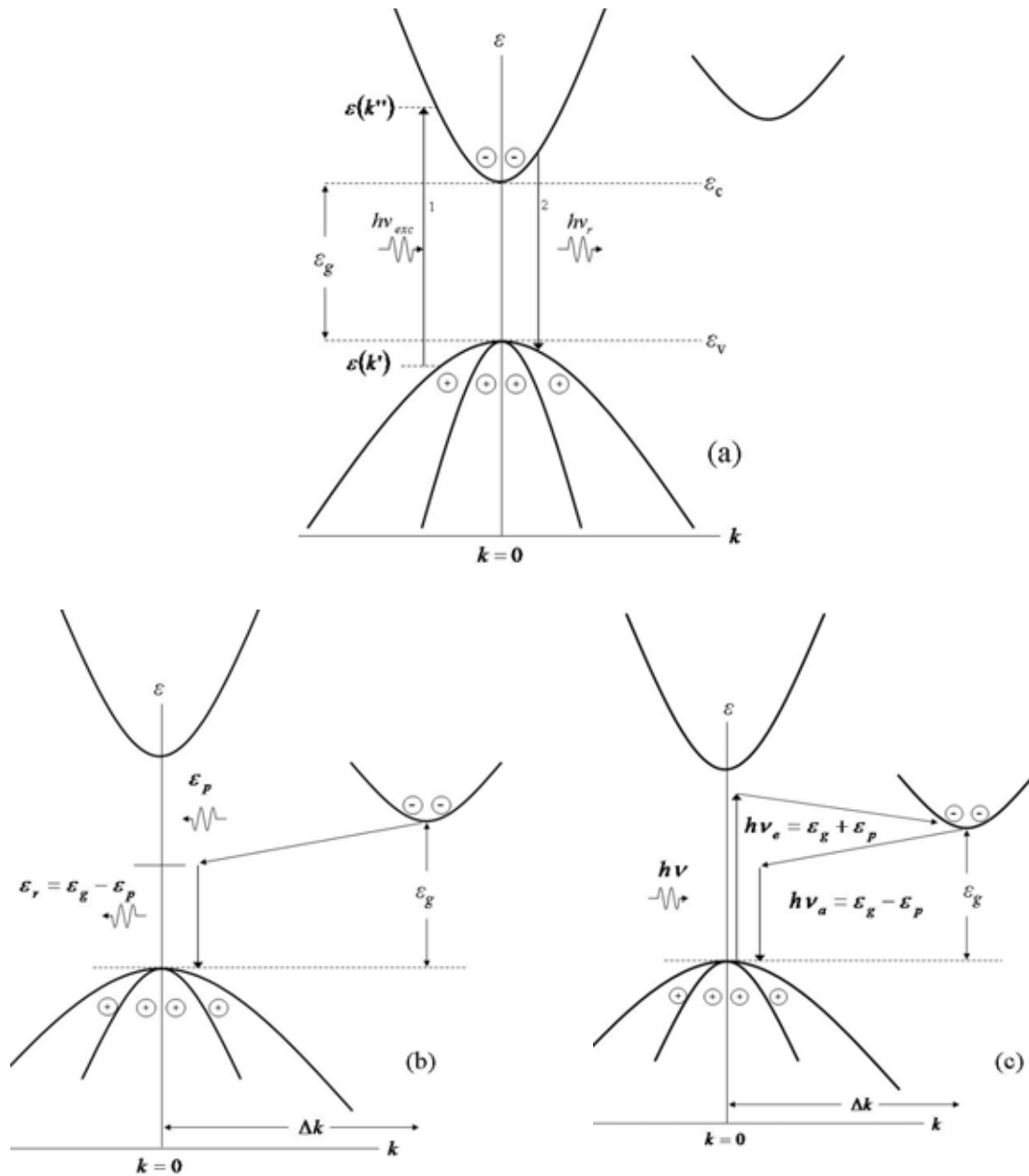
Figura 2.1 – Esquema dos processos de absorção e recombinação banda a banda em (a) semicondutor de gap direto, (b) e (c) semicondutores de gap indireto.
