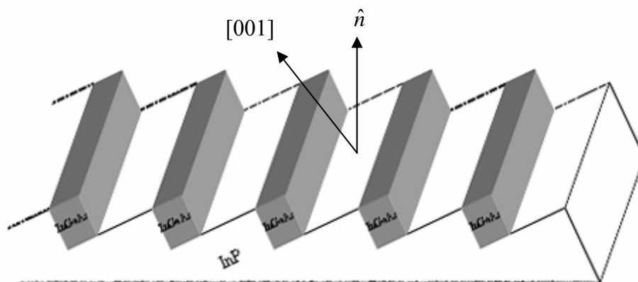
Figura 3.2 - Morfologia das amostras de fios quânticos usadas neste trabalho.
