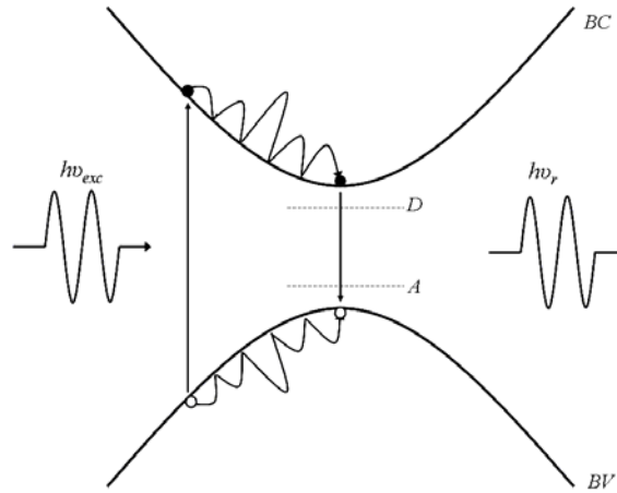
Figura 2.1: Representação dos processos de absorção, termalização e recombinação radiativa presentes em experimentos de PL. BC representa a banda de condução e BV representa a banda de valência.
