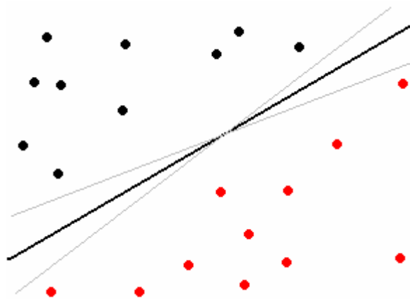
Figura 14: Hiperplano de separação de duas classes
