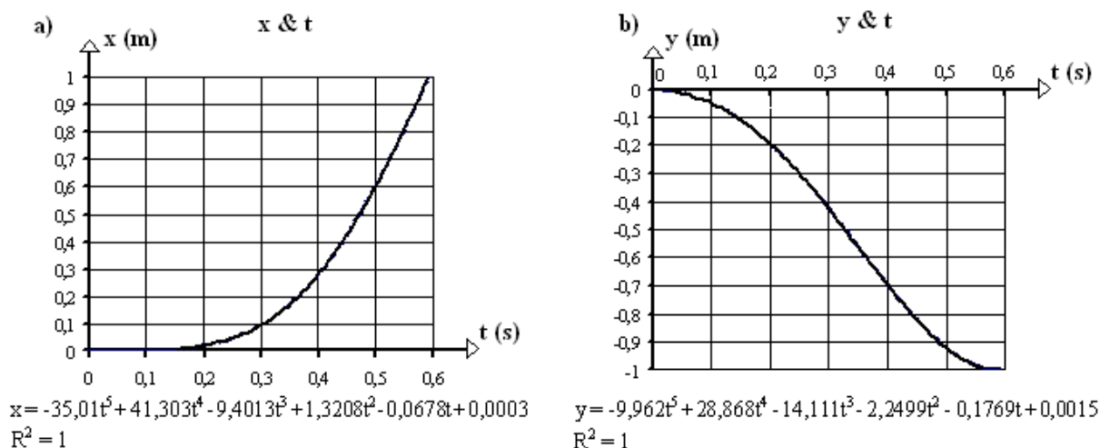
Figura A.5 – Gráfico e função de Regressão dos dados de posição em função do tempo. a) x \text{ & } t ; b) y \text{ & } t
