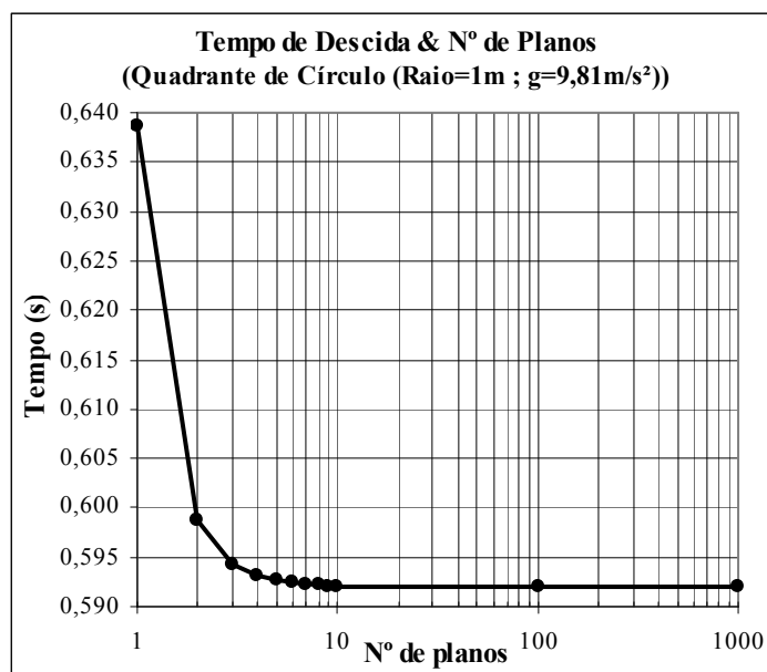
Figura A.4 – Tempo de descida & N° de Planos [1;1000]
