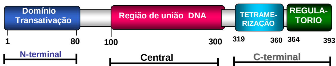
Figura 4: estrutura da proteína p53, modificado de Prokocimer&Rotter, 1994
