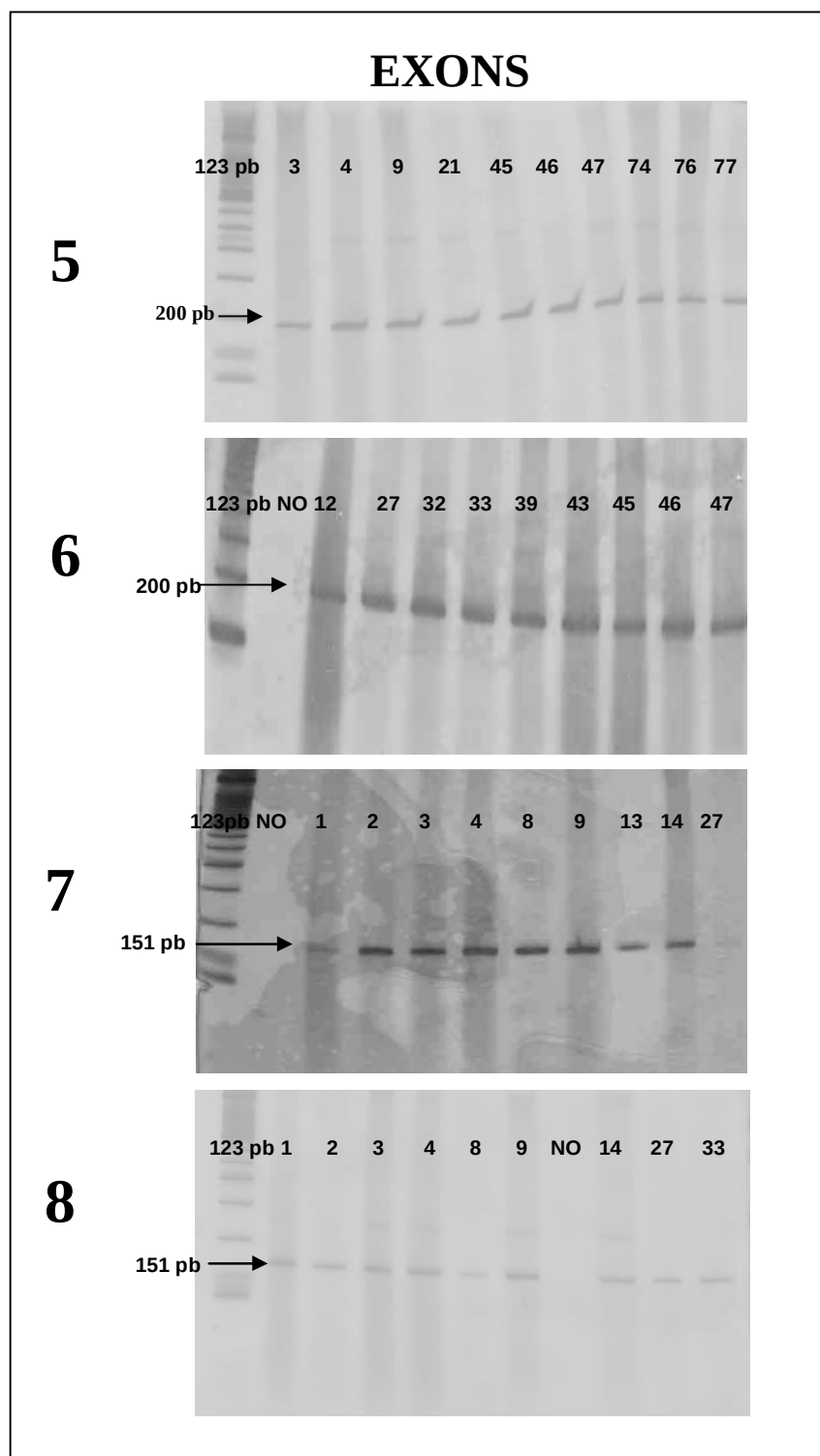
Figura 10: Padrão de bandas encontrado para o gene TP53 exons 5, 6, 7 e 8, em gel de poliacrilamida 7%
