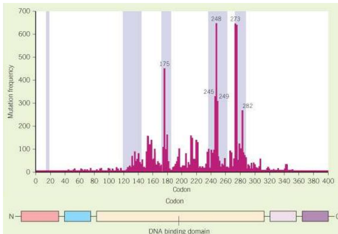
Figura 5: sítios e frequência de mutações do gene TP53 para todos os câncers. Hernandez-Boussard et al, 1999.
