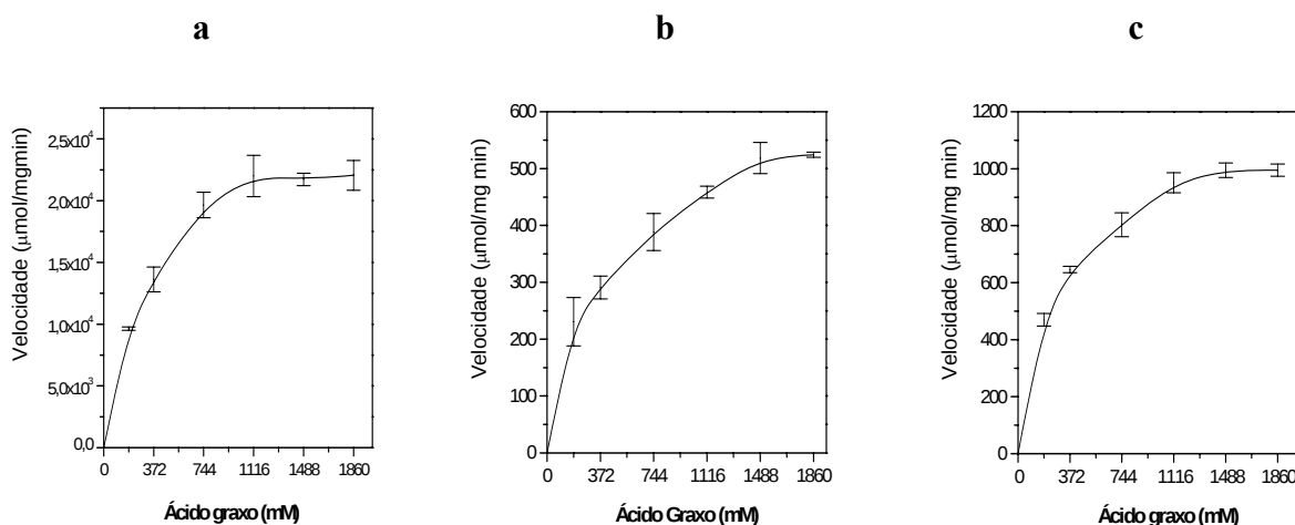
Figura 4.12. Atividades hidrolíticas da lipase livre (a) e imobilizada em POS-PVA ativado com glutaraldeído (b) e epiclorigrina (c) em função da concentração de substrato (expressa em conteúdo total de ácidos graxos contidos em emulsões azeite de oliva/ água) nas condições previamente estabelecidas.
