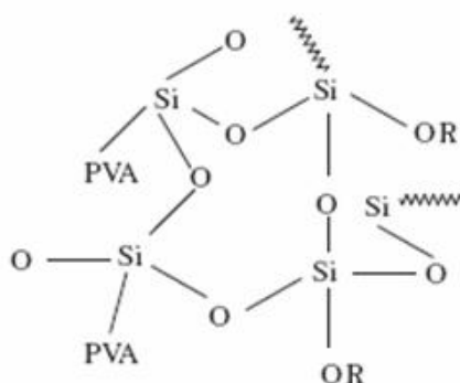
Figura 2.9. Estrutura da matriz polissiloxano-álcool polivinílico (POS-PVA).
