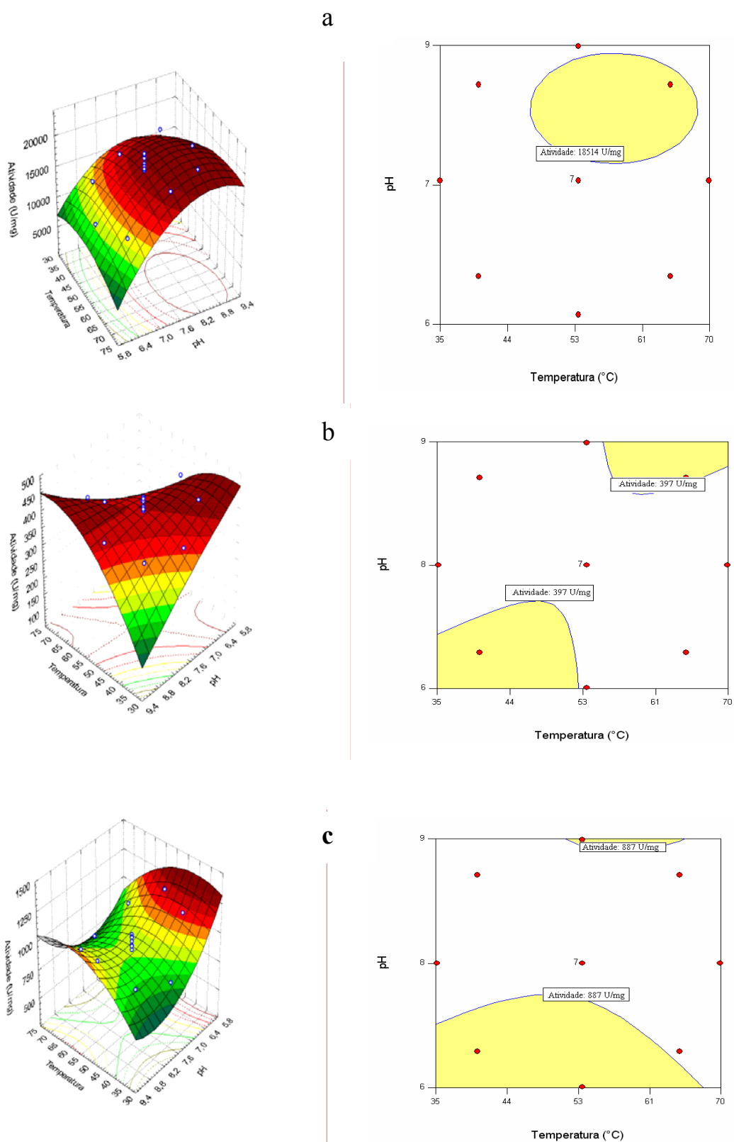
Figura 4.11. Superfícies de resposta e curvas de nível para a atividade da lipase AK livre (a), imobilizada em POS-PVA ativado com glutaraldeído (b) e epícloridrina (c) em função do pH e da temperatura.
