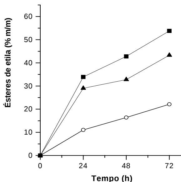
Figura 4.8. Perfil de formação dos monoésteres de etila em função do tempo na reação de etanolise do óleo de palma catalisada pela lipase AK livre (○) e imobilizada em POS-PVA ativado com glutaraldeído (▲) e epicloridrina (■). Razão molar óleo/etanol (1:18) a 40°C.
