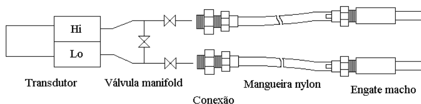
Figura 3.9 – Montagem dos transmissores de pressão.
