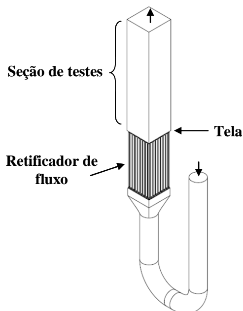
Figura 4.8 – Geometria que antecede a seção de testes.
