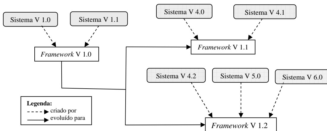
Figura 5 – Grafo de controle de versão de framework e dos sistemas gerados (adaptado de CAGNIN, 2005a)
