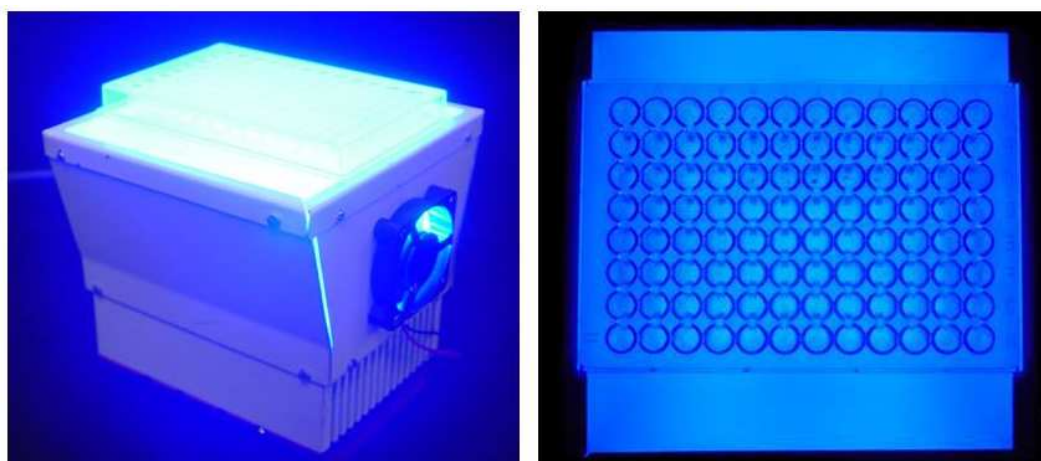
FIGURA 7 – Placa de orifícios posicionada sobre a superfície de iluminação da Bio Table acionada.
