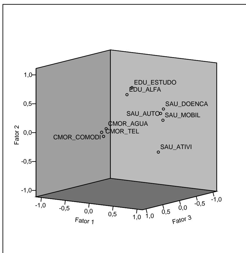
Gráfico 4.10 – Variáveis com relação aos fatores - Minas Gerais, rural, 2003
