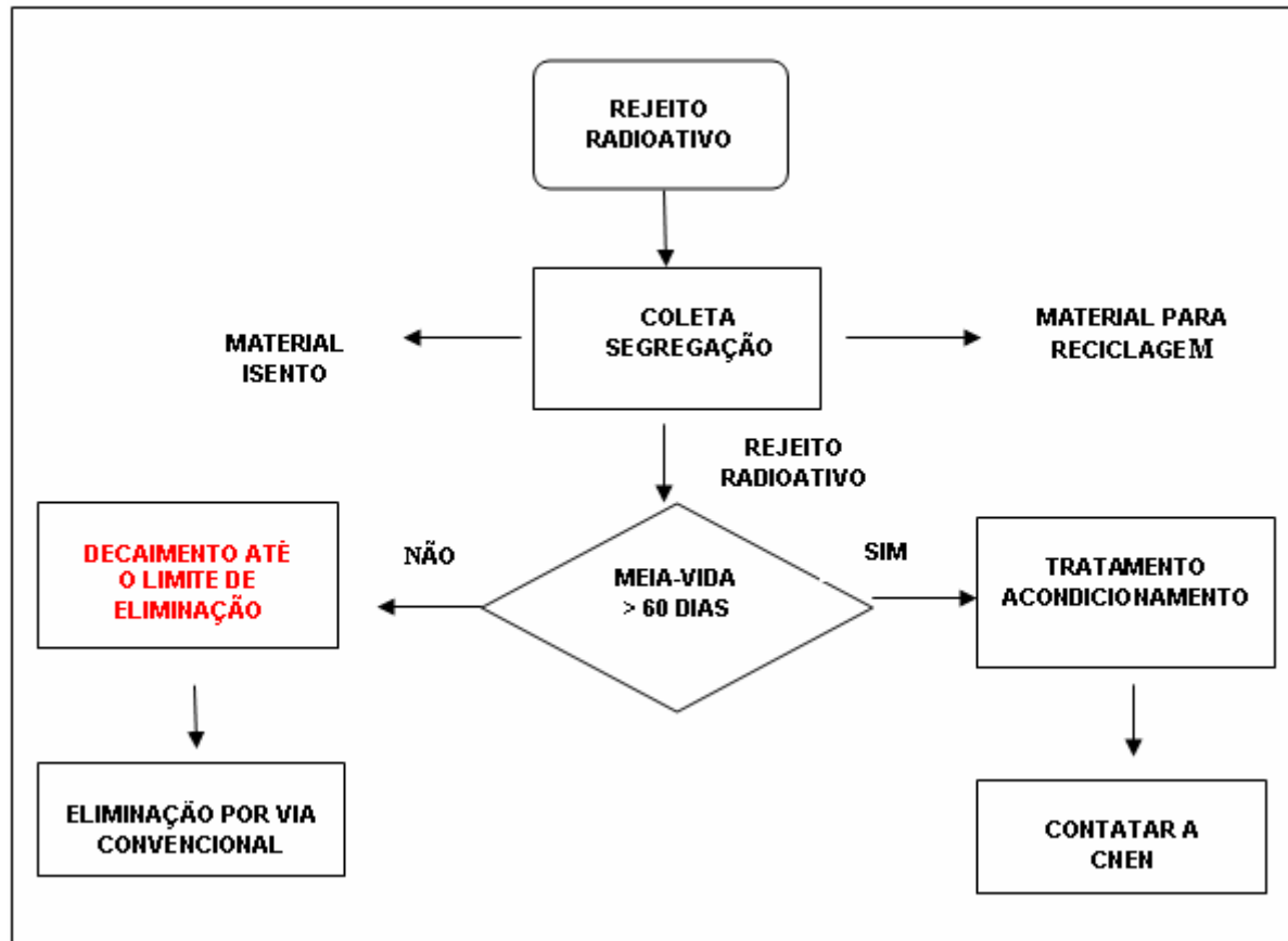
Figura 10. Fluxograma Básico de Gerência de Rejeitos Radioativos (CUSSIOL, 1999).
