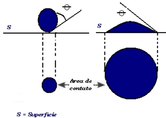
FIGURA 14 - Efeito da adição de surfactante na diminuição da tensão superficial
