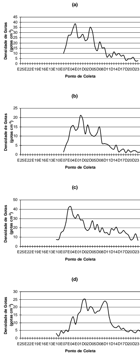
FIGURA 21 – Faixa de deposição total dos adjuvantes Fulltec® (a), Emultec plus® (b), Antideriva® (c) e da água como testemunha (d).
