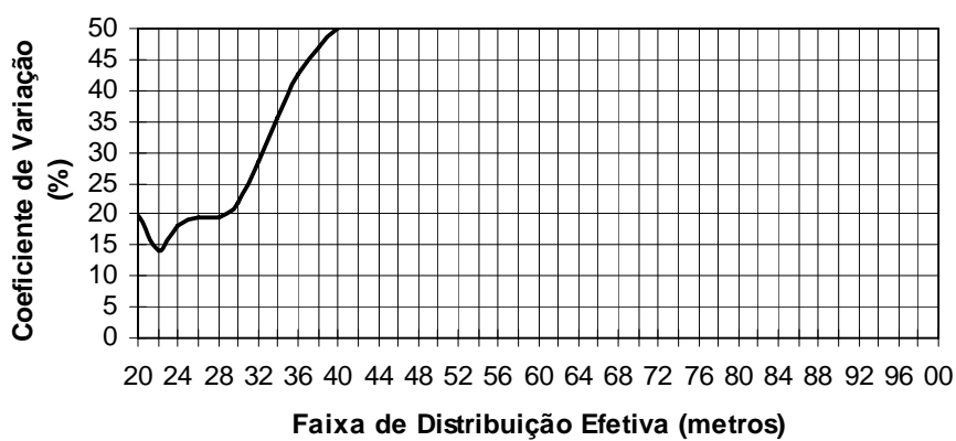
FIGURA 23 - Uniformidade de distribuição das diversas faixas efetivas da aplicação com o adjuvante Fulltec®, em vôos no mesmo sentido e em sentidos alternados.
