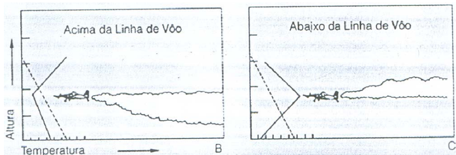
FIGURA 2 - Ponto de inversão térmica Fonte: Ozeki & Kunz, [198-].
