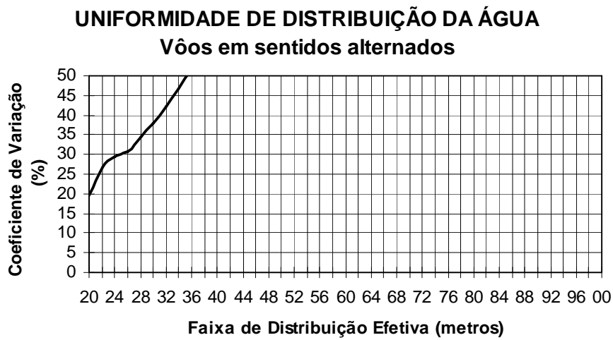
FIGURA 22 – Uniformidade de distribuição das diversas faixas efetivas da aplicação com água, em vôos no mesmo sentido e em sentidos alternados.
