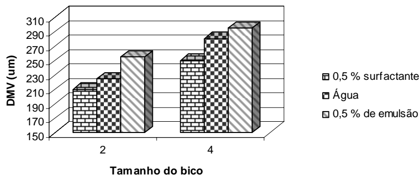
FIGURA 10 - Diâmetro mediano volumétrico produzido por dois bicos jato plano (leque), em função do tipo de líquido utilizado Fonte: Adaptado de Butler Ellis (2004), citado por Contiero, 2005).
