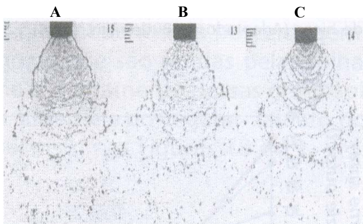
FIGURA 9 - Pulverização formada pelo bico jato plano com indução de ar: (A) calda com água + 0,5% de surfactante; (B) calda somente com água e (C) calda com água + formulação concentrado emulsionável
