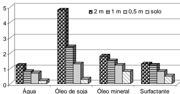
FIGURA 13 - Concentração média de clorpirifós ( \mu\text{g} clorpirifós.g material -1 ) nas folhas de milho e na superfície do solo. Fonte: Hills e Waller, 1989.
