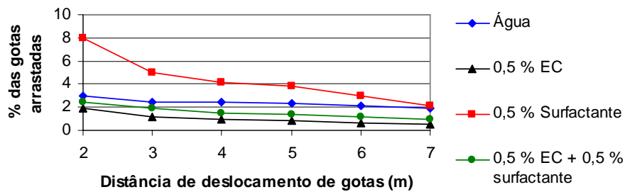
FIGURA 11 - Influência do vento, no deslocamento das gotas produzidas por um bico tipo jato plano (leque) "02" com indução de ar, em função do tipo de líquido aplicado, medido em túnel de vento (velocidade do vento de 2,0 \text{ m s}^{-1} ) Fonte: Adaptado de Butler Ellis & Bradley (2002) citados por Contiero, 2005.
