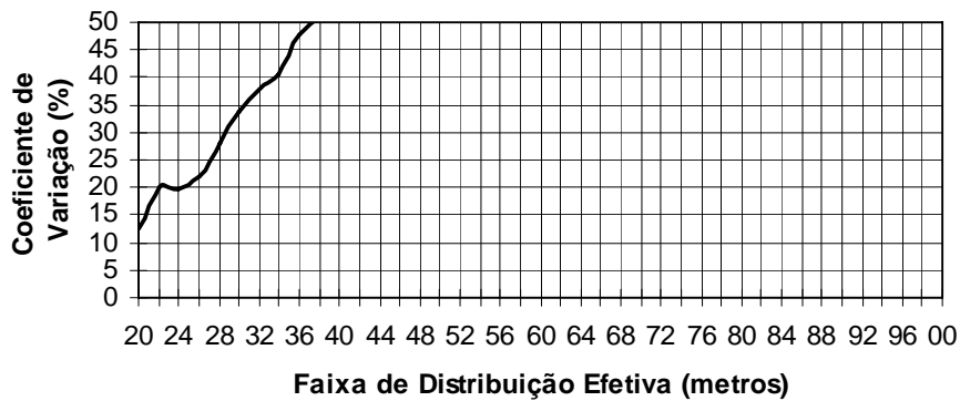
FIGURA 24 - Uniformidade de distribuição das diversas faixas efetivas da aplicação com o adjuvante Emultec plus®, em vôos no mesmo sentido e em sentidos alternados.
