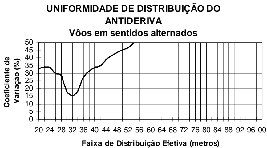
FIGURA 25 - Uniformidade de distribuição das diversas faixas efetivas da aplicação com o adjuvante Antideriva®, em vôos no mesmo sentido e em sentidos alternados.
