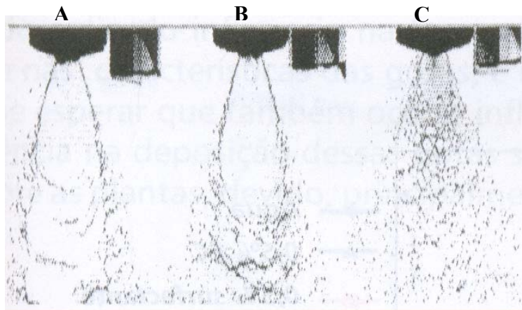
FIGURA 8 - Pulverização formada pelo bico jato plano: (A) calda com água + 0,5% de surfactante; (B) calda somente com água e (C) calda com água + formulação concentrado emulsionável
