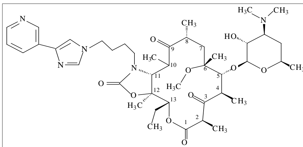
FIGURA 3.1: Estrutura química da telitromicina (GRAUL e CASTANER,1998; ZHANEL et al., 2002).
