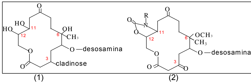
FIGURA 3.3: Diferenças entre as estruturas dos macrolídeos (1) e cetolídeos (2) (SHAIN e AMSDEN, 2002).
