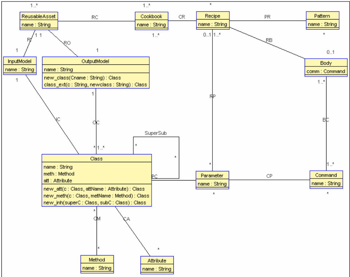
Figura 10 – Meta-modelo RDL.
