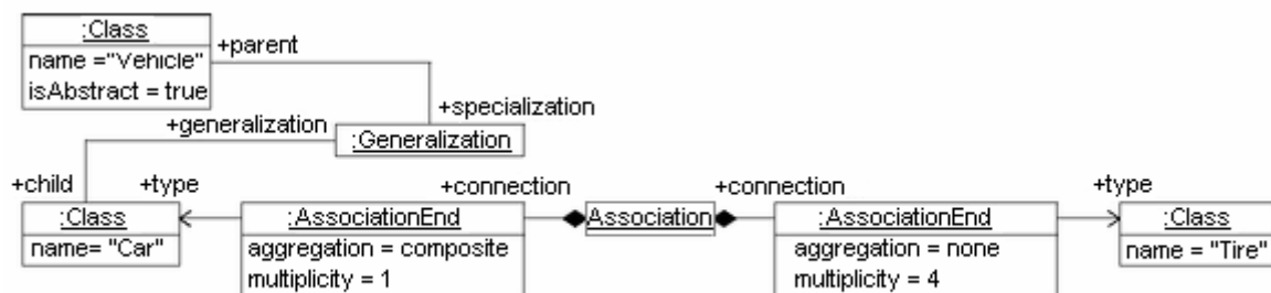
Figura 2 – Projeto baseado no modelo de semântica UML [RAS06].
