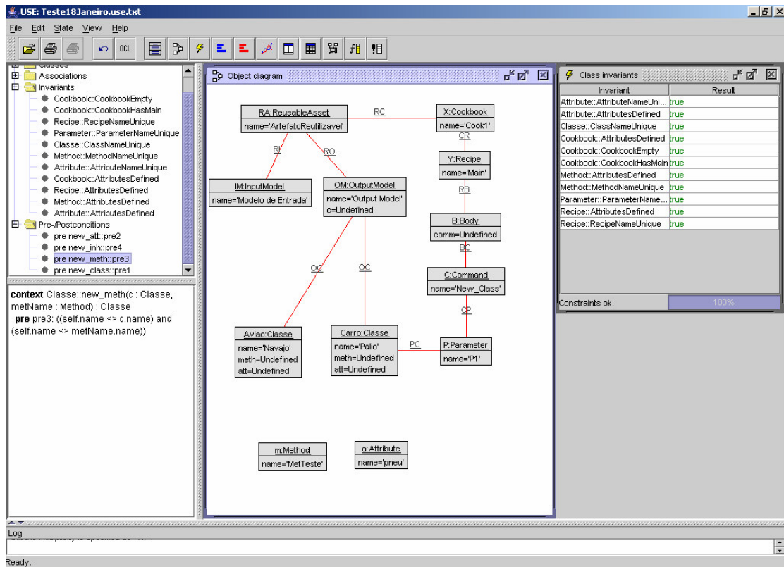
Figura 19 – Restrições OCL
