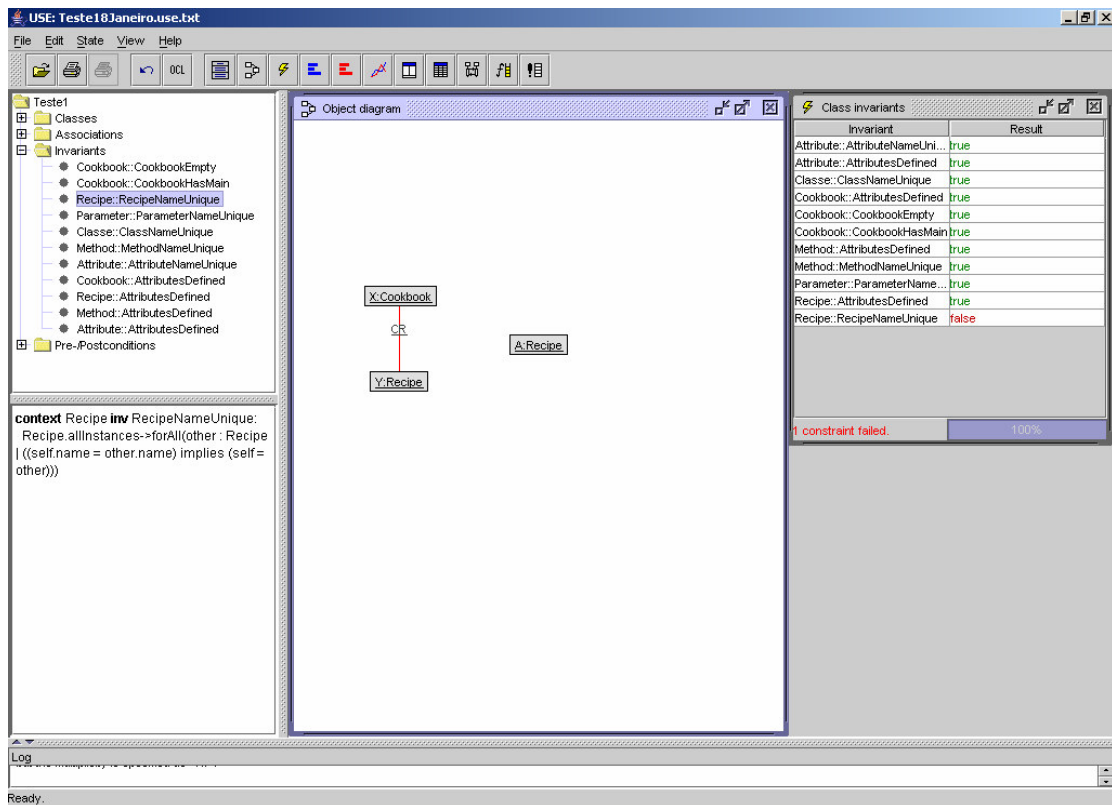
Figura 18 – Restrições OCL
