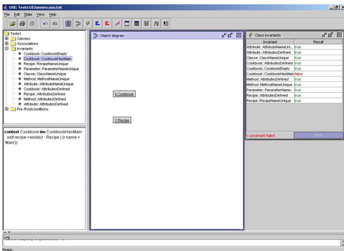
Figura 17 – Restrições OCL
