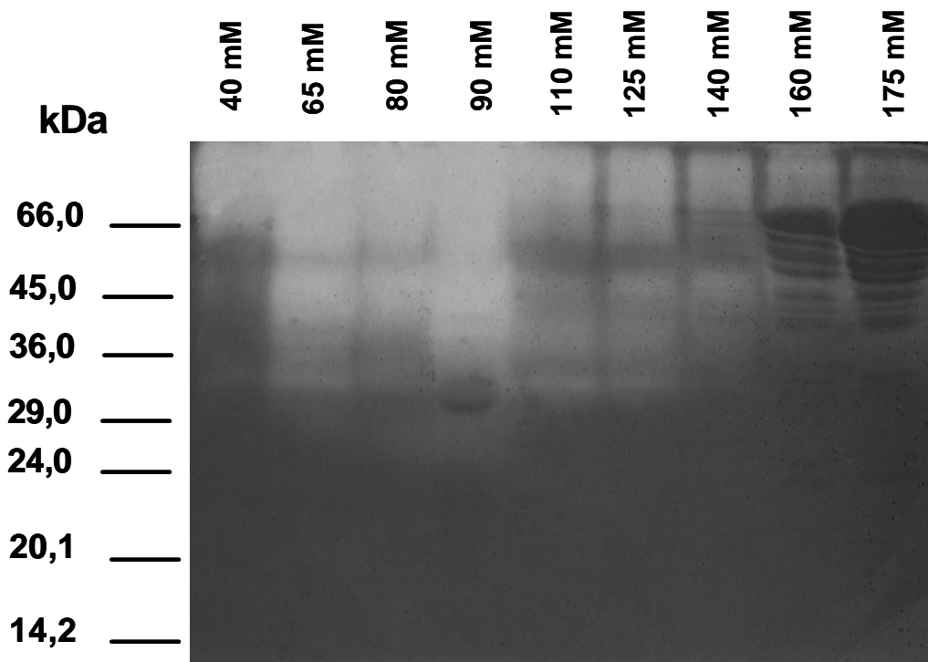
Figura 14. Enzimografia das frações com atividade esterásica eluídas da coluna de troca iônica. Cerca de 30 \mu g de proteínas de cada fração da coluna de DEAE-Sepharose (40 mM – 175 mM) foram resolvidas em gelatina-SDS-PAGE. Após a eletroforese os géis foram incubados (16 h) com tampão de ativação de serino-proteinase (10 mM fosfato de sódio pH 7,5) e em seguida, as proteases foram reveladas por coloração negativa. As faixas de gelatinólises foram detectadas por coloração negativa. Marcadores de massa moleculares estão indicados (kDa). Estes resultados são representativos de três ensaios independentes.
