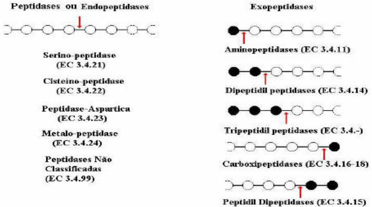
Figura 3. Classificação das enzimas peptidases, divididas em endopeptidases e exopeptidases . Figura extraída e modificada de (BARRETT, 1998).
