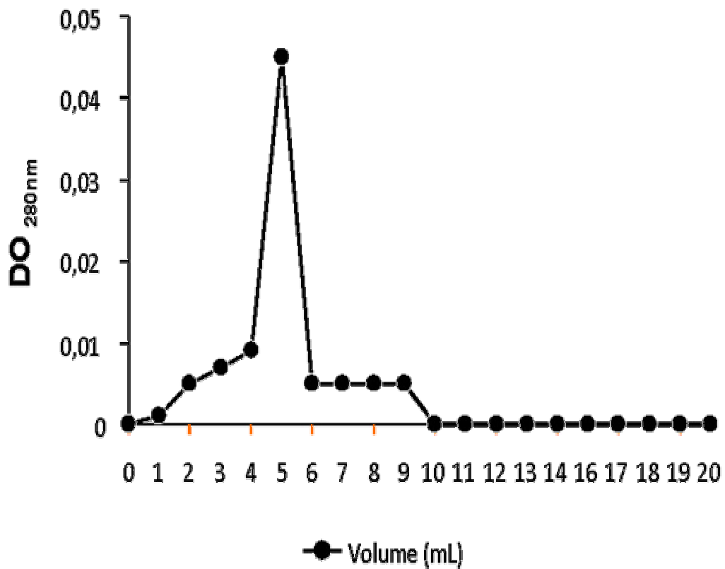
Figura 15. Cromatografia em Coluna de Aprotinina-agarose das proteínas com atividade esterásica de L3 eluídas da coluna de troca iônica. As frações da coluna de DEAE-Sephacell (40 mM – 175 mM) foram reunidas, concentradas e posteriormente na coluna de Aprotinina-agarose. A eluição foi seguida verificando-se a absorbância de 280 nm ( • ).
