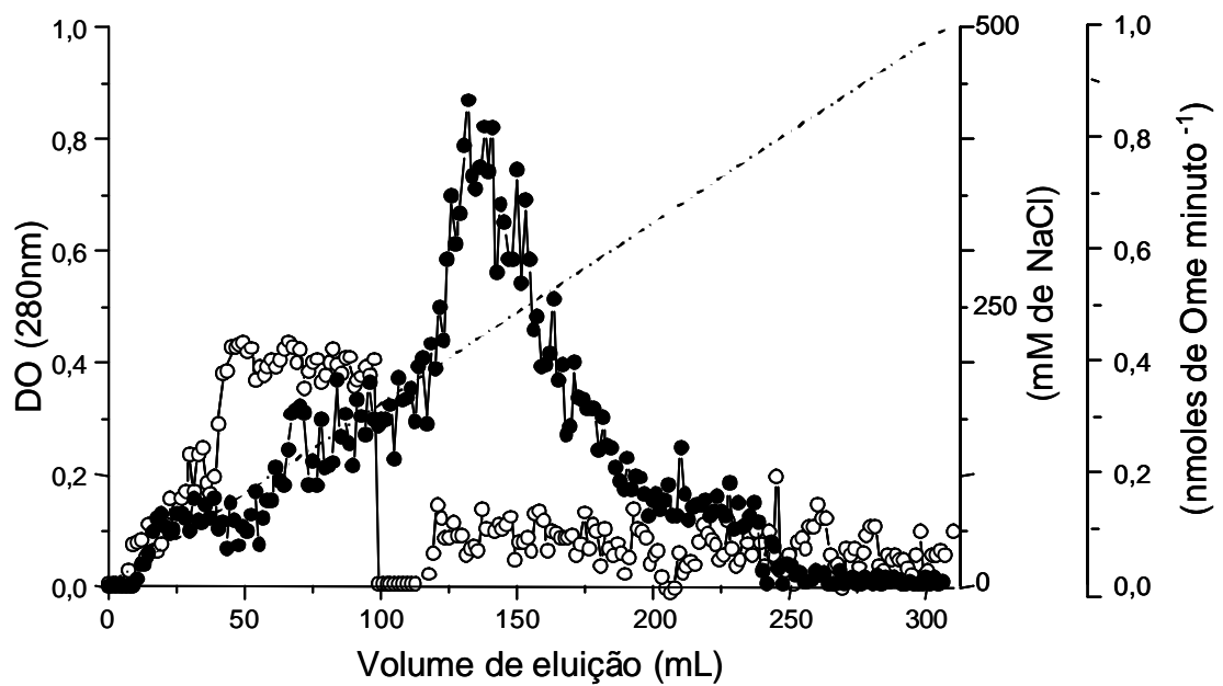
Figura 12. Fracionamento por cromatografia em DEAE-Sephacell das proteínas de L3 de Dermatobia hominis . As proteínas foram eluídas em um fluxo de 0,5 ml/min usando um gradiente linear de NaCl (0-500mM) em tampão 20mM de Tris-HCL (pH 7,2). A eluição das frações (1 ml) foi seguida verificando a absorvância a 280nm (?) e a atividade enzimática (nmols de Ome minuto -1 ) determinada com TAME a 247 nm (?).
