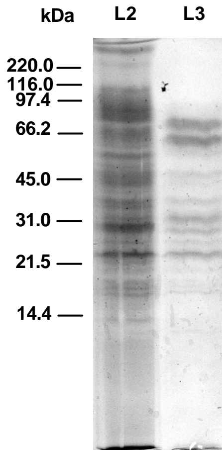
Figura 10. Perfil de proteínas das larvas de Dermatobia hominis . Extratos das larvas L2 e L3 (30 \mu g) foram resolvidos em ensaios de eletroforese em condições desnaturantes (SDS-PAGE a 12%), sendo os géis corados por prata. Marcadores de massa moleculares são indicados (kDa). Estes resultados são representativos de dois ensaios independentes.
