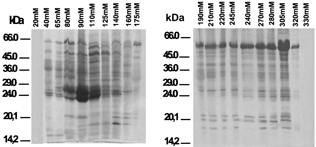
Figura 13. Eletroforese desnaturante em gel de poliacrilamida das frações de L3 eluídas da coluna de troca iônica. Cerca de 30 \mu\text{g} de proteínas de cada fração da coluna de DEAE-Sephacell (20 mM – 330mM) foram resolvidas em SDS-PAGE (12%). Após a eletroforese as proteínas foram reveladas pela técnica de impregnação pela prata. Os números indicados a esquerda representam os valores dos marcadores de massa molecular (kDa).
