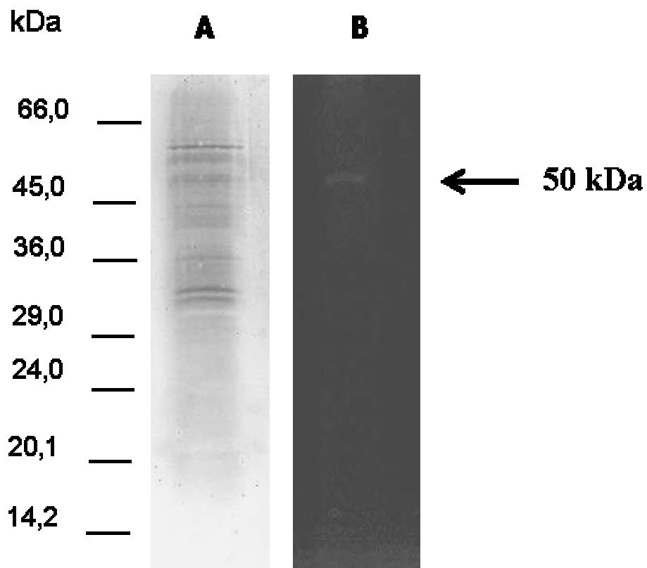
Figura 16. Análises por eletroforese das proteínas de L3 eluídas da coluna de Aprotinina-agarose. Cerca de 20µg da fração foi resolvida em SDS-PAGE (A) e gelatina- SDS-PAGE (B) e reveladas pela prata e por coloração negativa, respectivamente. Seta indica uma serino-proteinase de 50 kDa. Marcadores de massa moleculares estão indicados (kDa). Estes resultados são representativos de dois ensaios independentes.
