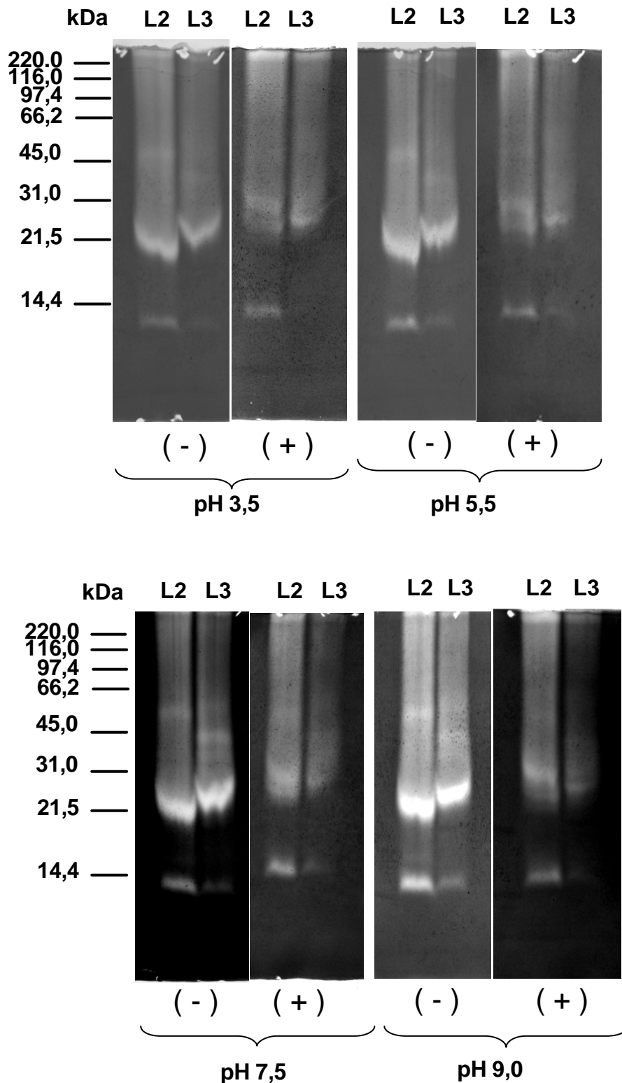
Figura 11. Atividade de Proteases larvares de Dermatobia hominis em gelatina-SDS-PAGE. Depois da eletroforese dos extratos larvares L2 e L3, (20 \mu g) os géis foram incubados com 10mM de tampão acetato de sódio (pH 3,5 e 5,5) ou 10 mM de tampão fosfato (pH 7,5 e 9,0) na ausência (-) ou presença (+) de 10 mM de PMSF. As faixas de gelatinólises foram detectadas por coloração negativa. Marcadores de massa molecular estão indicados (kDa). Estes resultados são representativos de três ensaios independentes.
