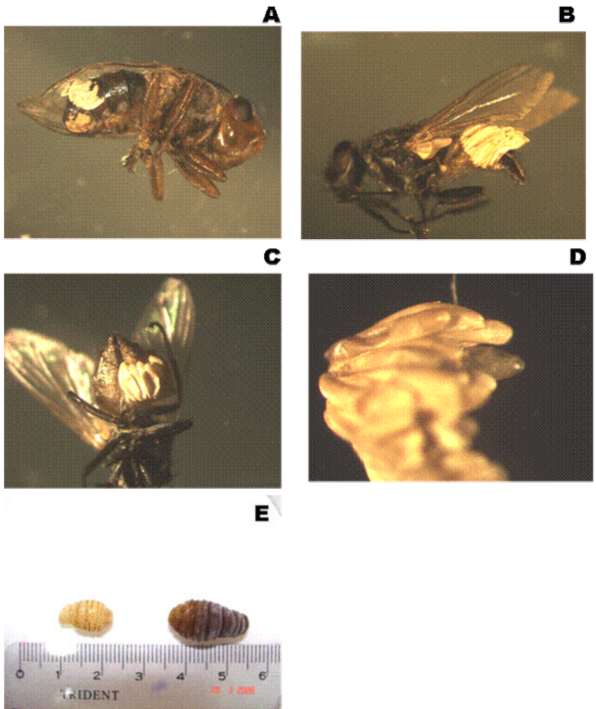
Figura 2. Formas adultas, larvares e foréticos de Dermatobia hominis . (A) Adulto de D.hominis com oviposição no abdômen, (B) Musca domestica com postura de D. hominis no abdômen, (C) Postura de D. hominis semelhante a “penca de banana”, (D) Larva de 1. o estágio saindo do opérculo, e (E) Larvas de D. hominis melanizada a direita (L3) e não melanizada a esquerda (L2).
