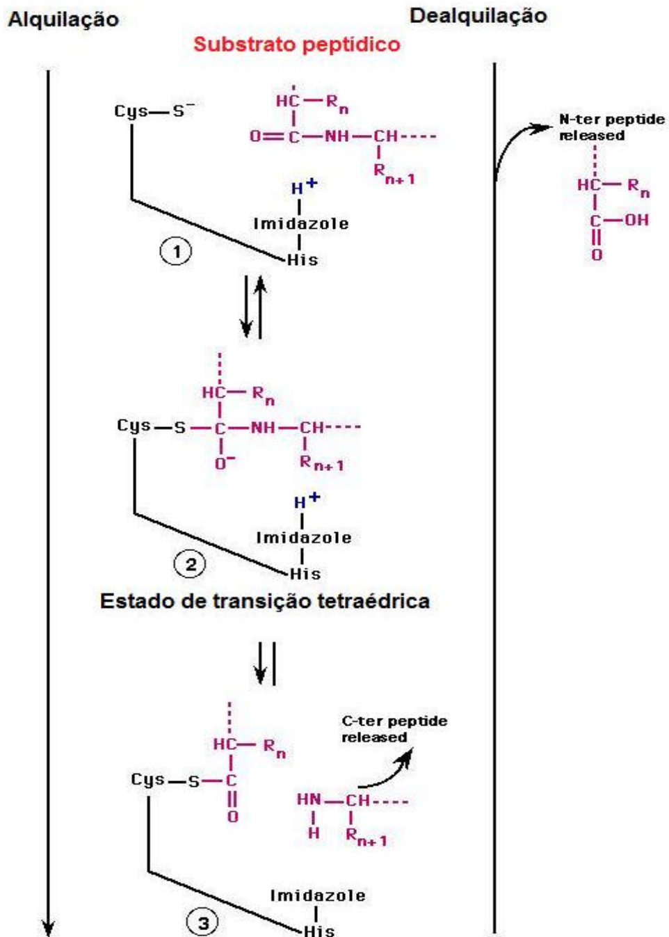
Figura 7. Mecanismo catalítico das cisteíno-proteínases, adaptado de ( http://delphi.phys.univ-tours.fr/Prolysis/introprotease.html ).
