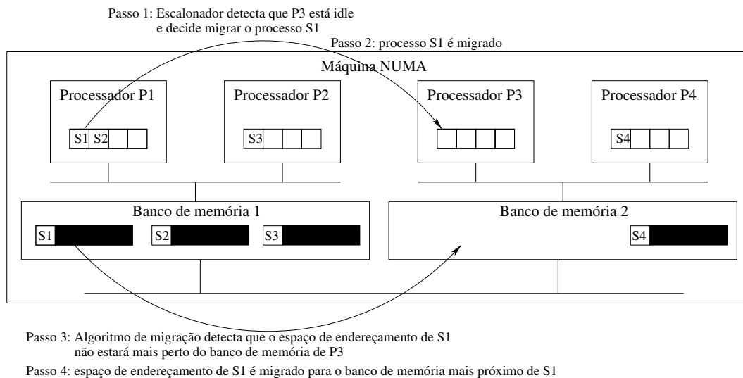
Figura 2.2: Migração do espaço de endereçamento de um processo
