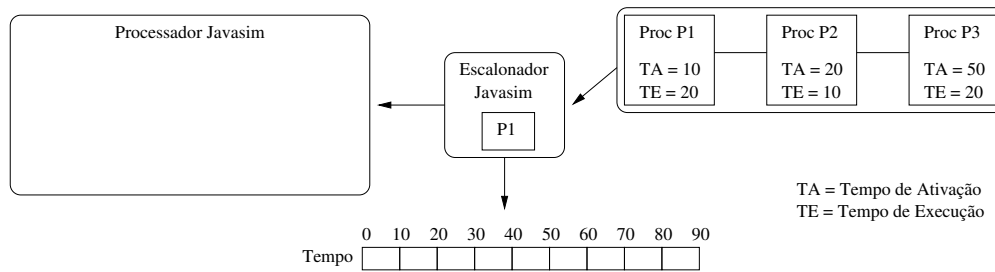
Figura 3.1: Funcionamento do Javsim - Parte 1 (Estrutura das tarefas)
