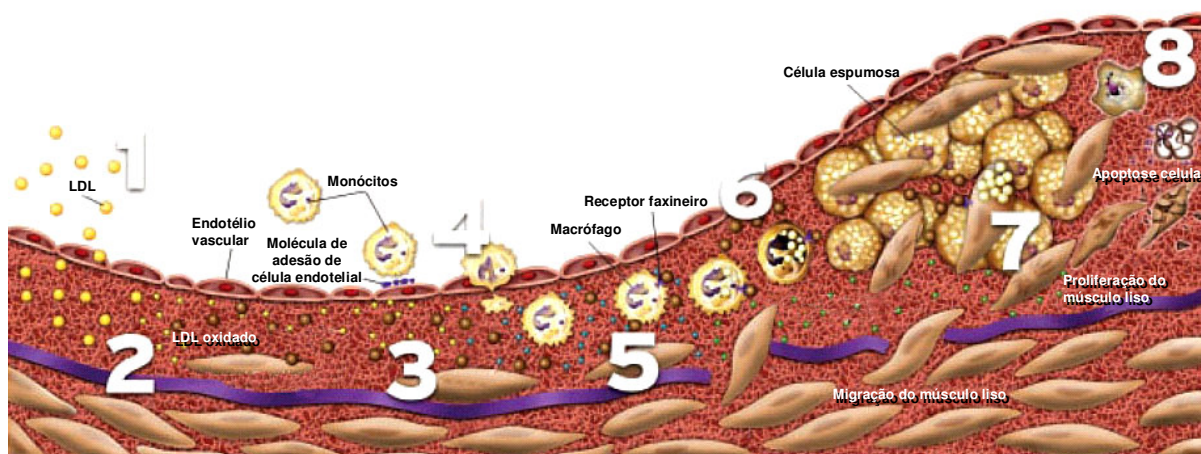
Figura 5 - Estágios do desenvolvimento de uma placa aterosclerótica.
