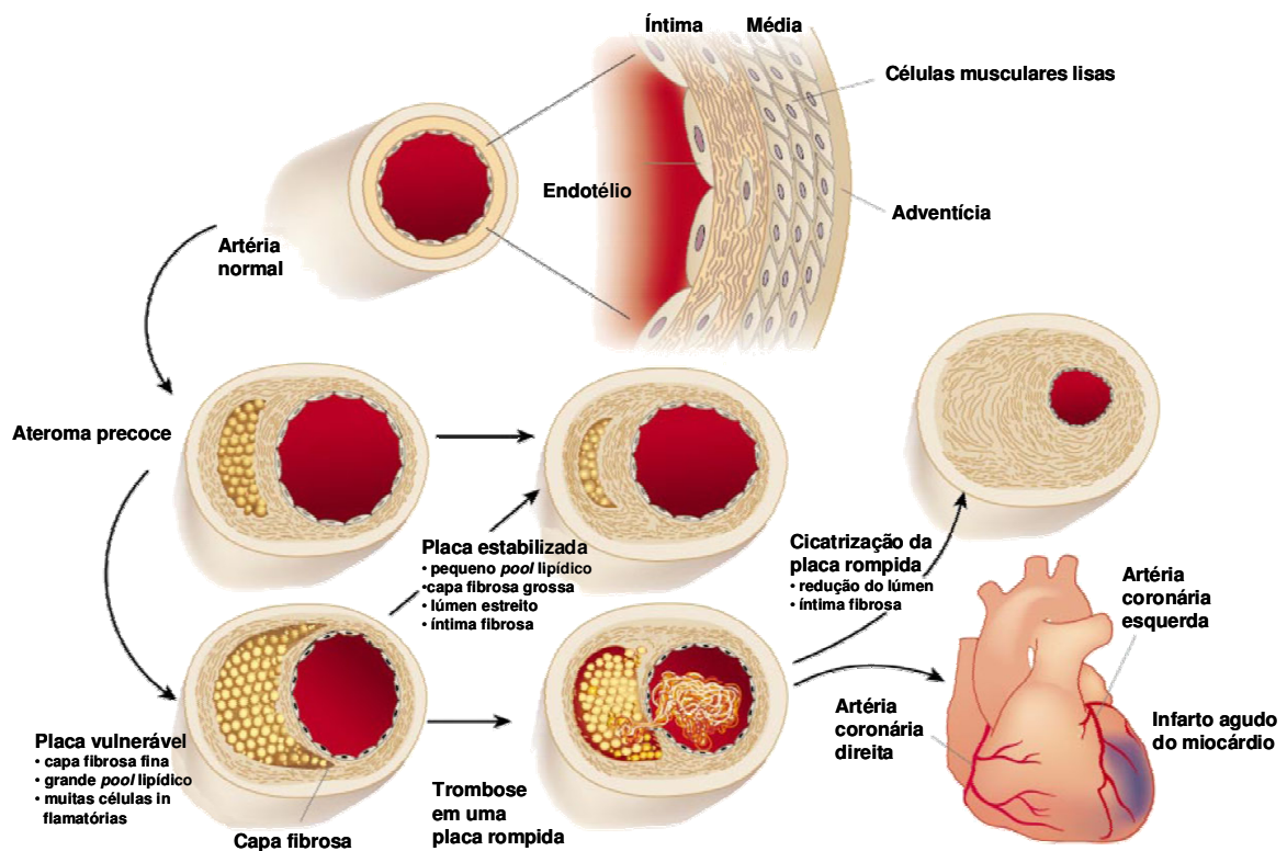
Figura 6 - Esquema da evolução de um ateroma. Adaptado de Libby, 2002.
