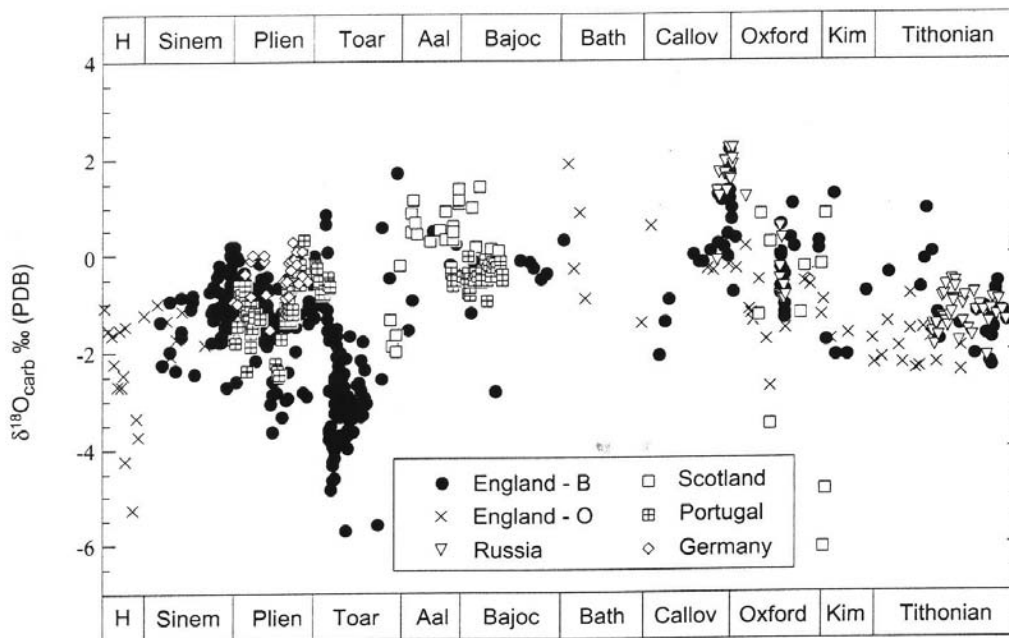
Figura 56 – Curva de \delta^{18}O para o Jurássico (Jenkyns, et al. 2002).
