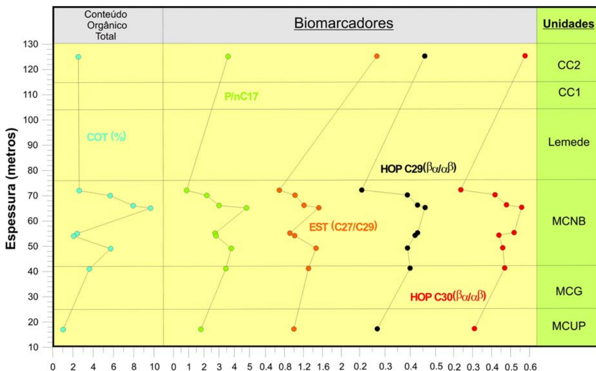
Figura 20 – Curvas de distribuição dos biomarcadores P/nC17, EST(C27/C29), HOP C29 e HOP C30 e suas correlações com o COT.
