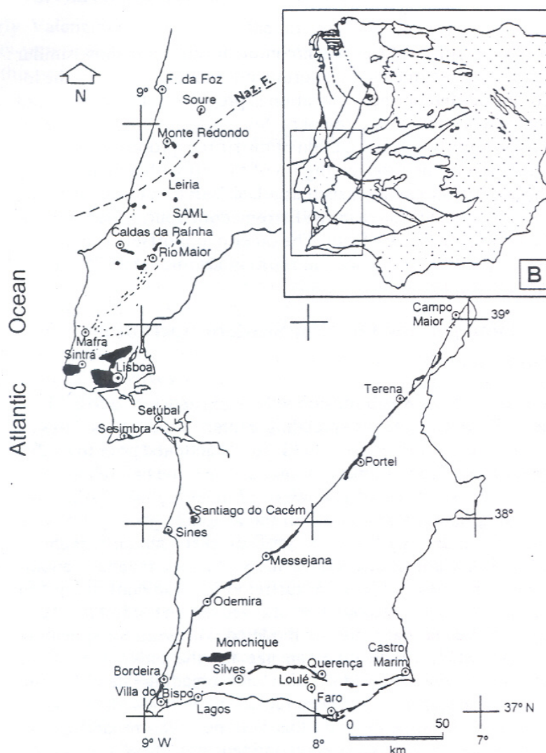
Figura 16 – Áreas de ocorrência das rochas ígneas mesozóicas na Bacia Lusitânica. SAML= Lineamento Serra D’aire – Montejuízo ; Naz. F= Falha de Nazaré (Pinheiro, et al. 1996).
