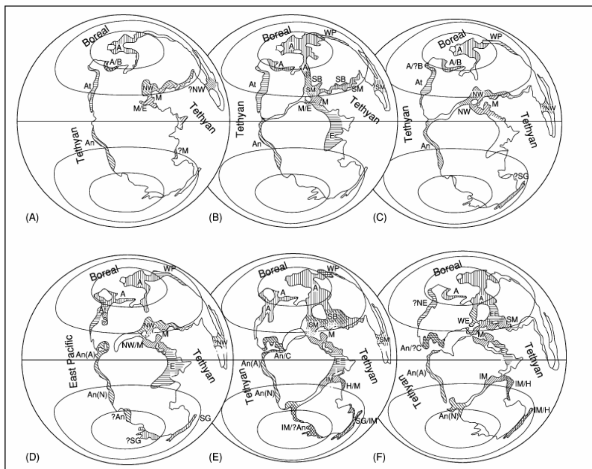
Figura 2 – A evolução dos continentes durante o Jurássico e suas províncias faunísticas. (A) Hetangiano-Eopliesnbaquiano; (B) Neopliesnbaquiano-Toarciiano; (C) Aaleniano-Eobajociano; (D) Neobajociano-parte inicial do Eocaloviano; (E) parte final do Eocaloviano-Kimmeridgiano; (F) Titoniano-Valanginiano. As províncias de amonites são: Região do Tétis - M, Mediterrâneo; NW, Noroeste da Europa; SM, Submediterrâneo; H, Himalaia; E, Etiópia; IM, Indo-Malgach; SG, Sula-Nova Guiné; C, Cuba; WP, Pacífico Oeste. Região do Pacífico Leste (Neobajociano – Batoniano) ou Tétis – At, Athabasca; Na, Andes. Região Boreal –A, Ártico; SB, Sub-Boreal; WE, Europa Oeste; EE, Europa Leste; B, Bering (Page, 2004).
