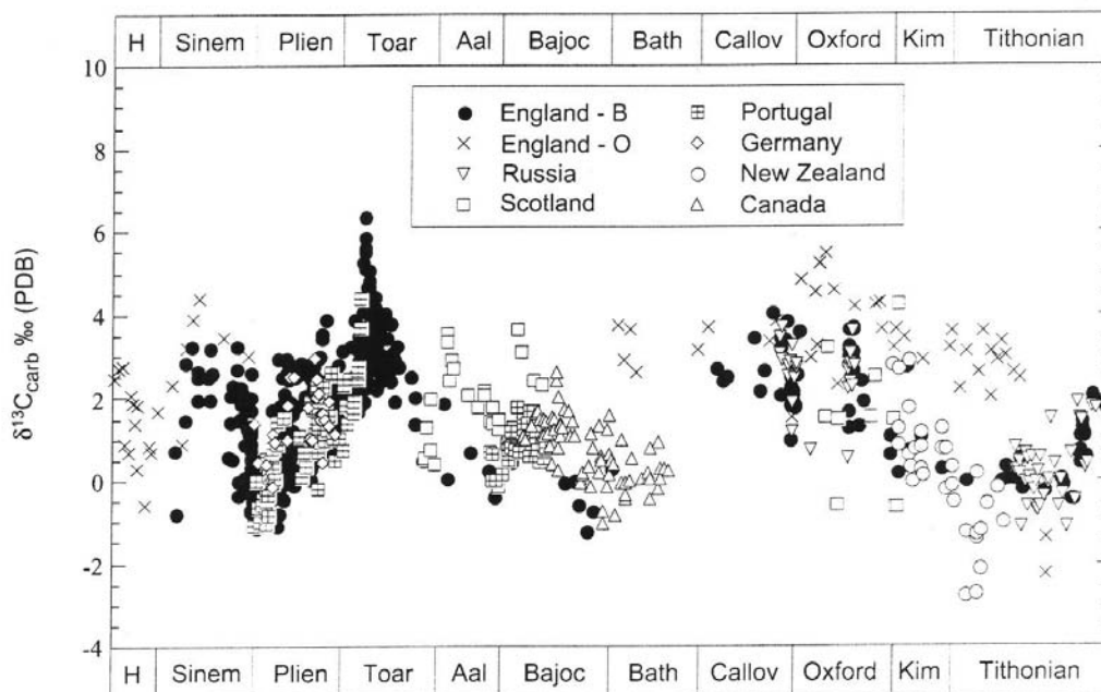
Figura 55 – Curva de \delta^{13}C para o Jurássico (Jenkyns, et al. 2002).
