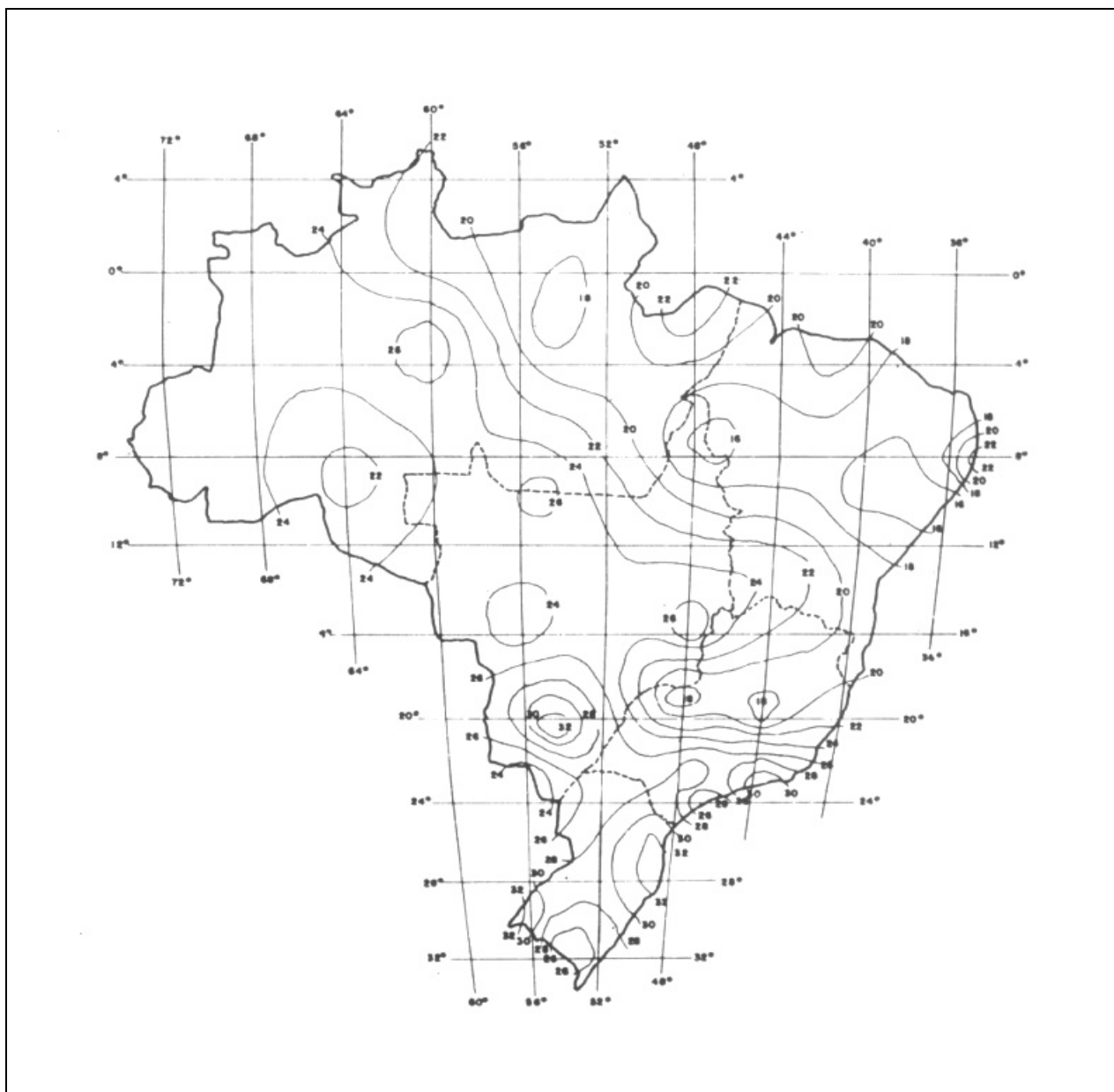
Figura A.6 – Velocidade Básica do Vento (m/s)
