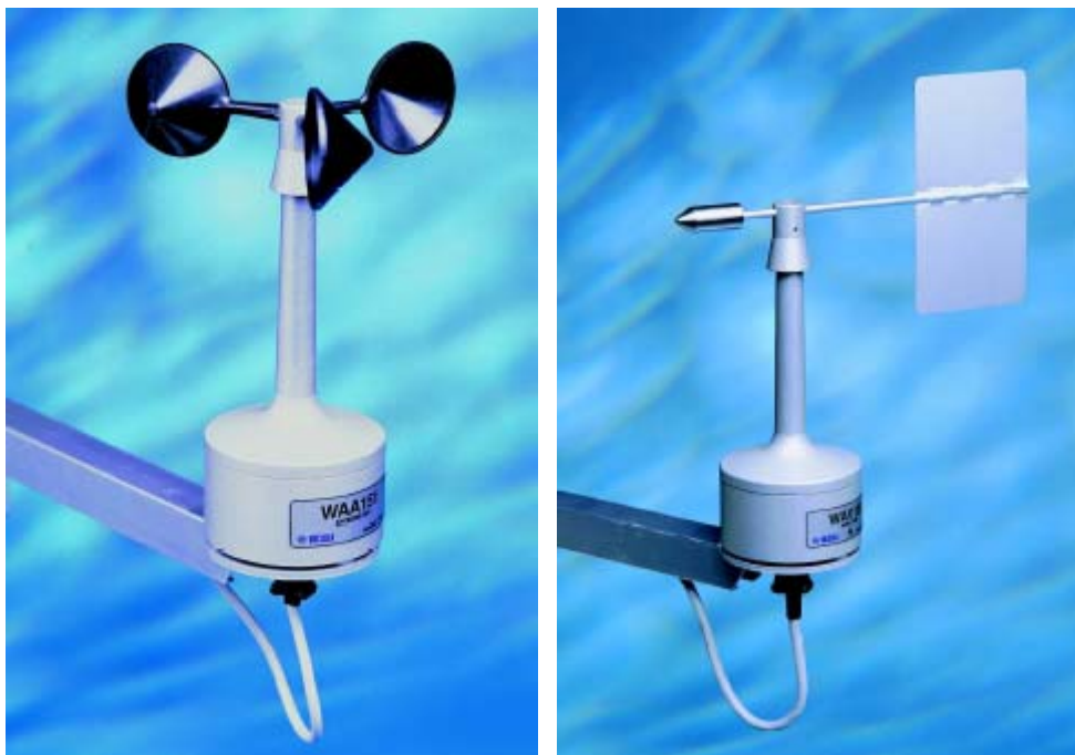
Figura 3.3 - Anemômetro tipo Concha e Leme Fonte: (HOBECO, 2005)
