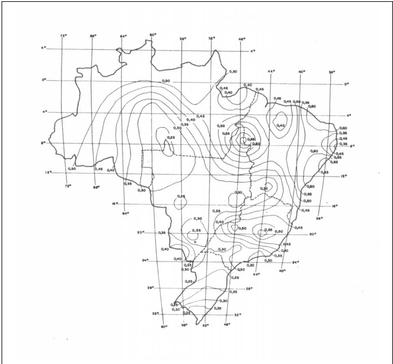
Figura A.7 – Parâmetro Alfa da Distribuição Estatística de Gumbel (m/s)^{-1}
