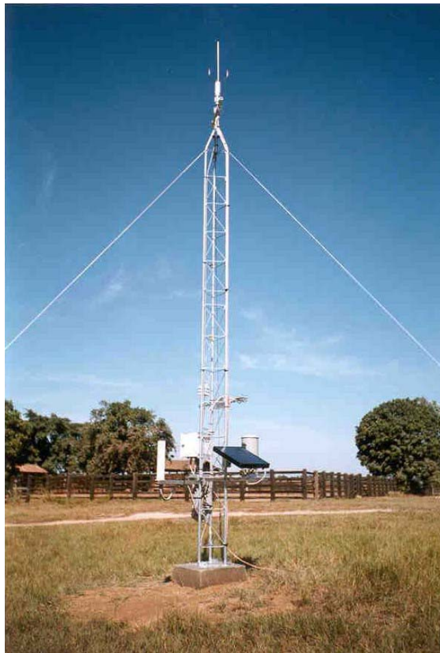
Figura 3.1 - PCD meteorológica do INPE em área rural de Goiás Fonte: (Foto realizada pelo autor, 1999)
