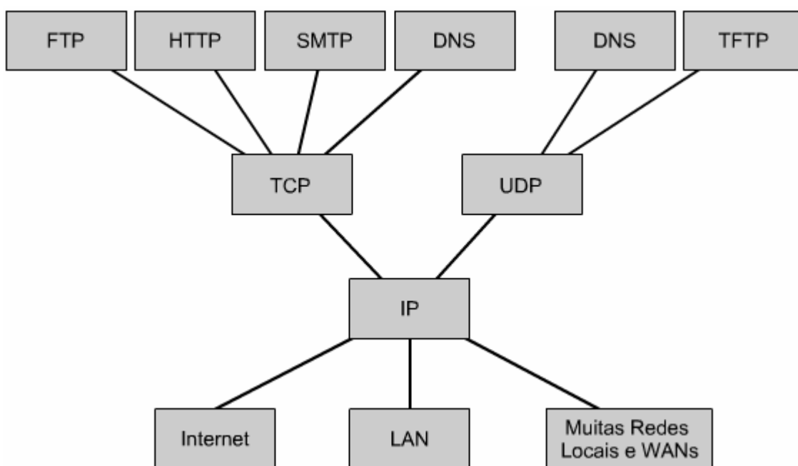
Figura 7 – Estrutura do modelo TCP/IP e seus protocolos
