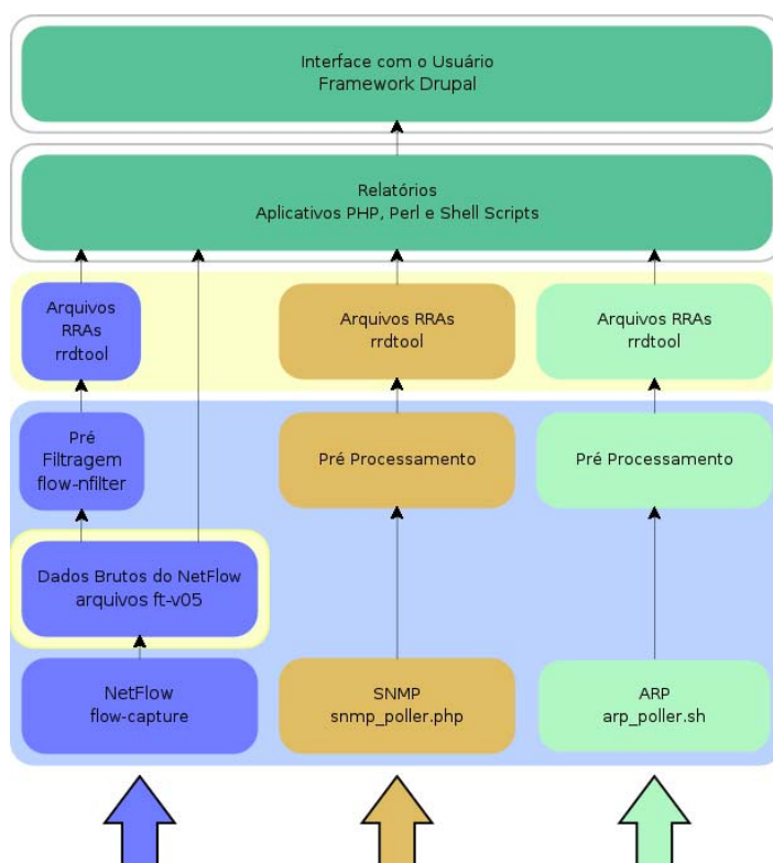
Figura 31 - Arquitetura implementada
