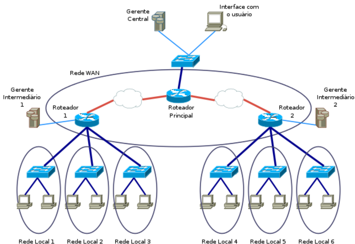
Figura 21 - Gerenciamento Distribuído
