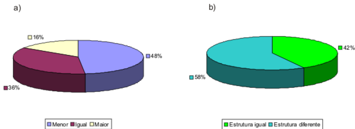
Figura 5.1: a) Gráfico percentual comparativo de tempo de execução da Nest2 em relação à Nest b) Gráfico de comparação entre estruturas geradas pela Nest2 e Nest
