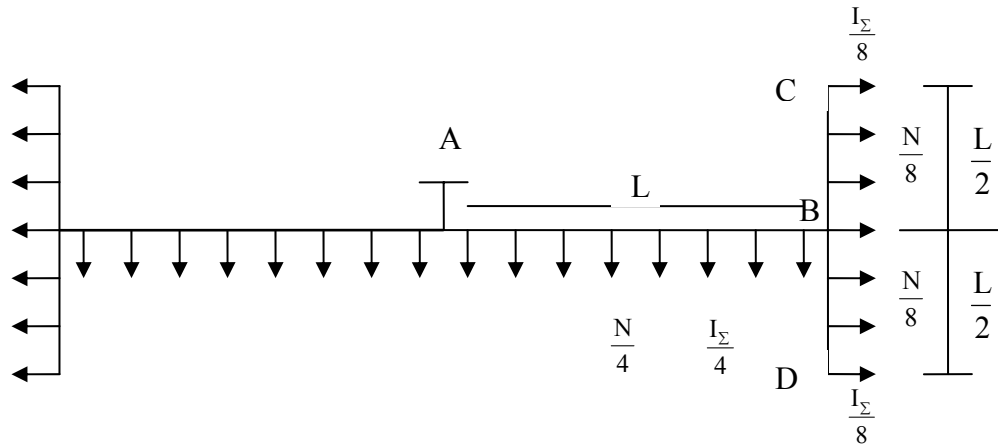
Figura 3.17 – Modelo 7 – Esquemático
