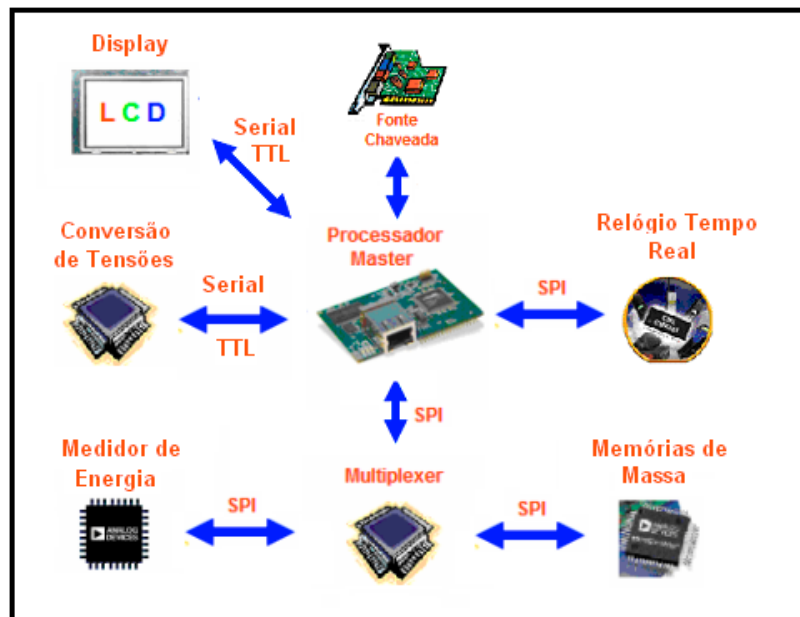
Figura 12. Diagrama interno do sistema microprocessado (SM).
