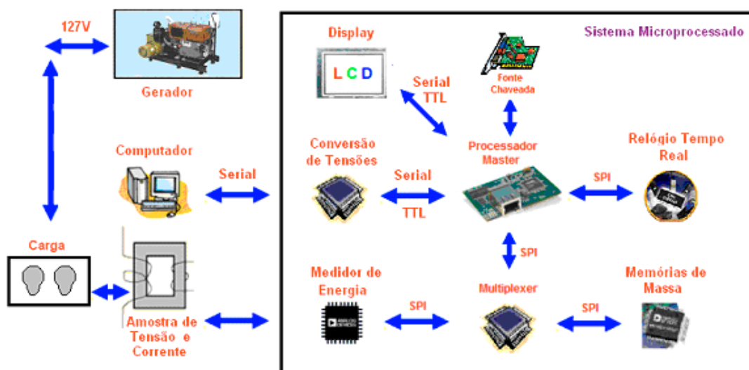
Figura 13. Diagrama interno do SM e respectivas conexões com PGEE e PCE.
