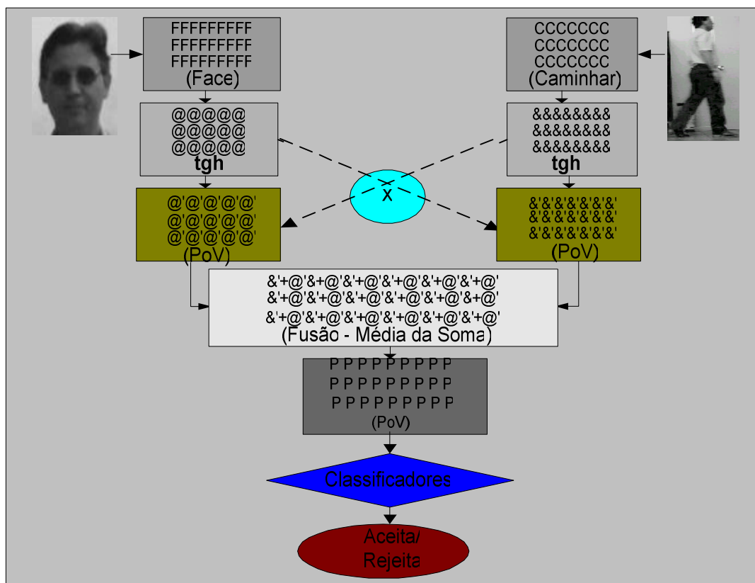
Figura 33 – Arquitetura com o esquema de fusão no nível de características
