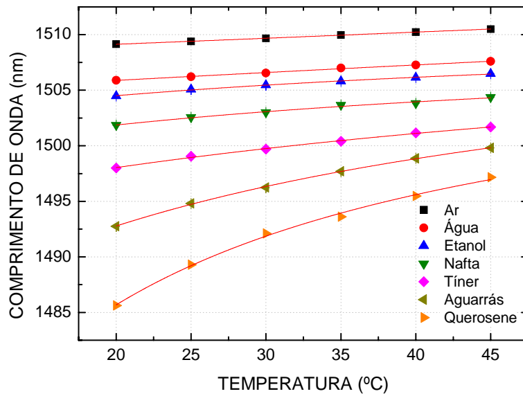
Figura 46 – Resposta do vale 3 da CLPG SE01 à variação de temperatura quando a rede está imersa nas diferentes amostras. As curvas representam o ajuste empírico, equação 30.
