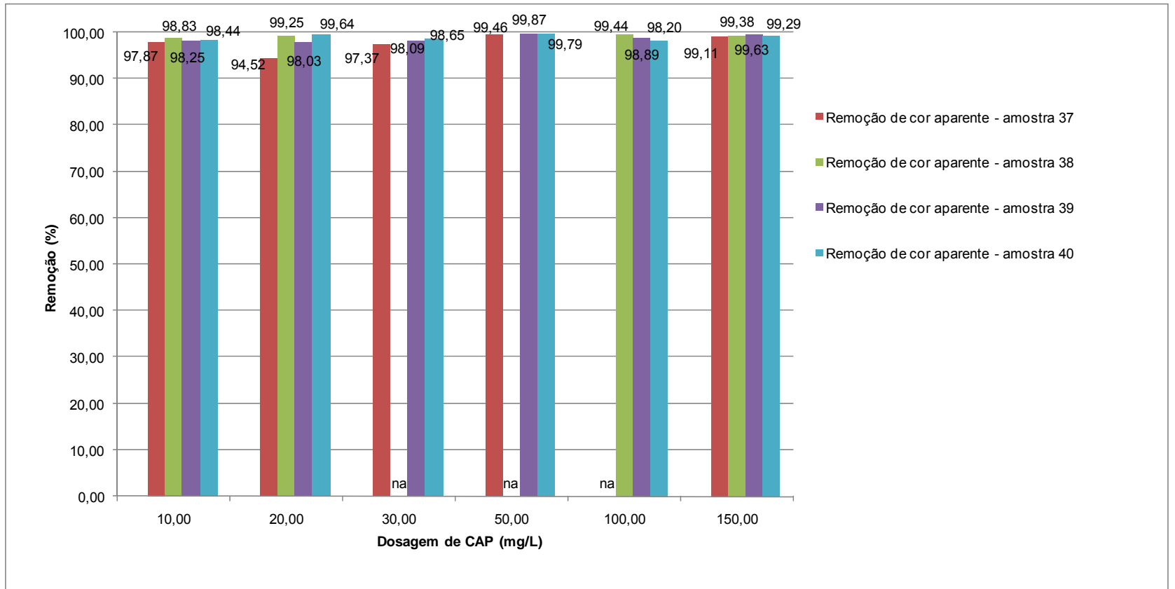
Figura 5.9 Gráfico dos valores remoção de cor aparente, em função da dosagem de CAP (mg/L)
