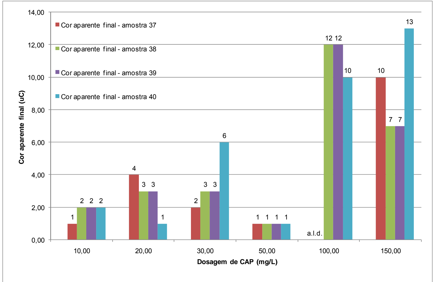
Figura 5.6 Gráfico dos valores de cor aparente “final-após filtração”, em função da dosagem de CAP (mg/L)
