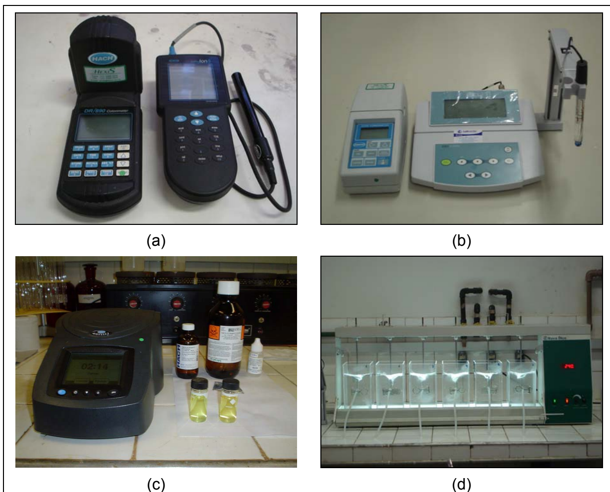
Figura 4.1 Colorímetro e condutivímetro (a); pHmêtro de bancada e turbidímetro; espectrofotômetro DR 2500 da Hach (c) e equipamento “jar-test” (d)
