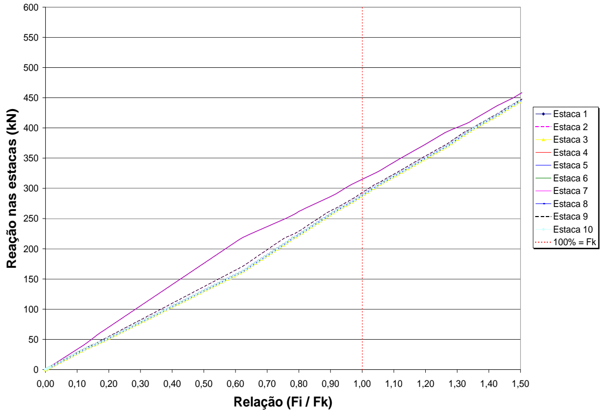
Figura 6.5: Reações nas estacas ao longo da aplicação das ações para bloco com altura de 115 cm e solo deformável
