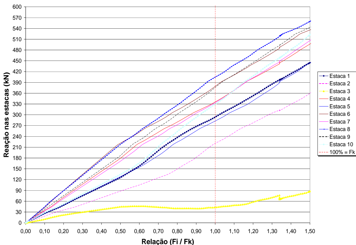
Figura 6.39: Reações nas estacas ao longo da aplicação das ações para bloco com altura de 115 cm e solo deformável
