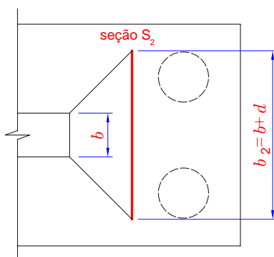
Figura 3.7: Largura da seção de referência S_2
