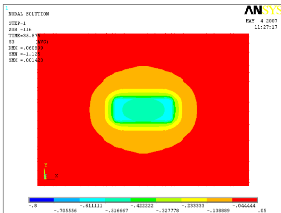
Figura 6.14: Campos de tensão de compressão - bloco com altura de 200 cm para solo deformável - valores em \text{kN}/\text{cm}^2
