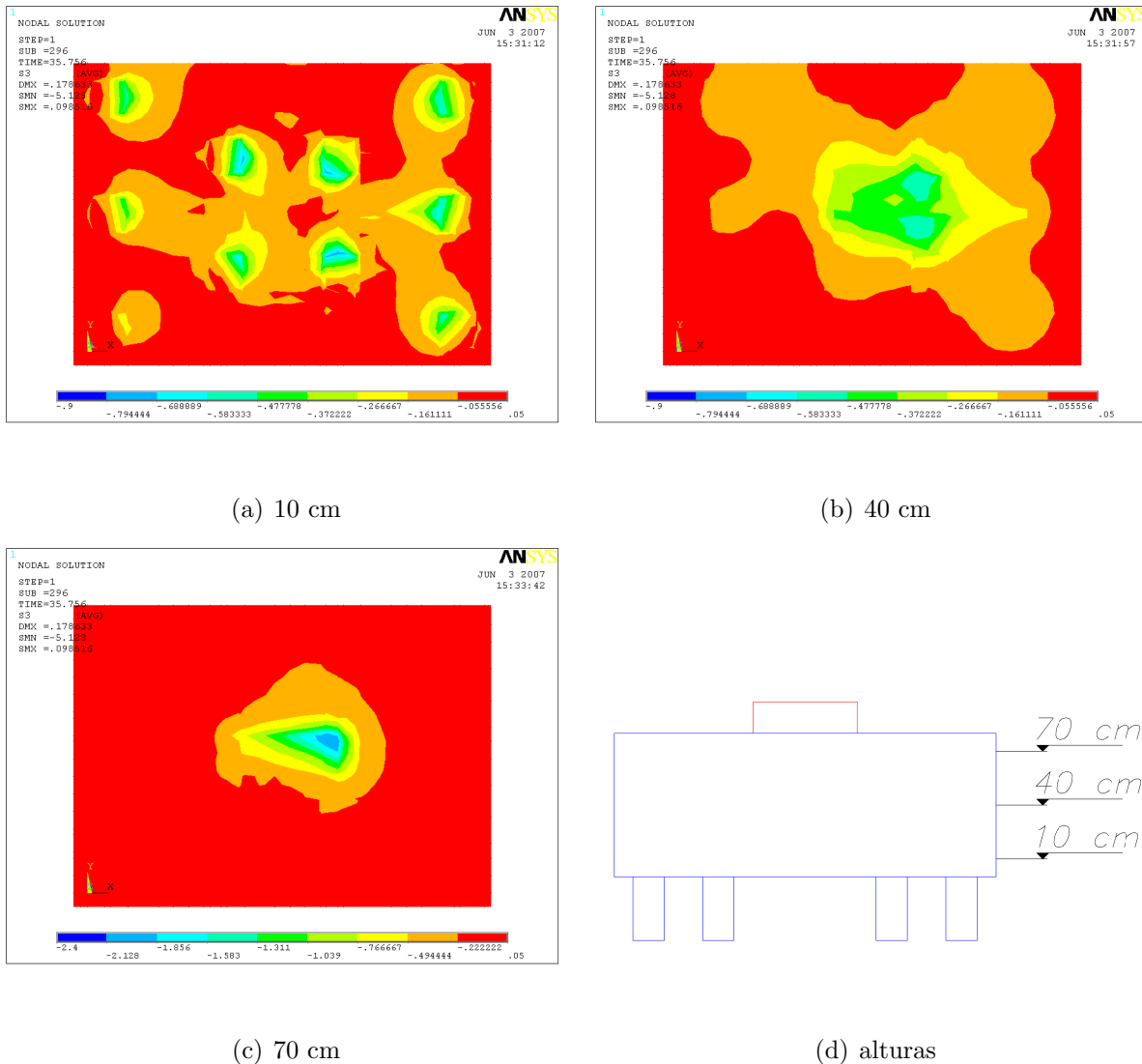
Figura 6.44: Campos de tensão de compressão - bloco com altura de 80 cm para solo deformável - valores em kN/cm 2
