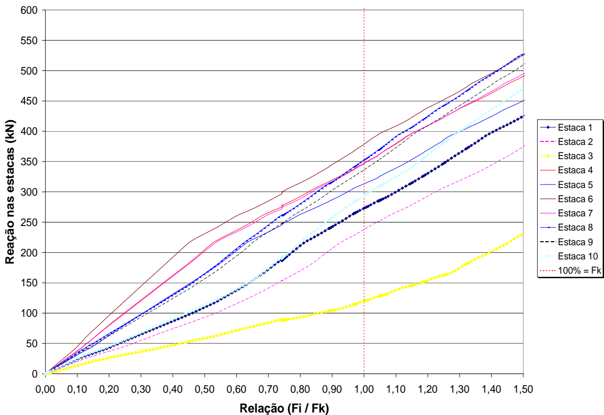
Figura 6.21: Reações nas estacas ao longo da aplicação das ações para bloco com altura de 80 cm e solo deformável
