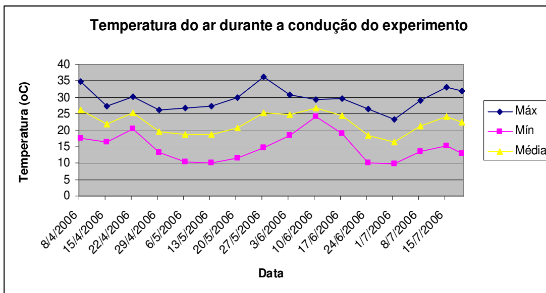
Figura 6. Variação do valor médio, a cada sete dias, da temperatura ambiente, máxima, mínima e média, em ambiente protegido com a cultura do pimentão, nos meses de abril a julho de 2006, no complexo de Controle Biológico e Cultivo Protegido Prof. Dr. Mário César Lopes – UNIOESTE – Marechal Cândido Rondon – PR, 2006.
