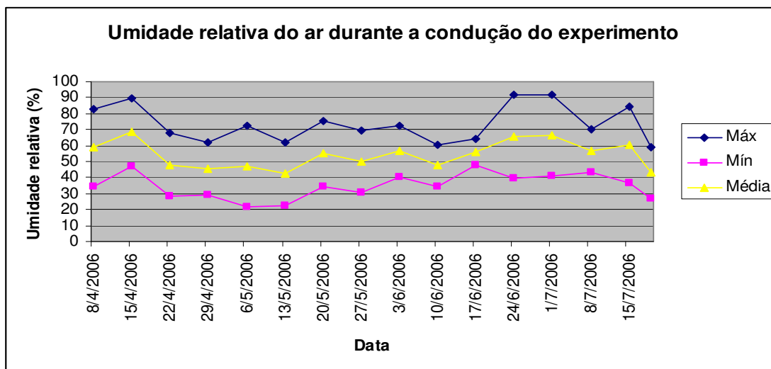
Figura 7. Variação do valor médio, a cada sete dias, da umidade relativa do ar, máxima, mínima e média, em ambiente protegido com a cultura do pimentão, nos meses de abril a julho de 2006, no complexo de Controle Biológico e Cultivo Protegido Prof. Dr. Mário César Lopes – UNIOESTE – Marechal Cândido Rondon – PR, 2006.
