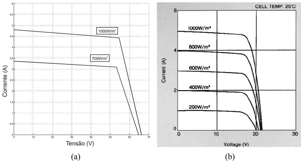
Figura 3.11 – (a) Curva característica de um painel fotovoltaico simulado no Software PSIM, (b) Curva característica do painel utilizado como referência fornecida pelo fabricante [54].
