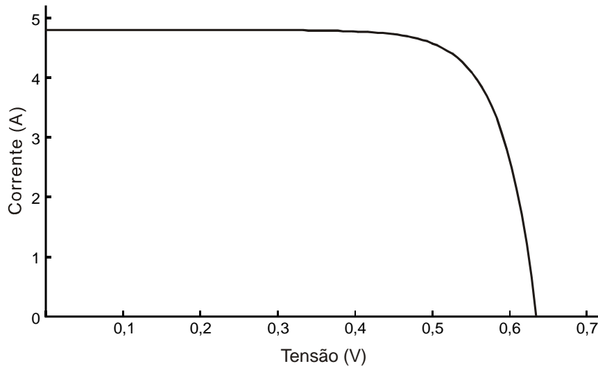
Figura 3.4 - Curva característica de uma célula fotovoltaica.
