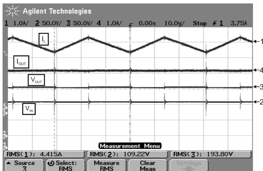
Figura 6.4 - Formas de onda da topologia centralizada sob radiação solar de 1000W/m 2 .
