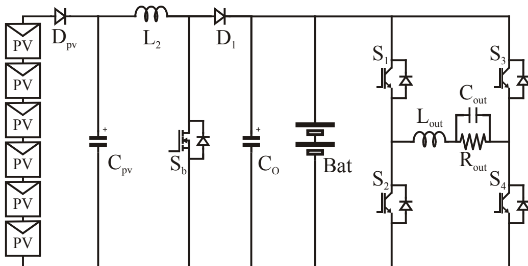
Figura 5.1 - Sistema tradicional.
