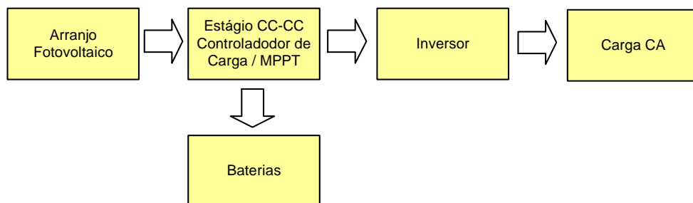
Figura 2.10. Sistema Fotovoltaico Isolado com Carga CA, Armazenamento de energia e MPPT
