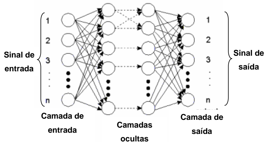
Figura 7: Grafo arquitetural de um MLP (Haykin, 1999).
