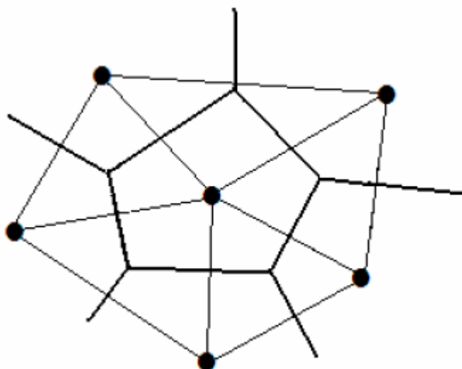
Figura 5: Mosaico de Voronoi (Roque, 2007).
