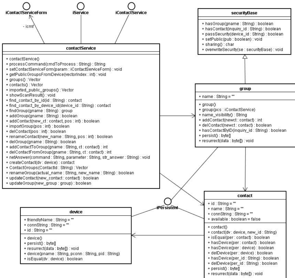
Figura 4.4: Componentes do Serviço de Contatos
