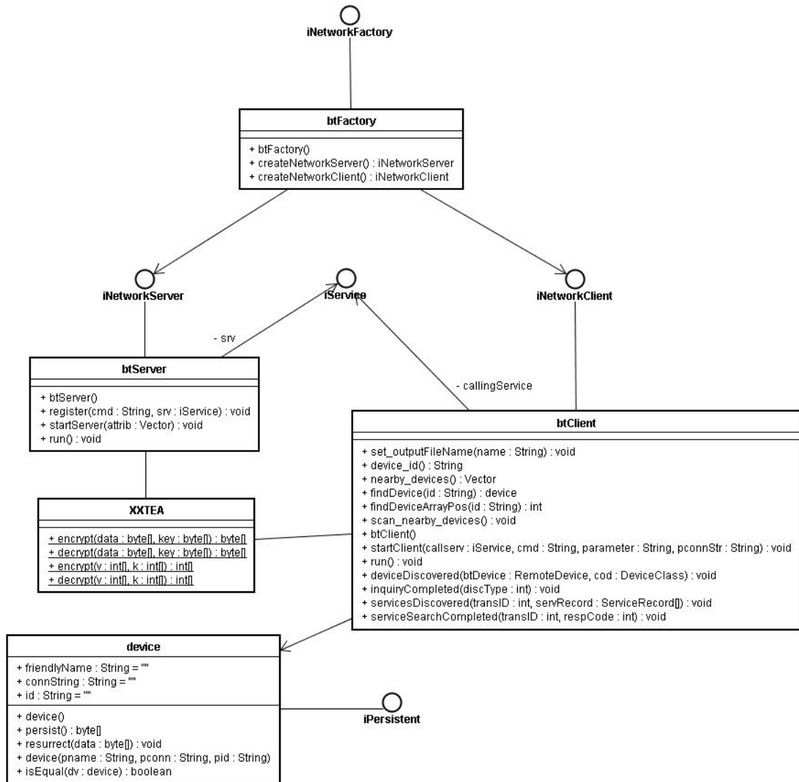
Figura 4.2: Diagrama dos componentes da Camada de Rede
