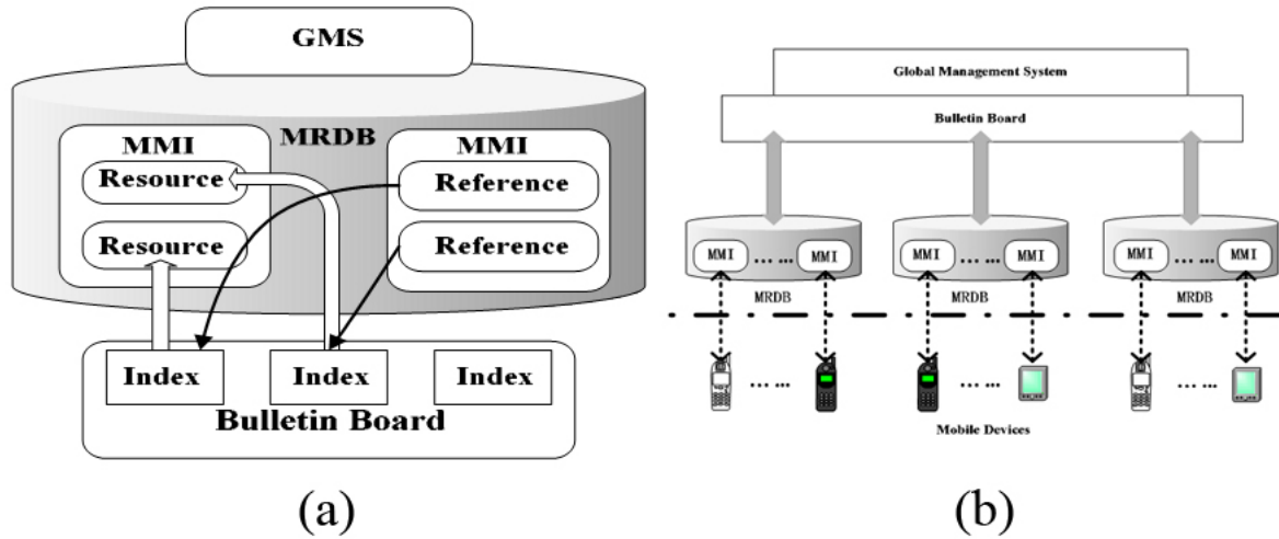
Figura 3.1: Arquitetura do MIRES
