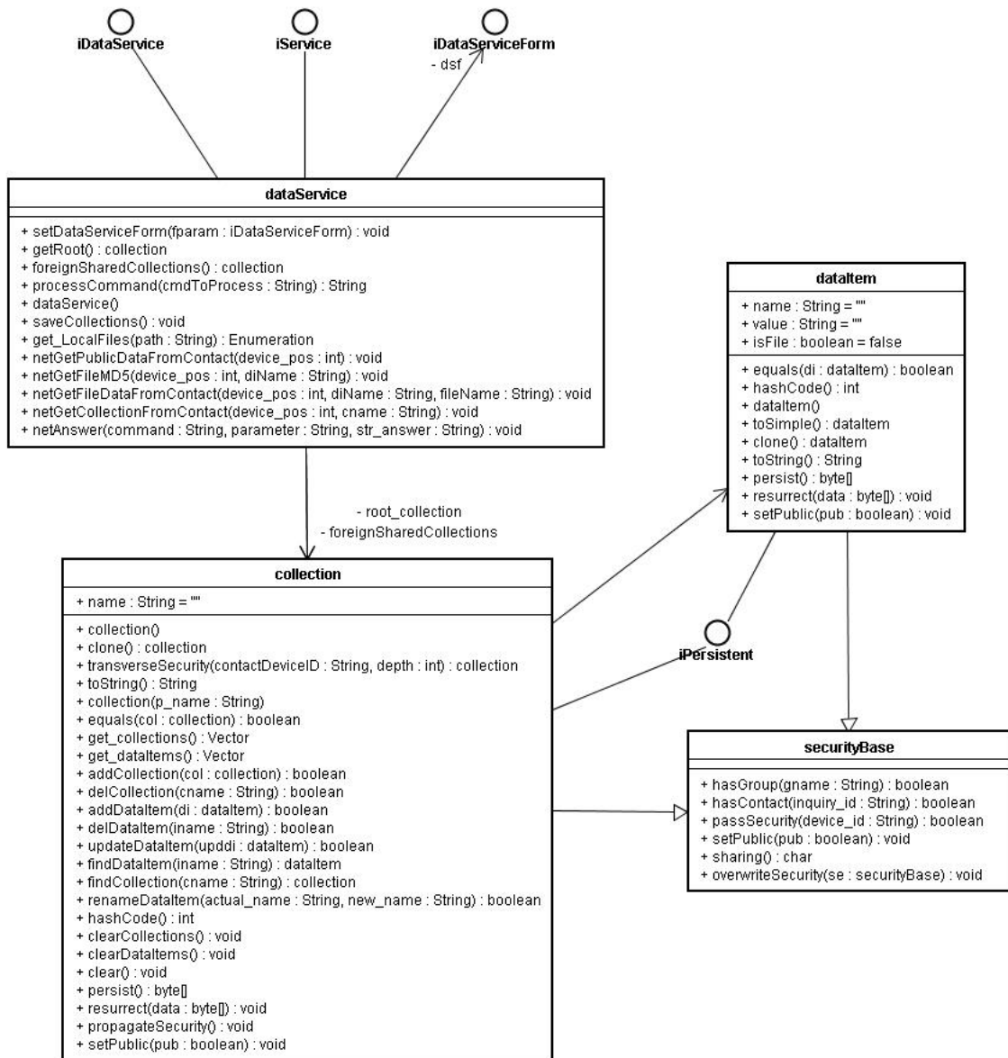
Figura 4.6: Componentes do Serviço de Dados
