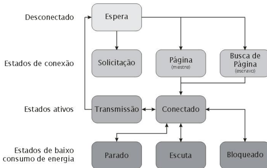
Figura 2.4: Diagrama de estados da especificação Bluetooth
