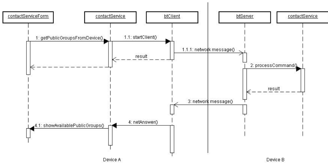
Figura 4.5: Exemplo de uma chamada callback
