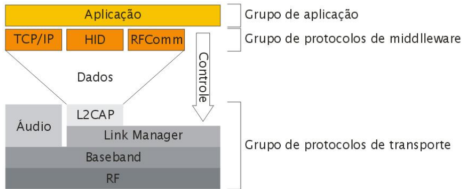
Figura 2.3: Pilha de protocolos Bluetooth
