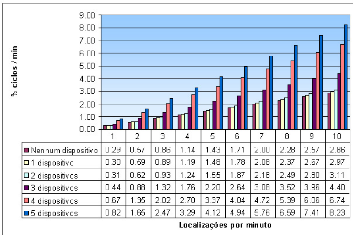
Figura 5.2: Ciclos de processamento na localização de dispositivos
