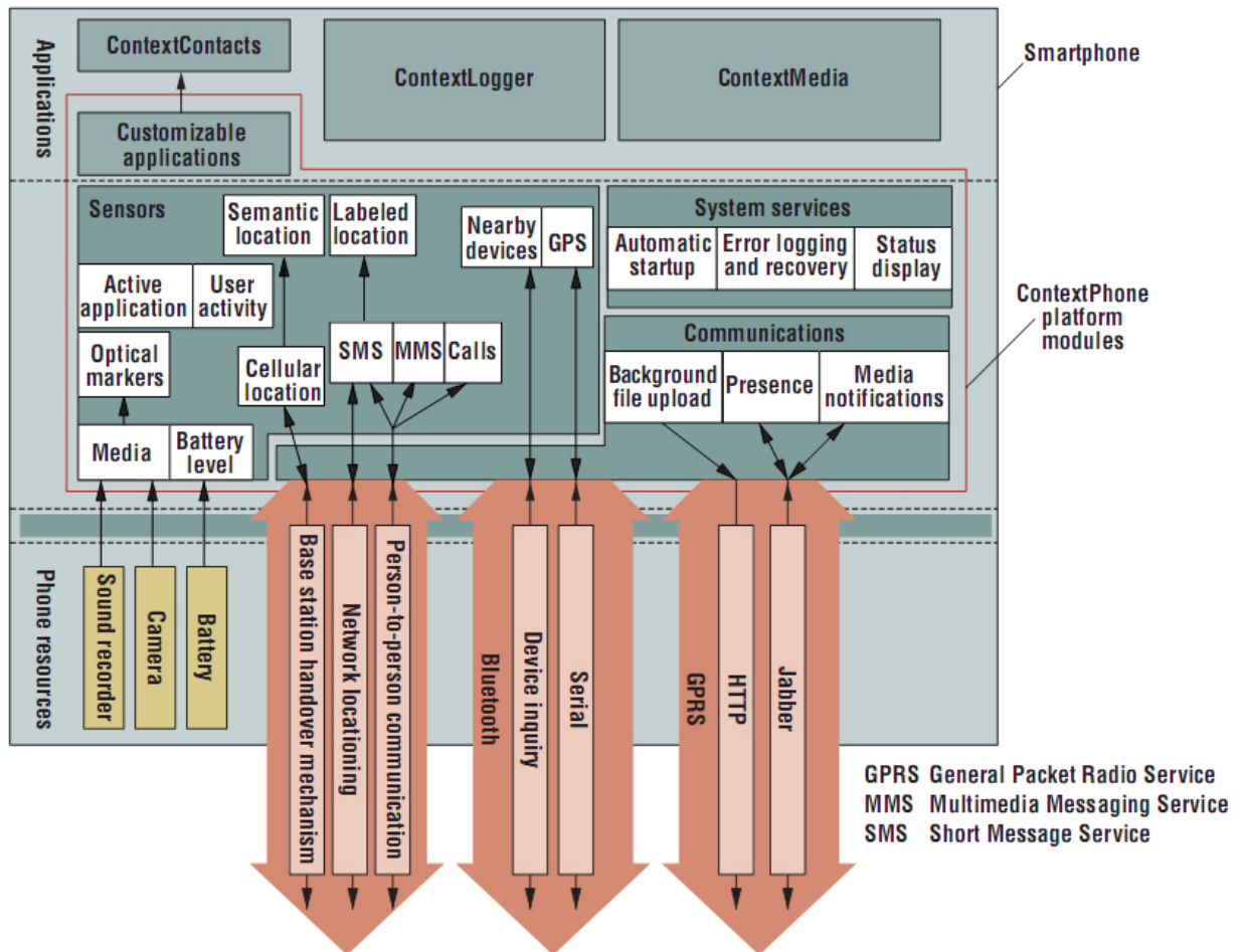
Figura 3.3: Arquitetura do ContextPhone
