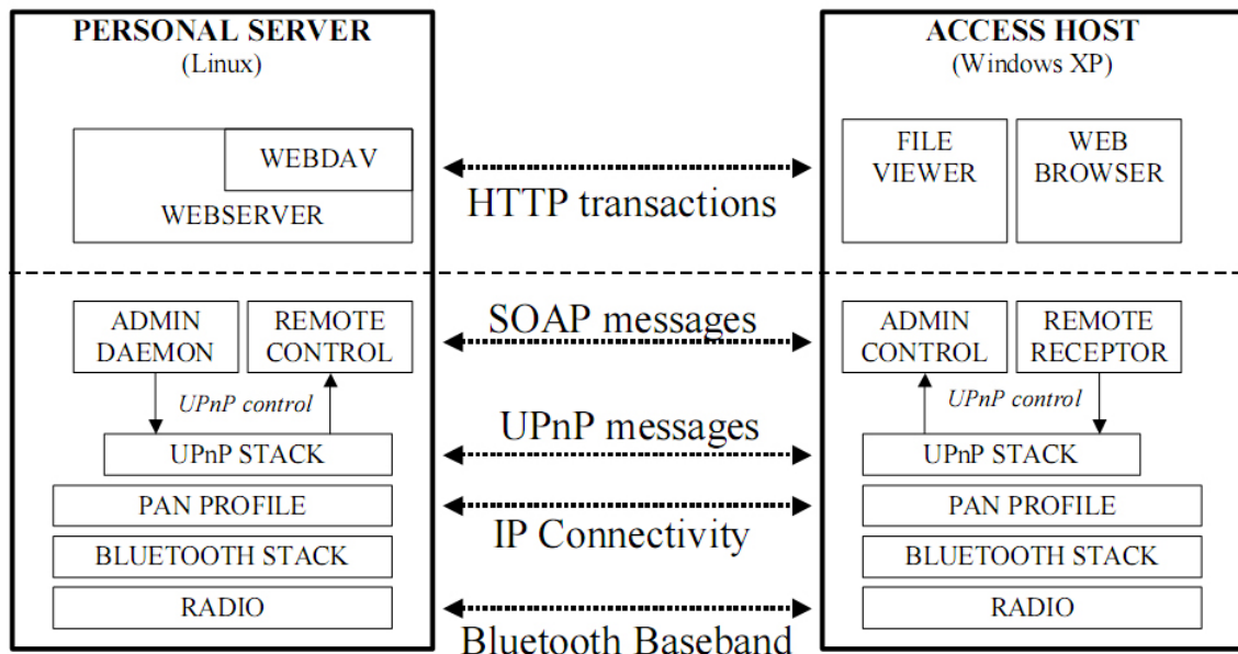
Figura 3.4: Arquitetura do PersonalServer
