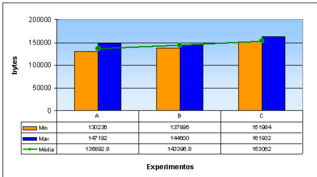
Figura 5.3: Média do consumo de memória na transferência de grupos
