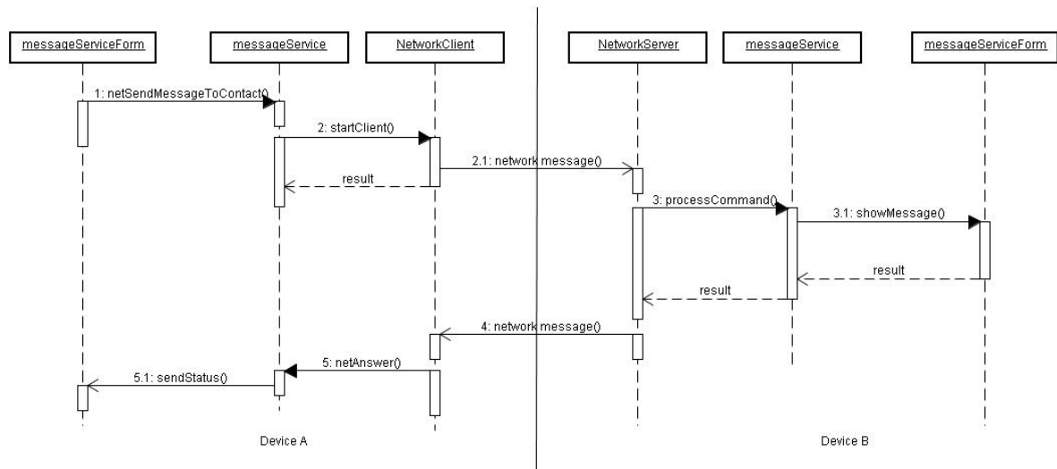
Figura 4.11: Diagrama de seqüência do envio de uma mensagem
