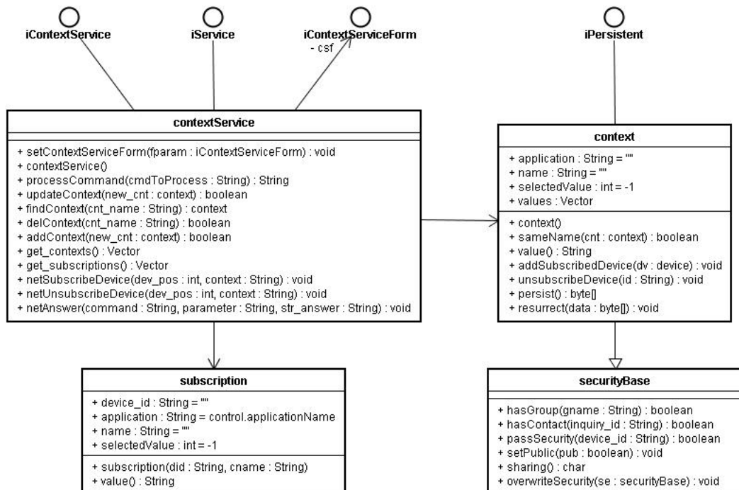
Figura 4.7: Componentes do Serviço de Contexto
