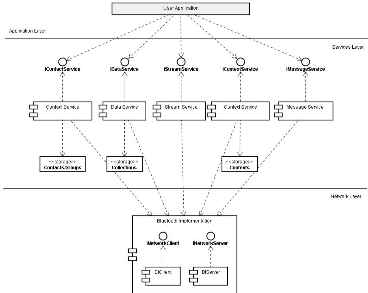
Figura 4.1: Diagrama dos componentes do SNU
