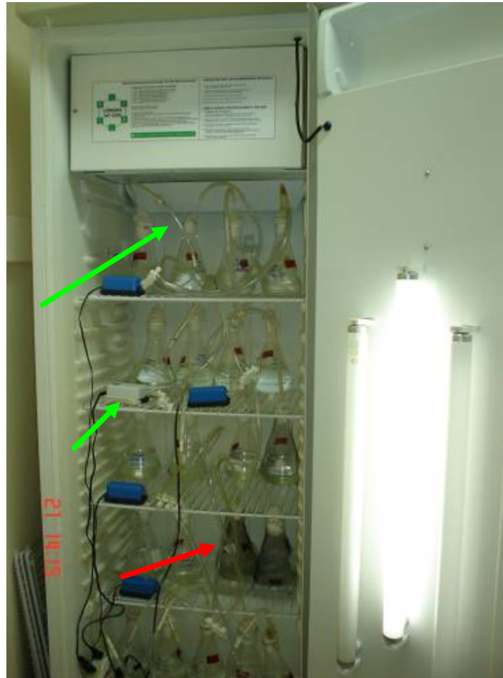
Figura 1: Incubadora com os erlenmeyers durante experimento de competição. Em detalhe erlenmeyers com os filtros pretos e sistema de aeração.
