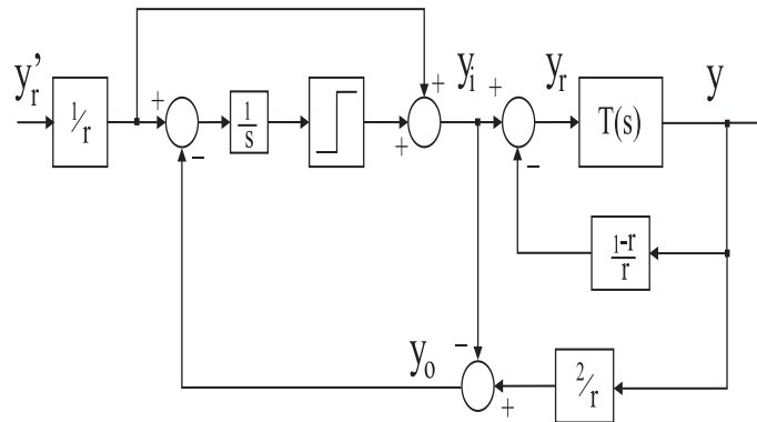
Figura 2.2: Estrutura do Experimento Ganho de Malha.
