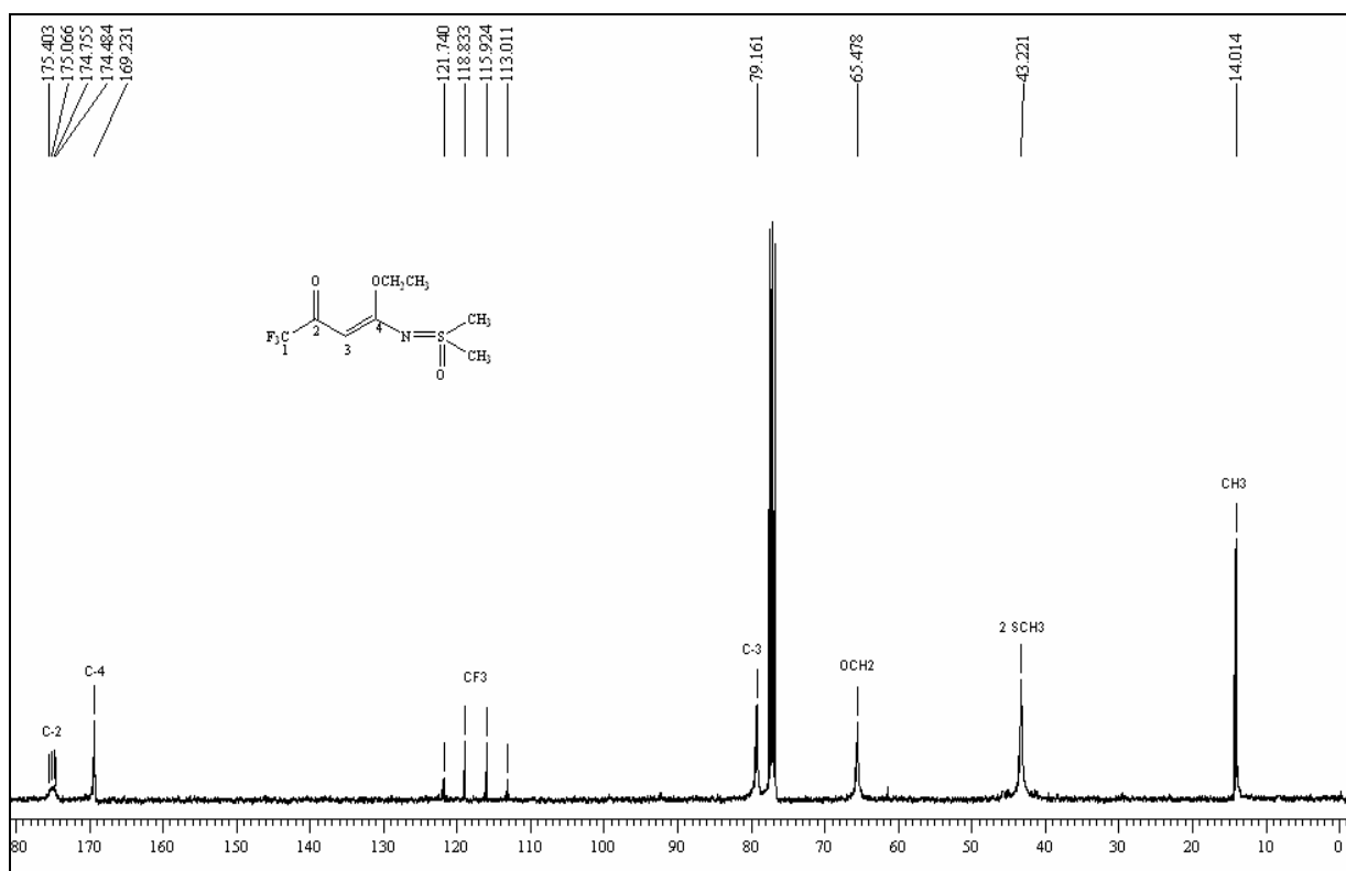
Figura 42 – Espectro de RMN ^1\text{H} a 200,13 MHz e RMN ^{13}\text{C} \{^1\text{H}\} a 100,61 MHz de 4-etóxi-4-dimetilsulfoximido-1,1,1-trifluor-3-buten-2-ona ( 51 ), em clorofórmio- d_1 .
