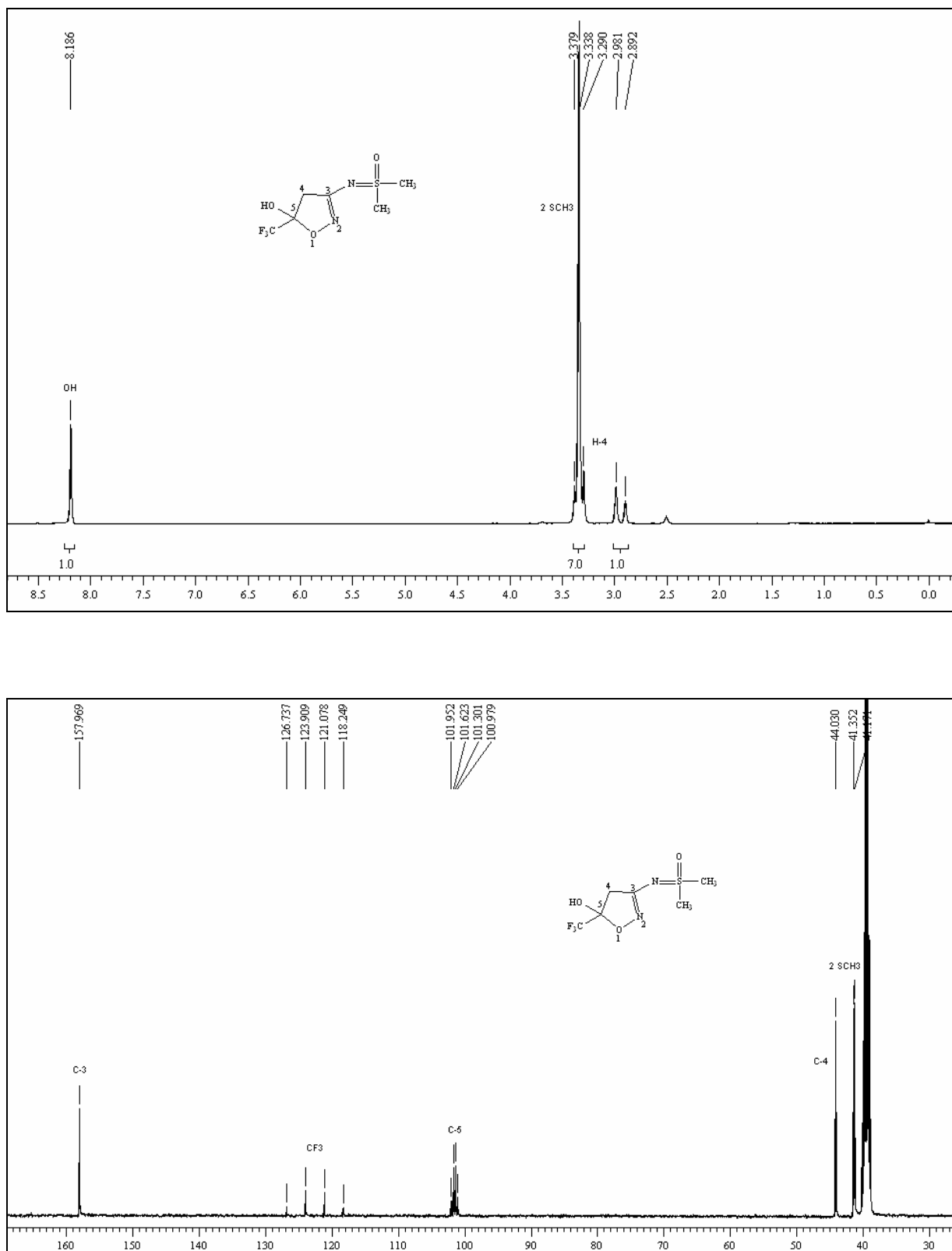
Figura 60 – Espectro de RMN ^1\text{H} a 200,13 MHz e RMN ^{13}\text{C} \{^1\text{H}\} a 100,61 MHz de 5-hidroxi-3-dimetilsulfoximido-5-trifluormetil-4,5-diidro-isoxazol ( 16 ), em \text{DMSO-}d_6 .
