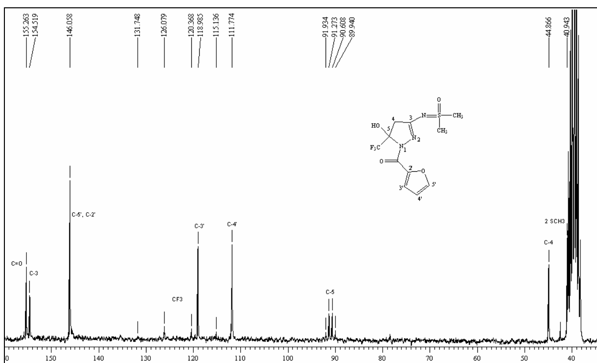
Figura 55 – Espectro de RMN 1 H a 200,13 MHz e RMN 13 C { 1 H} a 100,61 MHz de 5-hidroxi-3-dimetilsulfoximido-5-trifluormetil-4,5-diidro-1 H -1-(2-furanoil) pirazol ( 10 ), em DMSO- d 6 .
