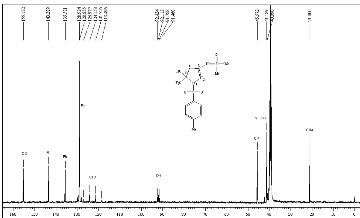
Figura 53 – Espectro de RMN ^1\text{H} a 200,13 MHz e RMN ^{13}\text{C} \{^1\text{H}\} a 100,61 MHz de 5-hidroxi-3-dimetilsulfoximido-5-trifluorometil-4,5-diidro-1H-1-tosilpirazol ( 8 ), em DMSO- d_6 .
