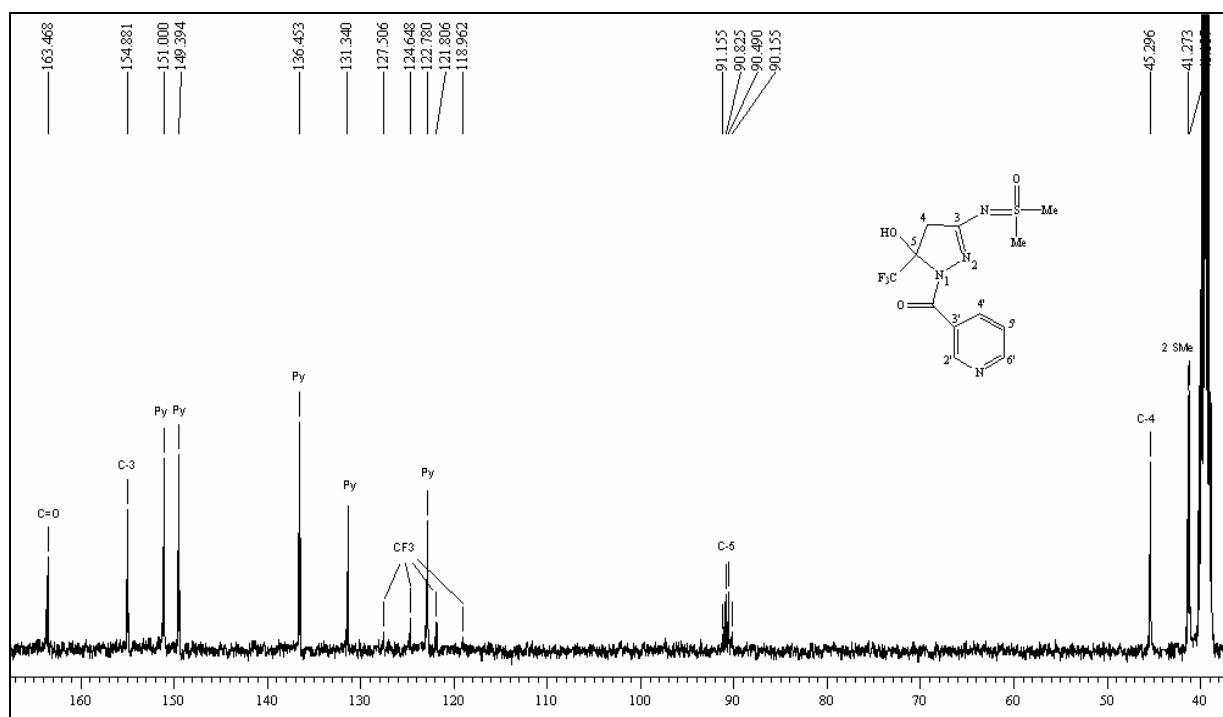
Figura 57 – Espectro de RMN 1 H a 200,13 MHz e RMN 13 C { 1 H} a 100,61 MHz de 5-hidroxi-3-dimetilsulfoximido-5-trifluorometil-4,5-diidro-1 H -1-nicotinoilpirazol ( 12 ), em DMSO- d 6 .
