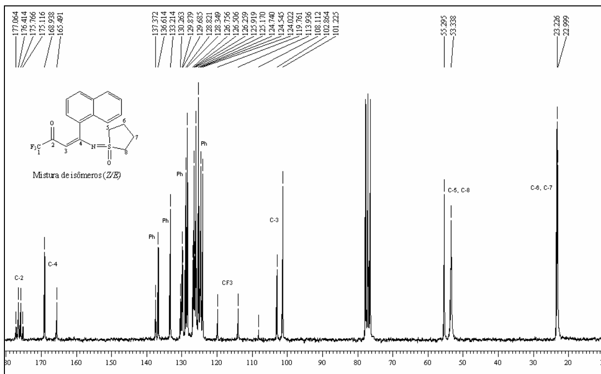
Figura 41 – Espectro de RMN ^1\text{H} a 200,13 MHz e RMN ^{13}\text{C} \{^1\text{H}\} a 100,61 MHz de 4-(1-naftil)-4-tetrametilenosulfoximido-1,1,1-trifluor-3-buten-2-ona ( 5k ), em clorofórmio- d_1 .
