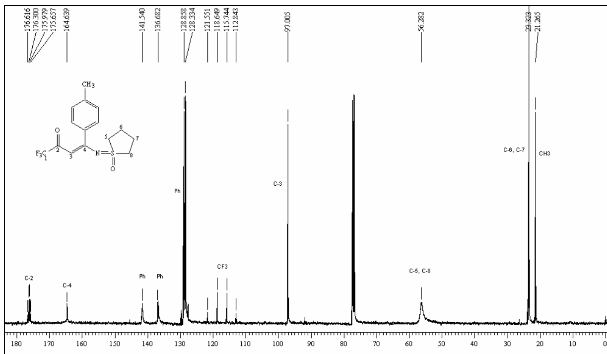
Figura 34 – Espectro de RMN ^1\text{H} a 200,13 MHz e RMN ^{13}\text{C} \{^1\text{H}\} a 100,61 MHz de 4-(4-metilfenil)-4-tetrametilenosulfoximido-1,1,1-trifluor-3-buten-2-ona ( 5d ), em clorofórmio- d_1 .
