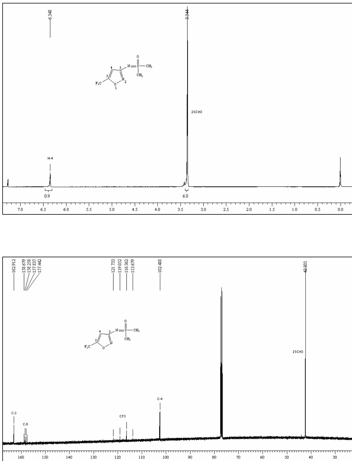
Figura 61 – Espectro de RMN 1 H a 200,13 MHz e RMN 13 C { 1 H} a 100,61 MHz de 3-dimetilsulfoximido-5-trifluormetil-isoxazol ( 17 ), em clorofórmio- d 1 .
