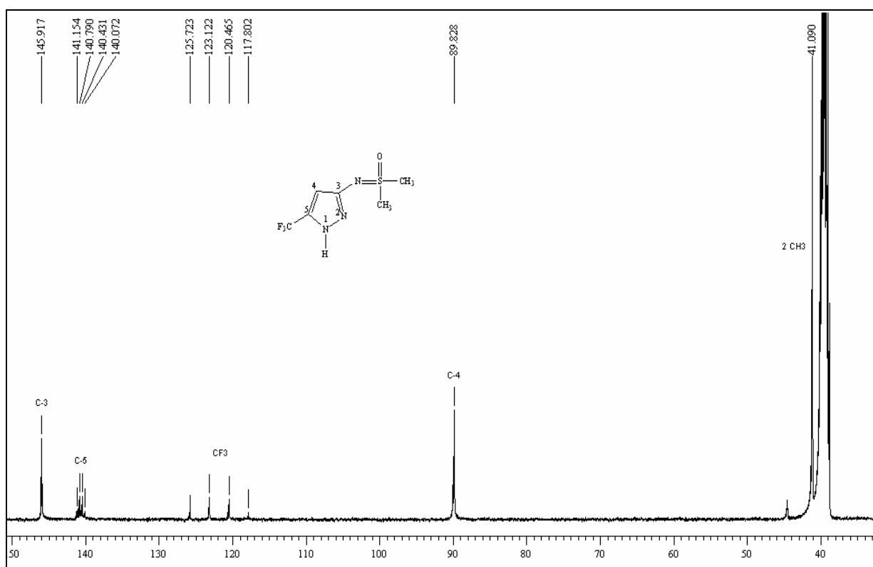
Figura 58 – Espectro de RMN ^1\text{H} a 200,13 MHz e RMN ^{13}\text{C} \{^1\text{H}\} a 100,61 MHz de 3-dimetilsulfoximido-5-trifluorometil-1H-pirazol ( 14 ), em \text{DMSO-}d_6 .
