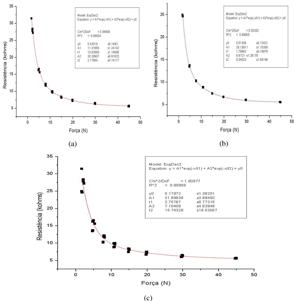
FIGURA. C.2. Curva de calibração: (a) ciclos ascendentes do sensor 3; (b) ciclos descendentes do sensor 3 e (c) todos os ciclos de calibração.
