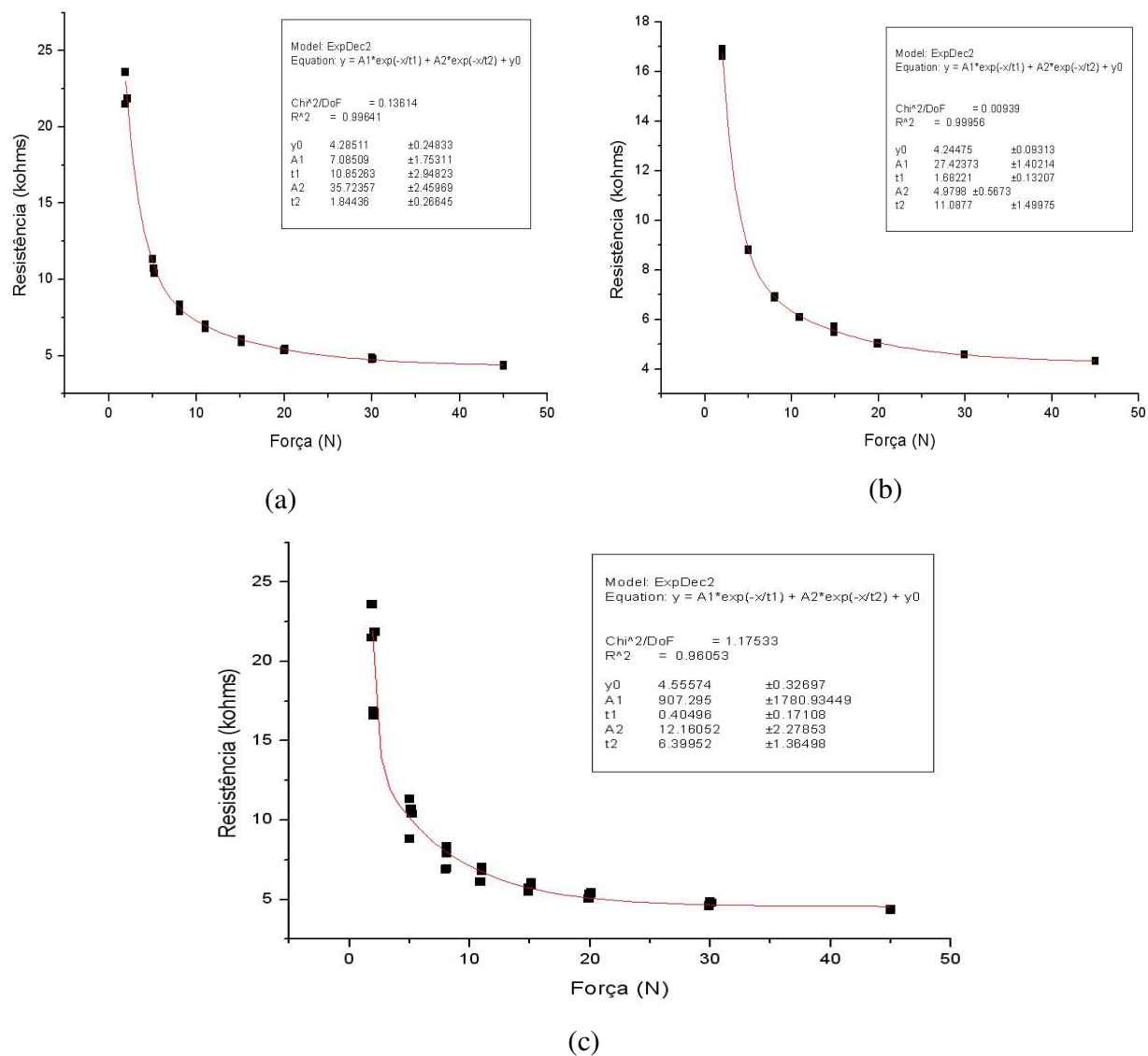
FIGURA. C.1. Curva de calibração: (a) ciclos ascendentes do sensor 2; (b) ciclos descendentes do sensor 2 e (c) todos os ciclos de calibração.
