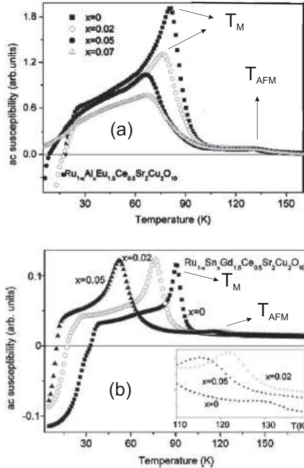
Figura 1.3: Componente real da susceptibilidade ac do composto (a) Ru_{1-x}Al_xSr_2Eu_{1.5}Ce_{0.5}Cu_2O_{10-\delta} . Componente real da susceptibilidade ac do composto (b) Ru_{1-x}Sn_xSr_2Eu_{1.5}Ce_{0.5}Cu_2O_{10-\delta} [10, 11]. As transições magnéticas estão indicadas em T_{AFM} (transição antiferromagnética da amostra, que em T_M era paramagnética) e T_{M2} (realce da magnetização do composto, que segundo a literatura pode ser da parte ferromagnética ou da parte antiferromagnética onde ocorreria uma espécie de “canting”). A transição supercondutora ocorre em T_{SC} . A T_M (transição ferromagnética de parte da amostra) não é mostrada, mas normalmente é observada através de Espectroscopia Mössbauer [10, 11].
