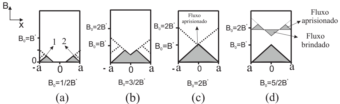
Figura 2.7: (a) Perfil de campo magnético aprisionado no estado reverso, com H_{ap} = 0 , no plano XZ da placa supercondutora da Fig. 2.1, segundo o modelo de Bean, para o caso de baixos campos máximos aplicados ( H_{ap} < H^* , onde H^* é o campo de penetração total da amostra, ou seja, penetração até o centro do plano XZ ). 1 e 2 indicam a linha do retorno que limita o fluxo aprisionado do lado esquerdo da placa ( x < 0 ) e a linha do retorno que limita o fluxo aprisionado do lado direito ( x > 0 ), respectivamente. (b) Perfil de campo magnético no estado reverso com H_{ap} = 0 após à aplicação de um campo máximo maior do que H^* . (c) Perfil de campo magnético no estado reverso com H_{ap} = 0 após à aplicação de um campo máximo igual a 2H^* . Repare que nesse caso o perfil de campo foi completamente revertido, sendo simétrico, com relação a reta H = H^* , ao perfil de campo para H_{ap} = 2H^* . Isso indica que a magnetização também foi toda revertida, mudando de sinal com relação a primeira etapa de penetração do campo (penetração virgem). (d) Esse último quadro ilustra o perfil de campo no estado reverso para H_{ap} = 0 após a amostra ter sido submetida à aplicação de um campo magnético máximo maior do que 2H^* . Repare que nesse caso, para qualquer H_{ap} > 2H^* , que o perfil de campo aprisionado é sempre igual ao perfil do caso (c), onde o campo magnético máximo aplicado foi H_{ap} = 2H^* . O quadro também ilustra os fluxos aprisionados e blindados durante a reversão do campo aplicado. Em todos os casos o campo magnético H_{ap} foi aplicado com a amostra no estado virgem, ou seja, sem histórico magnético.
