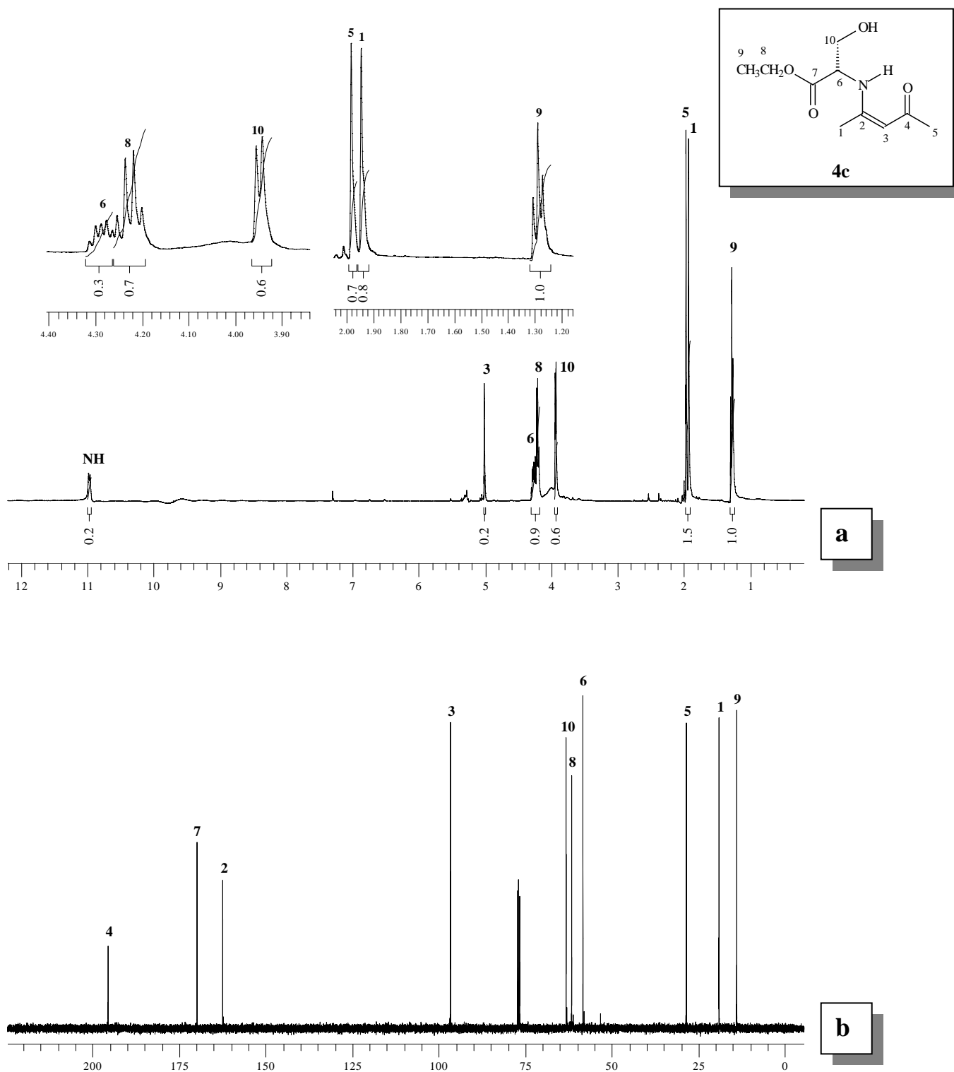
Figura 42 - Espectro de RMN de ^1\text{H} (a) a 400 MHz e ^{13}\text{C} (b) a 100 MHz em \text{CDCl}_3 do ( S,Z )-3-hidroxi-2-(4-oxo-2-pentenilamino)-propanoato de etila ( 4c ).
