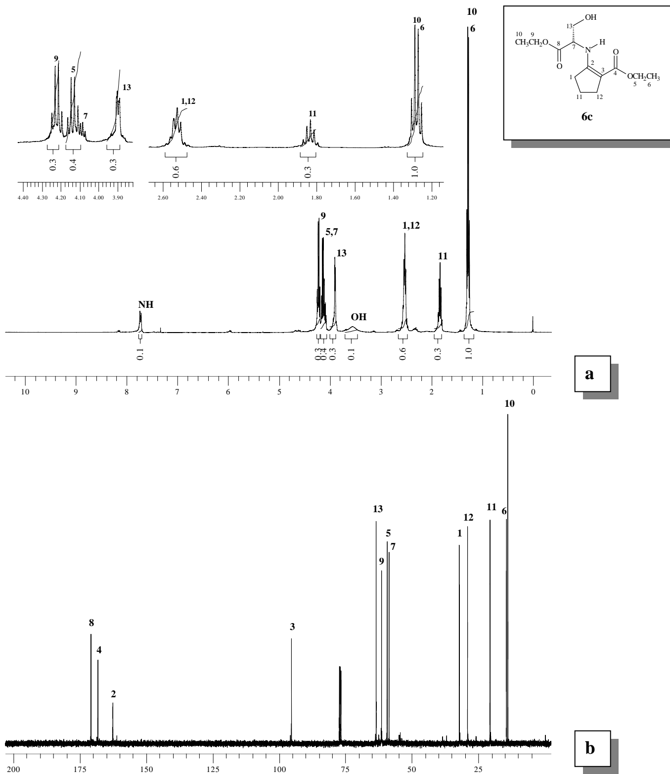
Figura 55 - Espectro de RMN de ^1\text{H} (a) a 400 MHz e ^{13}\text{C} (b) a 100 MHz em \text{CDCl}_3 do ( S )-2-(1-etóxi-3-hidróxi-1-oxo-2-propanilamina) -1-ciclopentenecarboxilato de etila ( 6c ).
