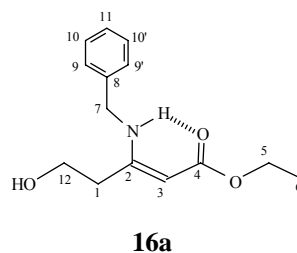
Figura 24: Estrutura proposta para o composto 16 .
