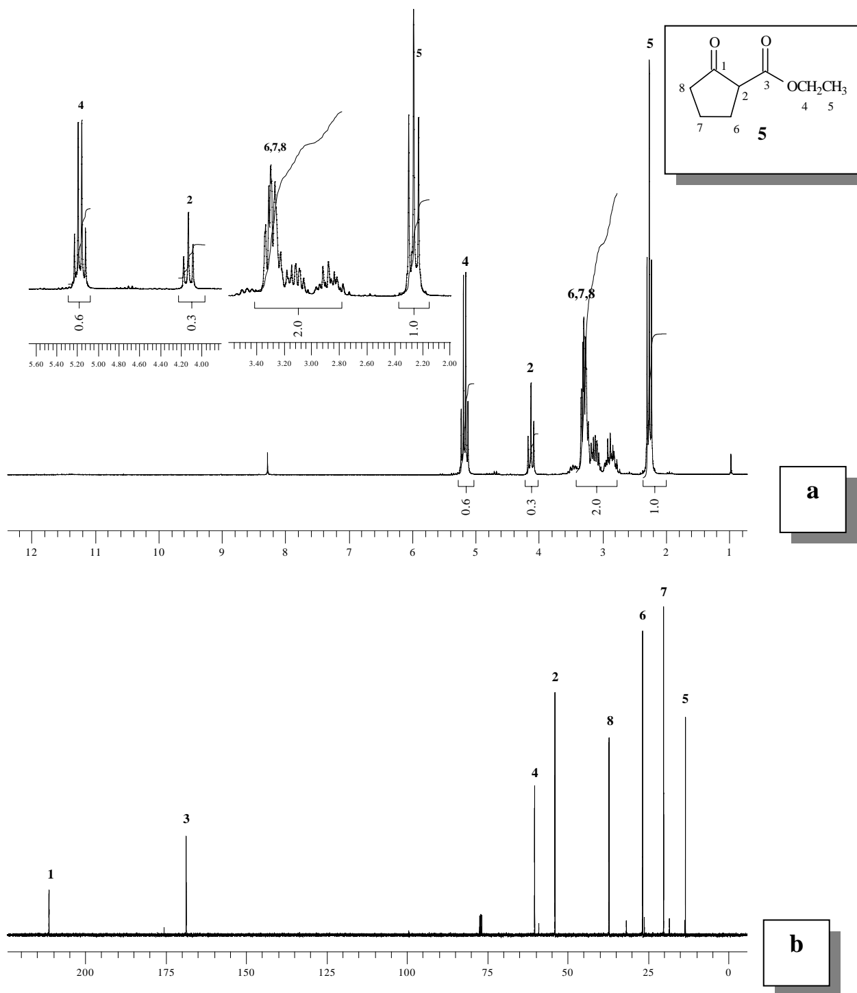
Figura 51- Espectro de RMN de 1 H (a) a 200 MHz e 13 C (b) a 100 MHz em CDCl 3 do 2- oxo-1-ciclopentanocarboxilato de etila (5).
