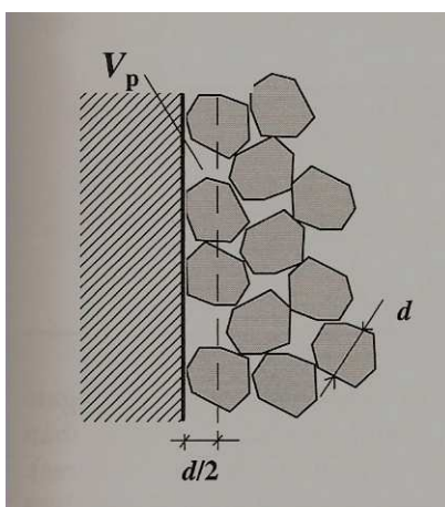
Figura 26: modelo de Bem-Aïm, demonstrando o volume perturbado de container (Fonte: De Larrard, 1999)
