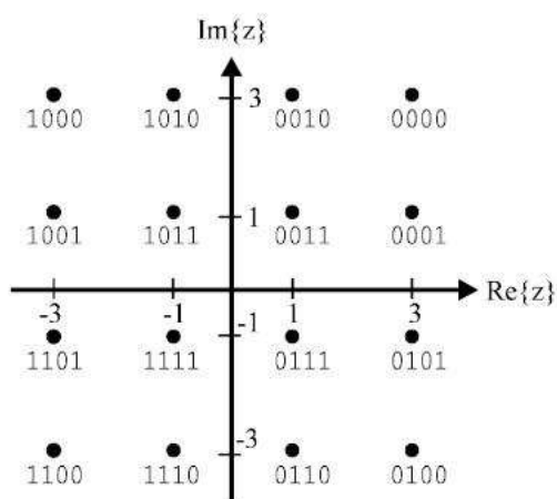
Figura 2.13 – Constelação 16QAM [5]
