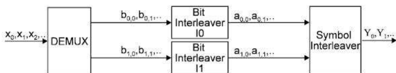
Figura 2.9 – Entrelaçador Interno para modulação QPSK [5]
