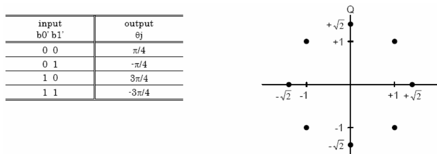
Figura 2.22 – Mapeamento para uma modulação DQPSK
