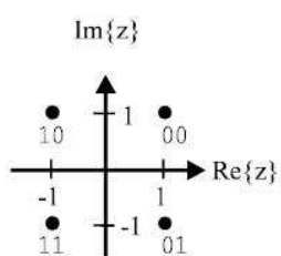
Figura 2.12 – Constelação QPSK [5]
