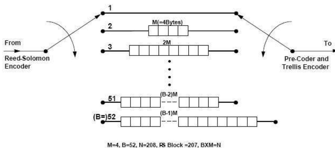
Figura 2.2 – Entrelaçador de dados [4]
