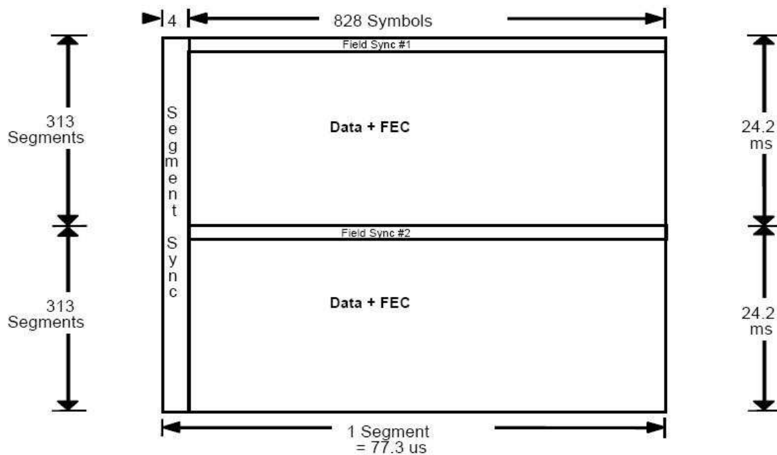
Figura 2.4 – Estrutura do Frame
