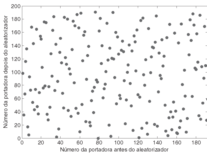
Figura 2.32 – Gráfico de dispersão das portadoras dentro de um segmento no modo 4K
