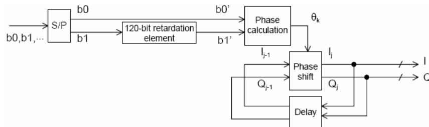
Figura 2.21 – Interleaver de Bit para modulação DQPSK
