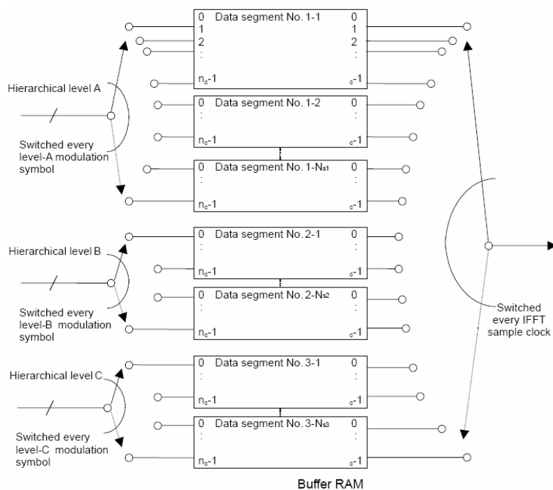
Figura 2.29 – Combinador de Níveis Hierárquicos
