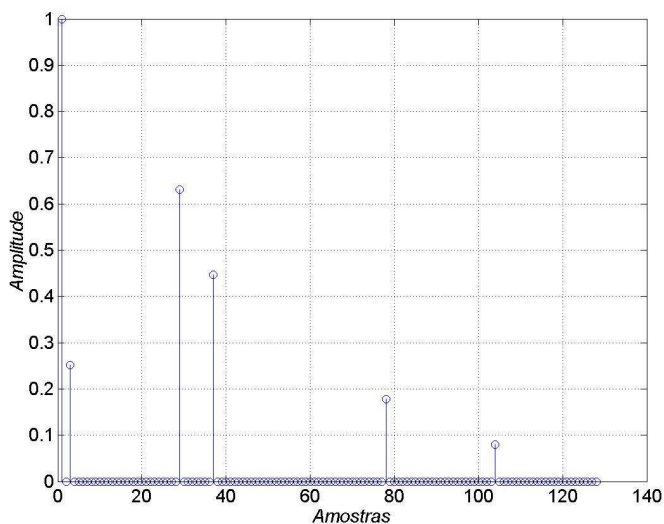
Figura 4.2 – Magnitude da resposta ao impulso do canal Brazil B no domínio do tempo.
