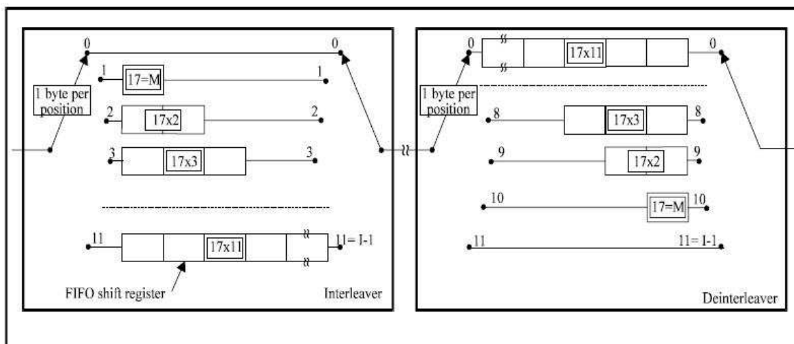
Figura 2.8 – Figura do Interleaver e Deinterleaver [5]
