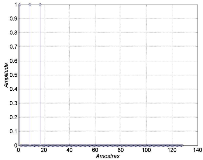
Figura 4.5 – Magnitude da resposta ao impulso do canal Brazil E no domínio do tempo.
