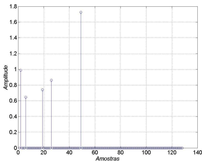
Figura 4.4 – Magnitude da resposta ao impulso do canal Brazil D no domínio do tempo.
