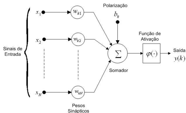
Figura 3.1 – Modelo de um neurônio não-linear [7]
