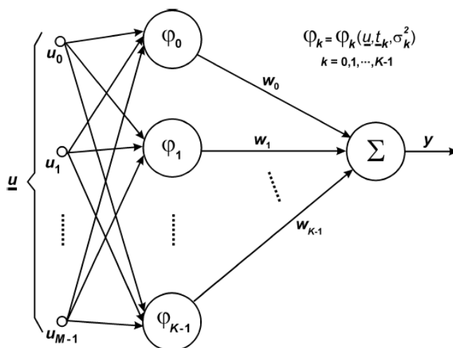
Figura 3.2 – Arquitetura de uma rede RBF [7]
