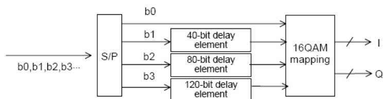
Figura 2.25 – Interleaver de Bit para modulação 16QAM
