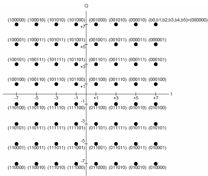
Figura 2.28 – Mapeamento para uma modulação 64QAM
