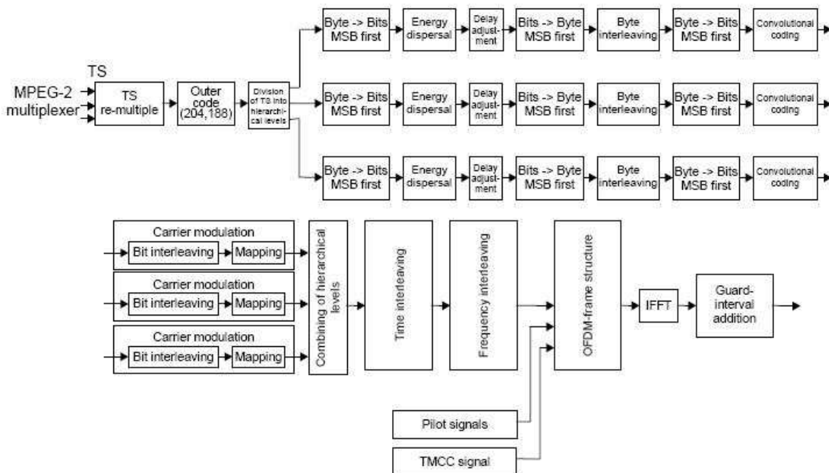
Figura 2.17 – Diagramas de bloco do sistema ISDB [6]
