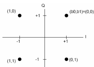
Figura 2.24 – Mapeamento para uma modulação QPSK
