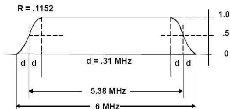
Figura 2.6 – Resposta do Filtro de Nyquist
