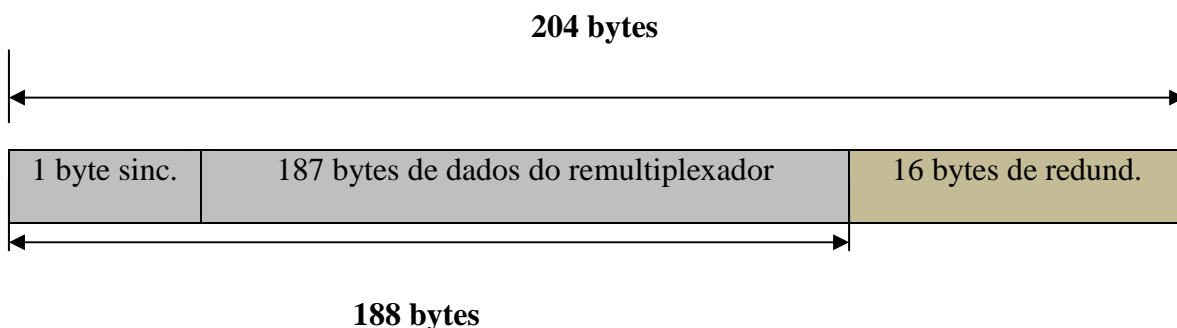
Figura 2.20 – Pacotes de saída do codificador Reed Solomon
