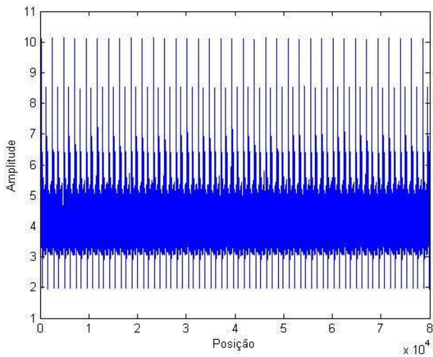
Figura 5.13 – Saída da RNA para o canal Brazil B identificando todos IGs.
