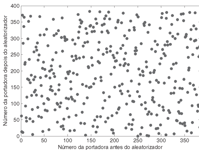
Figura 2.33 – Gráfico de dispersão das portadoras dentro de um segmento no modo 8K
