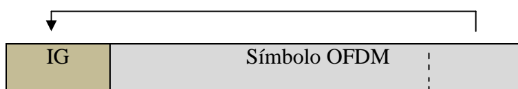
Figura 2.15 – Figura do Símbolo OFDM com o Intervalo de Guarda
