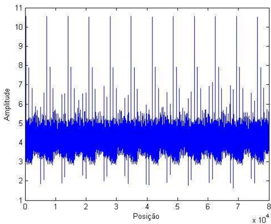
Figura 5.5 – Saída da RNA para o canal Brazil A
