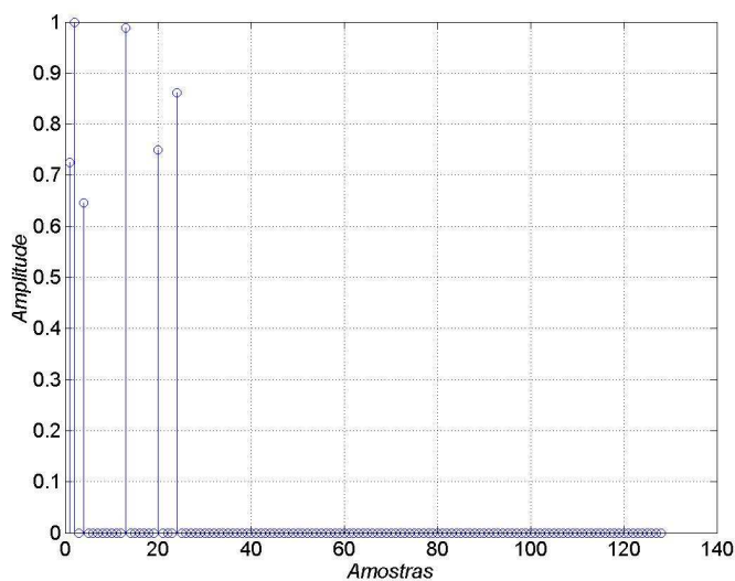
Figura 4.3 – Magnitude da resposta ao impulso do canal Brazil C no domínio do tempo.
