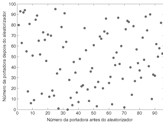
Figura 2.31 – Gráfico de dispersão das portadoras dentro de um segmento no modo 2K
