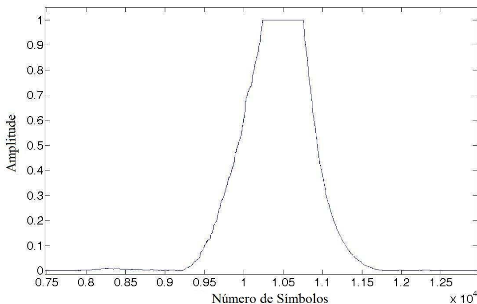
Figura 5.2 – Platô do Intervalo de Guarda do Símbolo de tamanho 1/4
