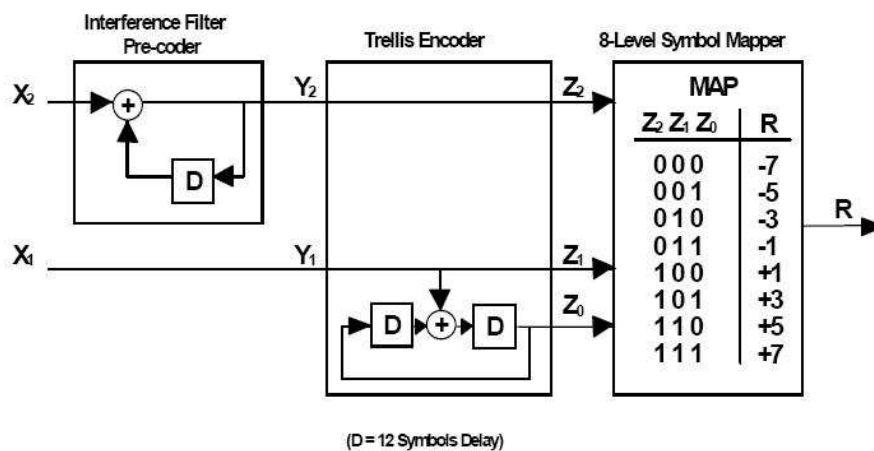
Figura 2.5 – Filtro de Interferência, Codificador de Treliça e Mapeador de símbolos 8VSB
