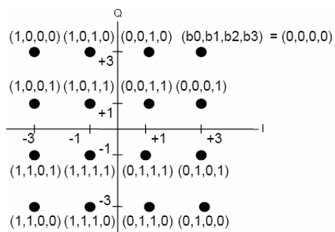
Figura 2.26 – Mapeamento para uma modulação 16QAM
