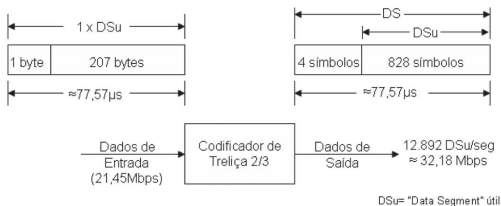
Figura 2.3 – Entrada e Saída dos dados do bloco Codificador de Treliça [4]
