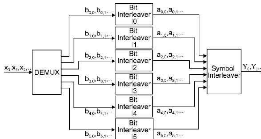
Figura 2.11 – Entrelaçador Interno para modulação 64QAM [5]
