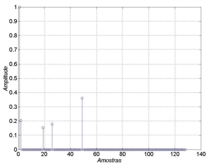
Figura 4.1 – Magnitude da resposta ao impulso do canal Brazil A no domínio do tempo.
