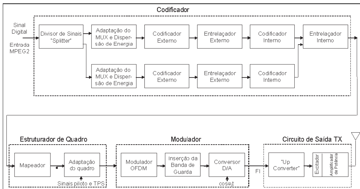
Figura 2.7 – Diagrama em Blocos do Sistema DVB [5]
