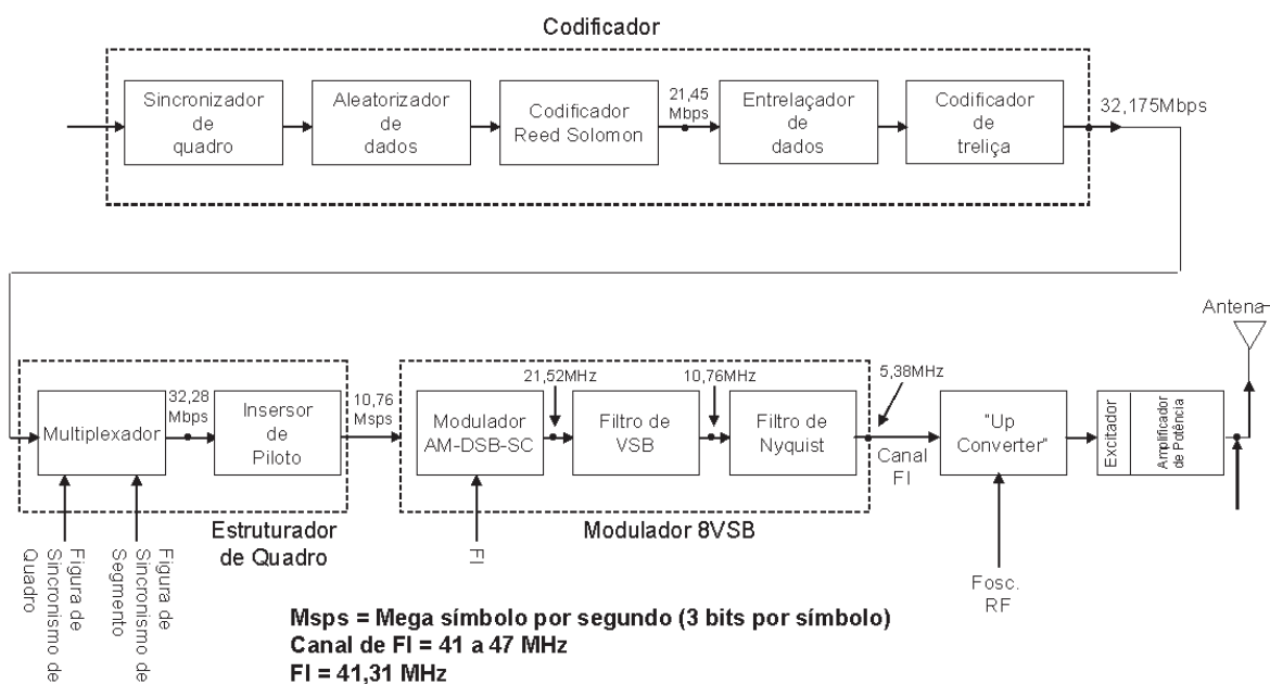
Figura 2.1 – Diagrama de Blocos do sistema ATSC [4]
