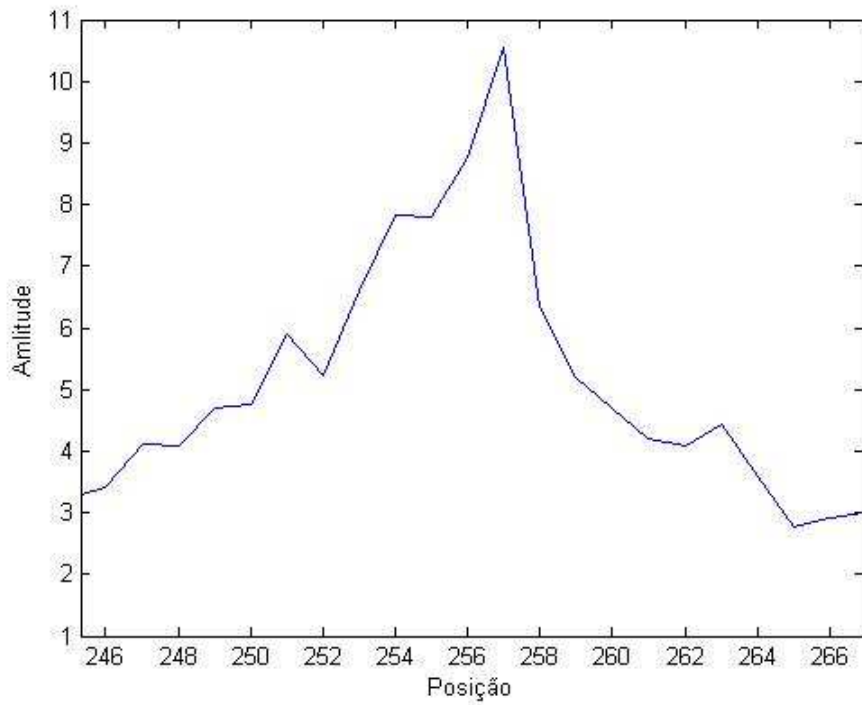
Figura 5.17 – Posição Inicial do Primeiro Símbolo OFDM do Canal Brazil A
