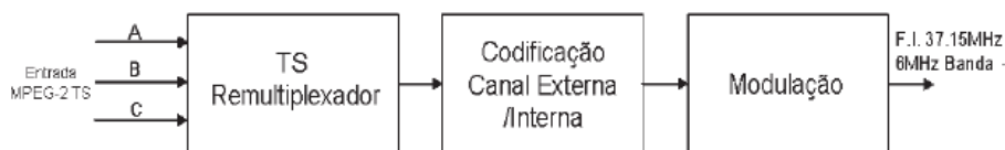
Figura 2.18 – Sistema ISDB dividido em três blocos
