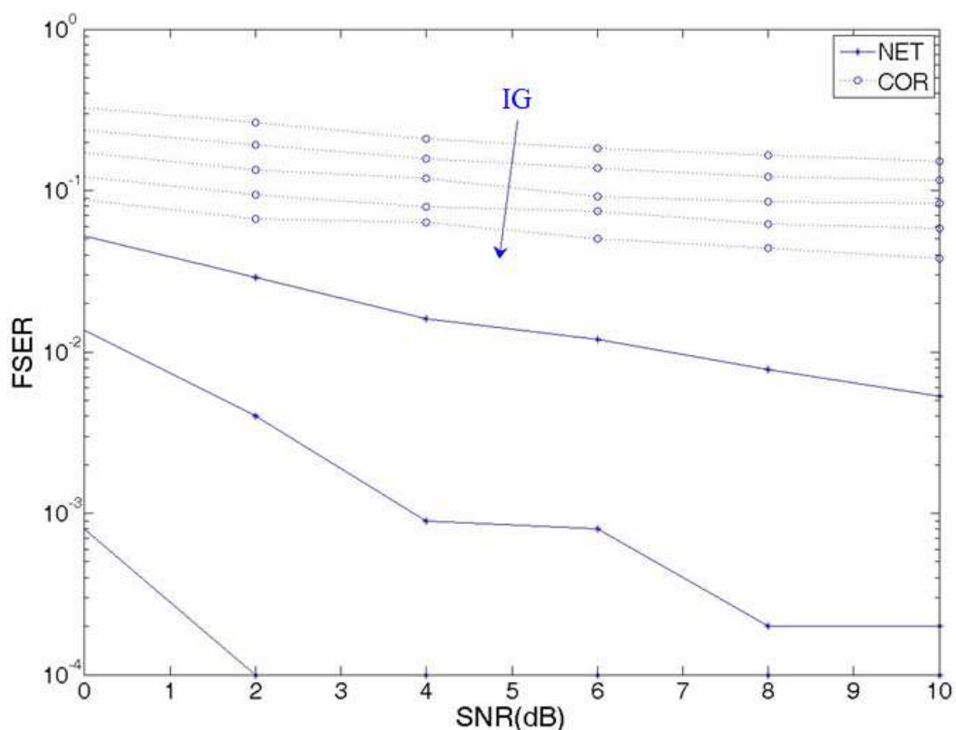
Figura 5.3 – Curva de FSER da identificação por RNA e por Correlação para IGs e SNR diferentes
