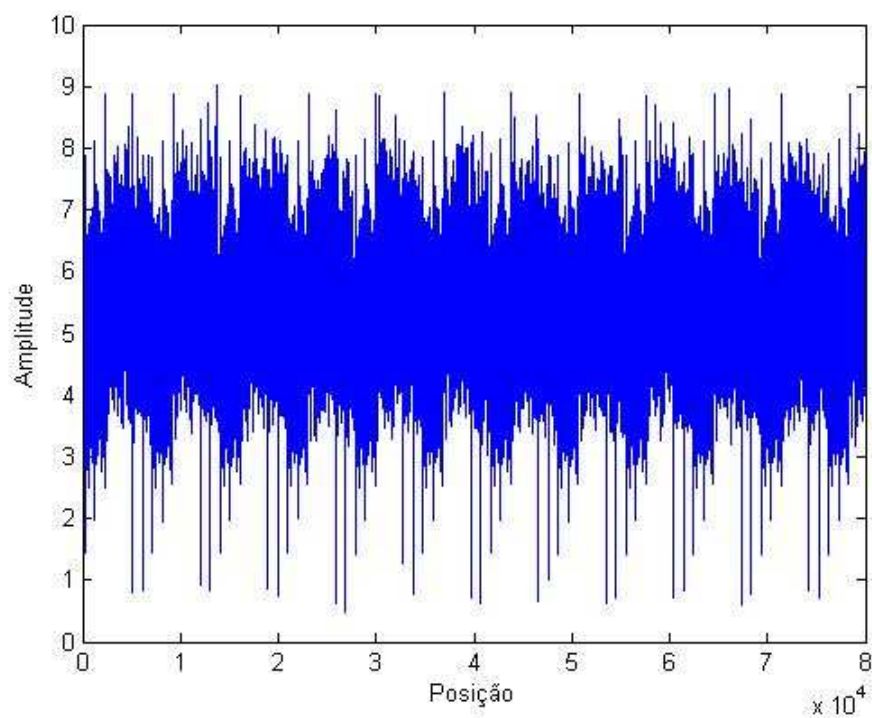
Figura 5.7 – Saída da RNA para o canal Brazil C
