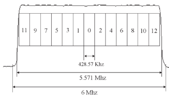
Figura 2.16 – Figura da segmentação do canal de 6MHz
