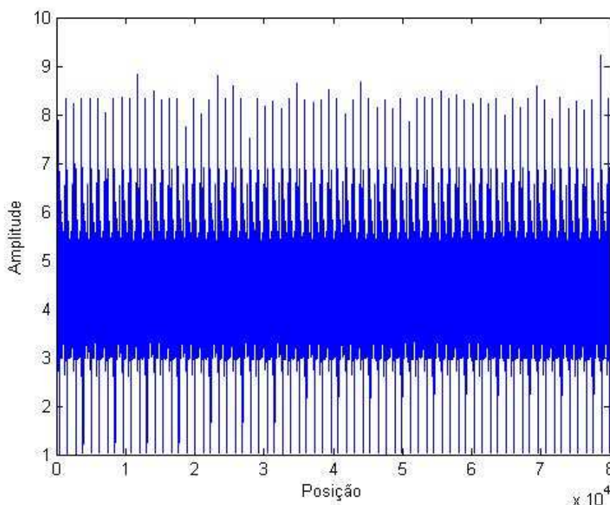
Figura 5.16 – Saída da RNA para o canal Brazil E identificando todos IGs.
