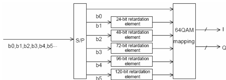
Figura 2.27 – Interleaver de Bit para modulação 64QAM
