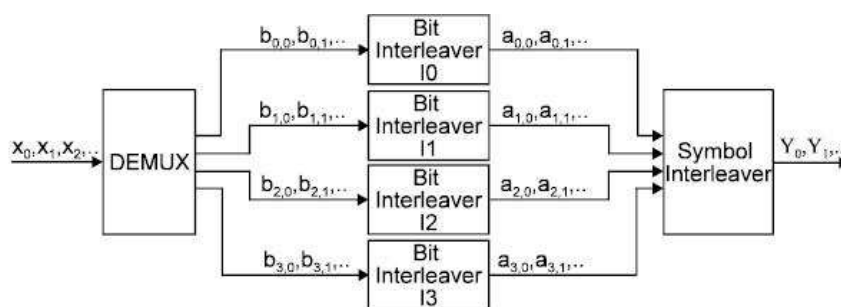
Figura 2.10 – Entrelaçador Interno para modulação 16QAM [5]
