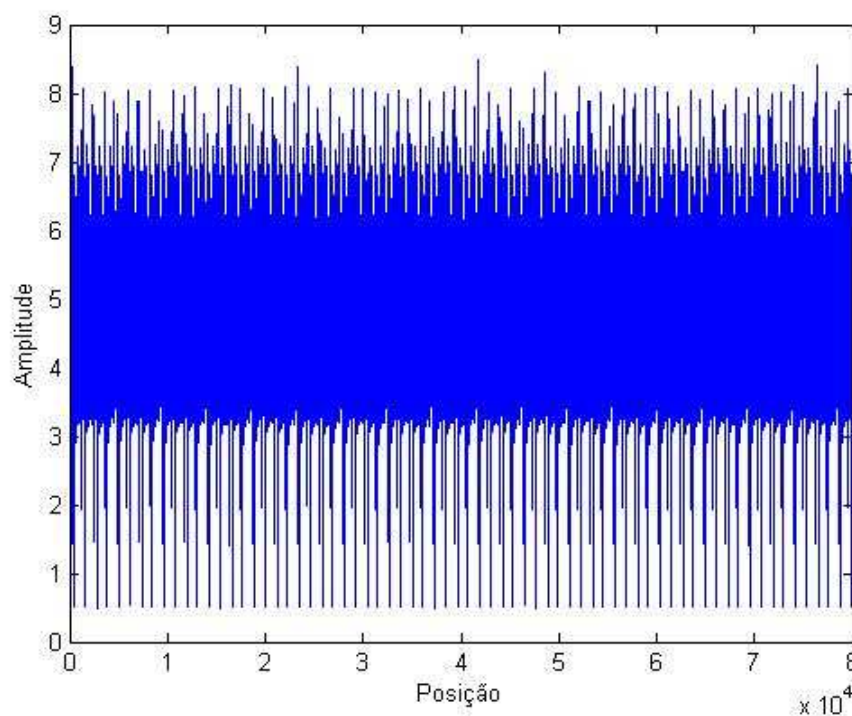
Figura 5.14 – Saída da RNA para o canal Brazil C identificando todos IGs.
