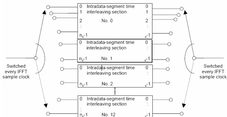
Figura 2.30 – Interleaver de Tempo
