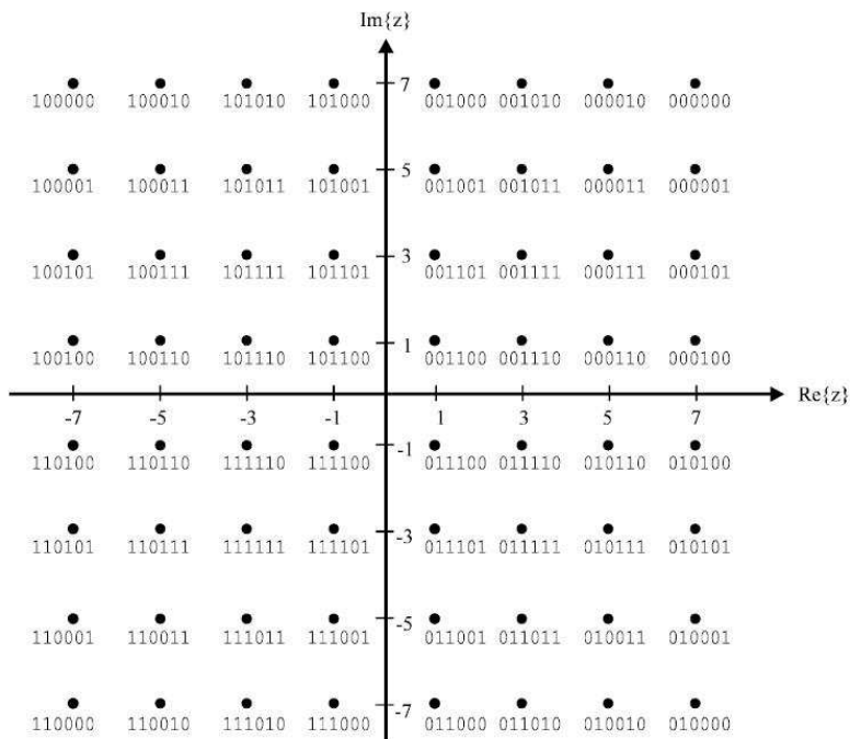
Figura 2.14 – Constelação 64QAM [5]
