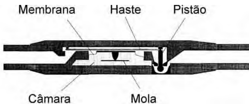
Fig. 2.7 – Válvula Beverly Reverential Valve, ilustrada por Drake & Sainte-Rose (1994).
