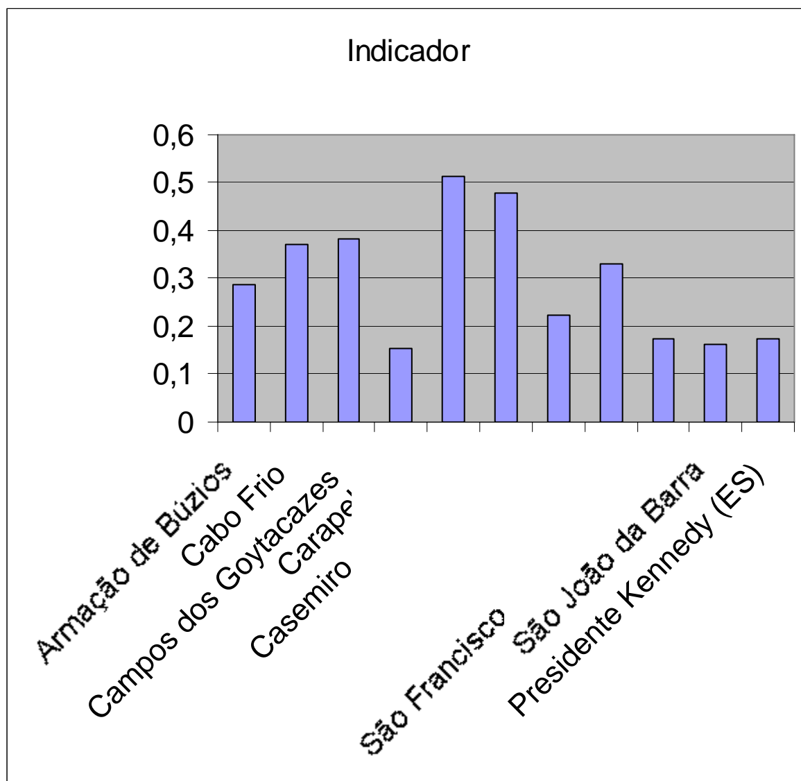
Figura 1 – Qualidade de Vida – IQM nos Municípios que compõe a OMPETRO – 2000
