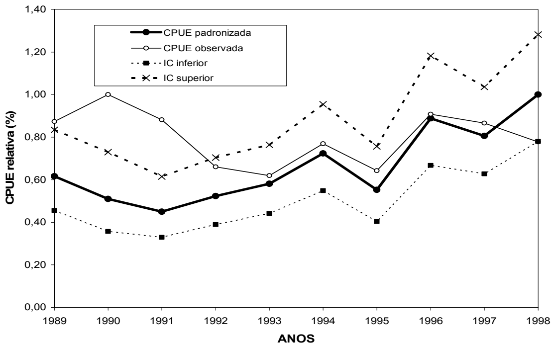
Figura 50 – CPUE padronizada estimada pelo modelo delta-Gamma, com respectivos intervalos de confiança e CPUE nominal, do bonito listrado, para o período 1989-1998. Valores escalonados em relação ao valor máximo de cada série de CPUE.
