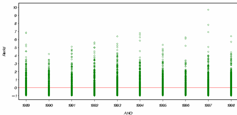
Figura 48 – Gráfico dos resíduos por ano. Modelo linear generalizado misto, com distribuição Gamma, aplicado aos dados de CPUE das capturas positivas do bonito listrado das pescarias com isca-viva, no sudeste e sul do Brasil, no período de 1989 a 1998.
