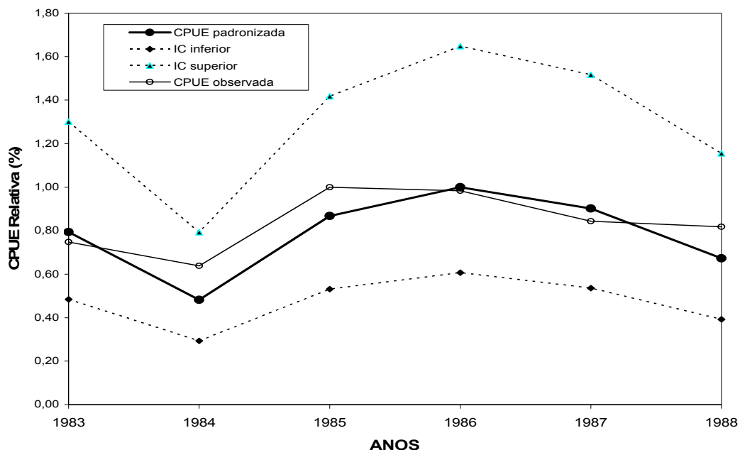
Figura 65 – CPUE padronizada estimada pelo modelo delta-Gamma, com respectivos intervalos de confiança e CPUE nominal do bonito listrado, para o período 1983-1988. Valores escalonados em relação ao valor máximo de cada série de CPUE.
