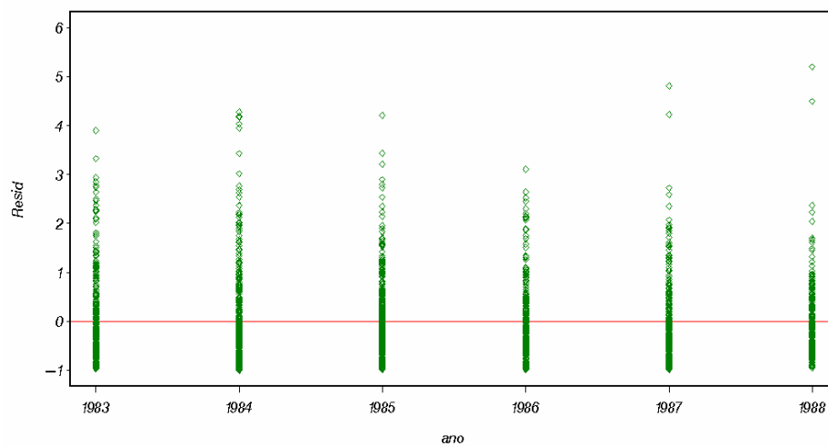
Figura 63 – Dispersão dos resíduos por ano. Modelo linear generalizado misto, com distribuição Gamma, ajustado aos dados de CPUE das capturas positivas do bonito listrado, das pescarias com vara e isca-viva, no sudeste e sul do Brasil, no período de 1983 a 1988.
