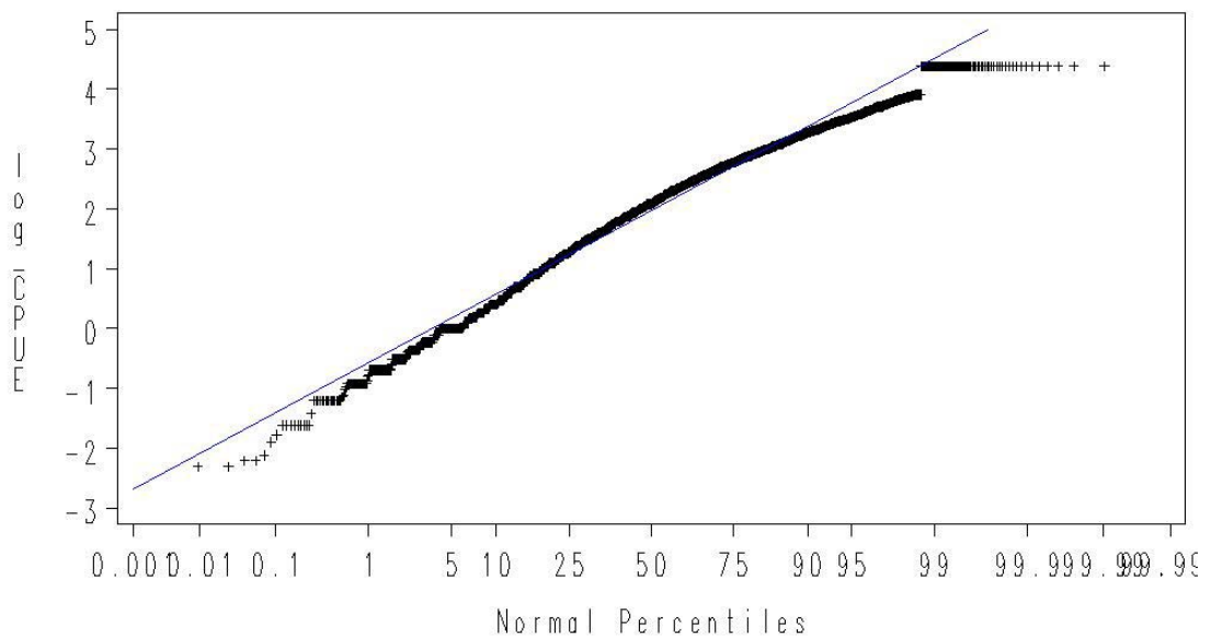
Figura 33 – Gráfico normal de probabilidade do logaritmo da CPUE positiva do bonito listrado, das pescarias dos barcos arrendados nacionalizados, no período 1983-1998, em função dos percentis da distribuição normal padrão.
