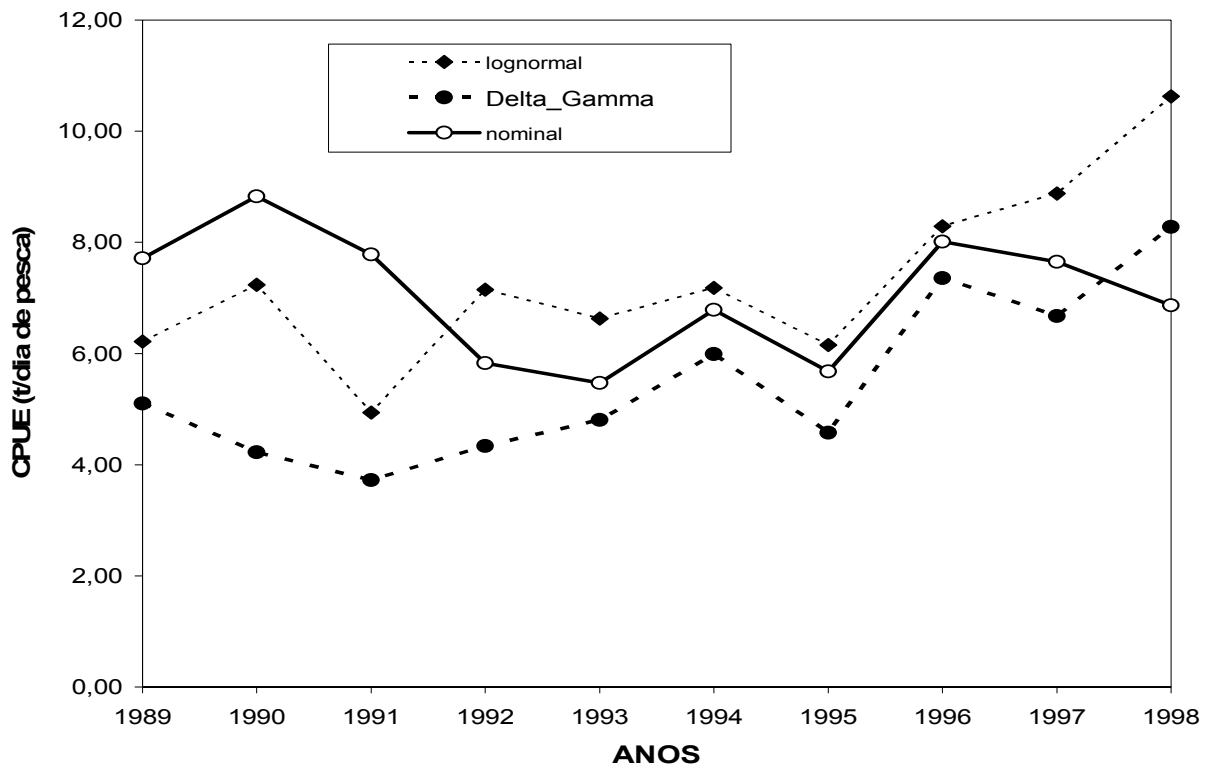
Figura 51 – Comparação entre a CPUE nominal e as duas séries de CPUE do bonito listrado, padronizadas pelos modelos delta-lognormal e delta-Gamma, da pescaria com isca-viva, do sudeste e sul do Brasil, no período 1989-1998.
